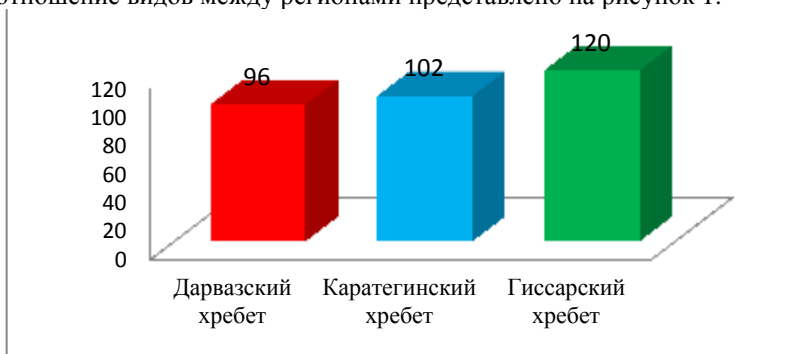
Рисунок 1. - Соотношение видов.
