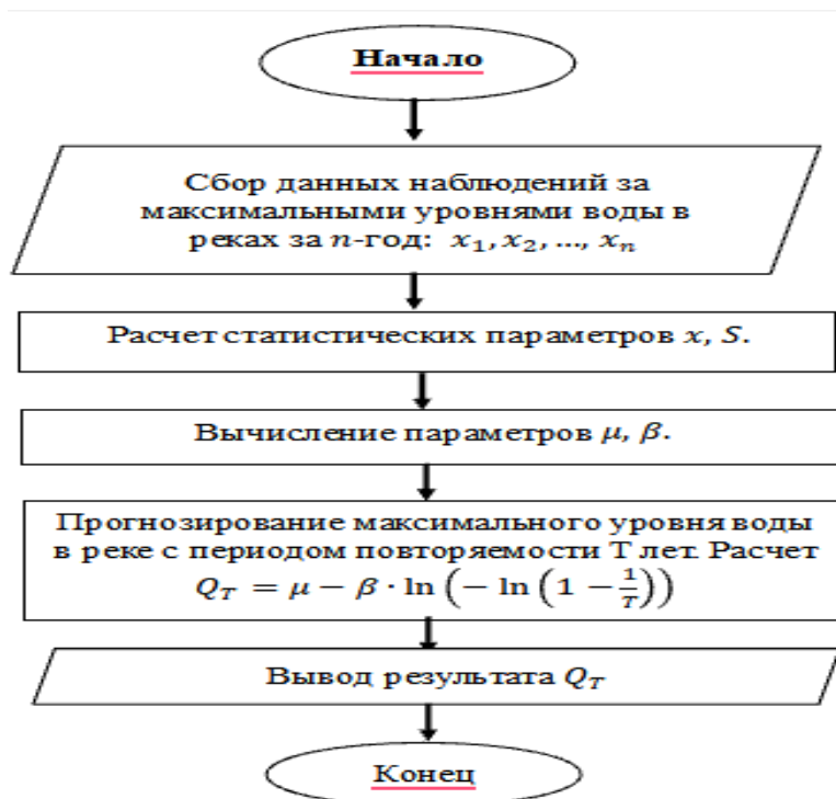
Рисунок 3.1.2. - Блок-схема алгоритма прогнозирования экстремальных уровней воды в реке с использованием модели Гумбеля
