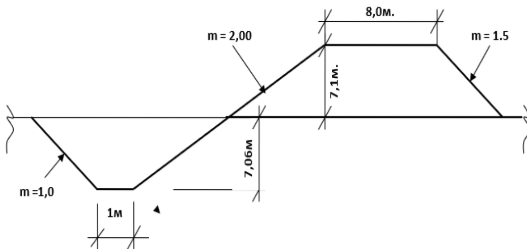
Расми 3.1.2. - Параметрҳои лоиҳавии садд
