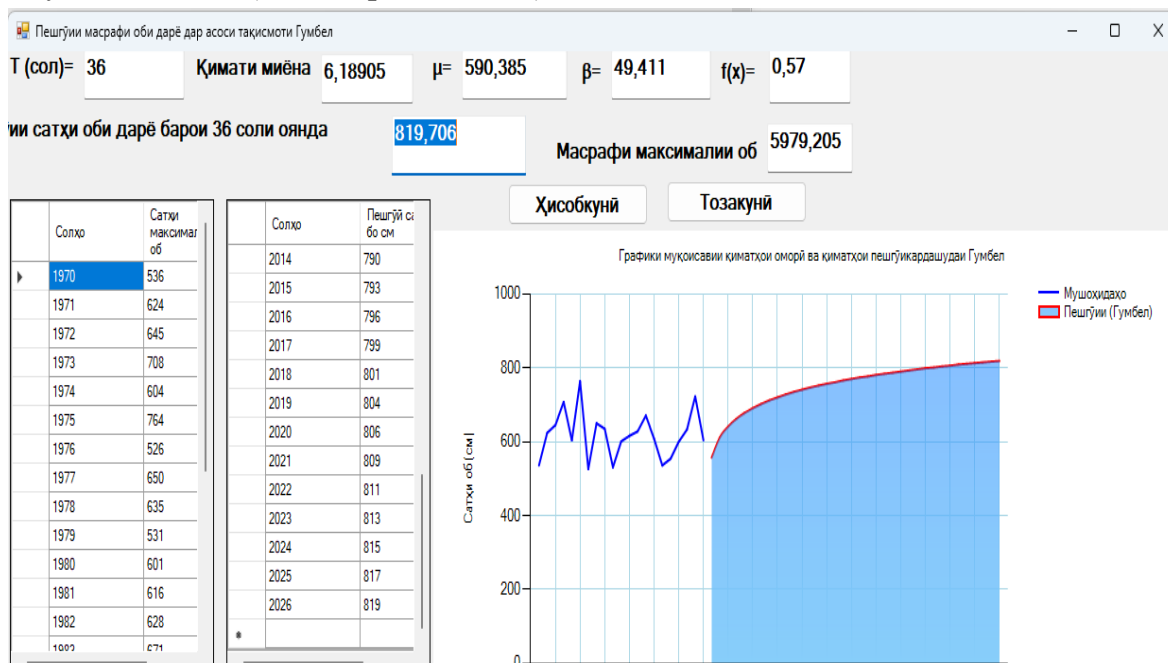
Расми 3.1.3. - Натиҷаи пешгӯии сатҳи оби дарё барои соли 2026
