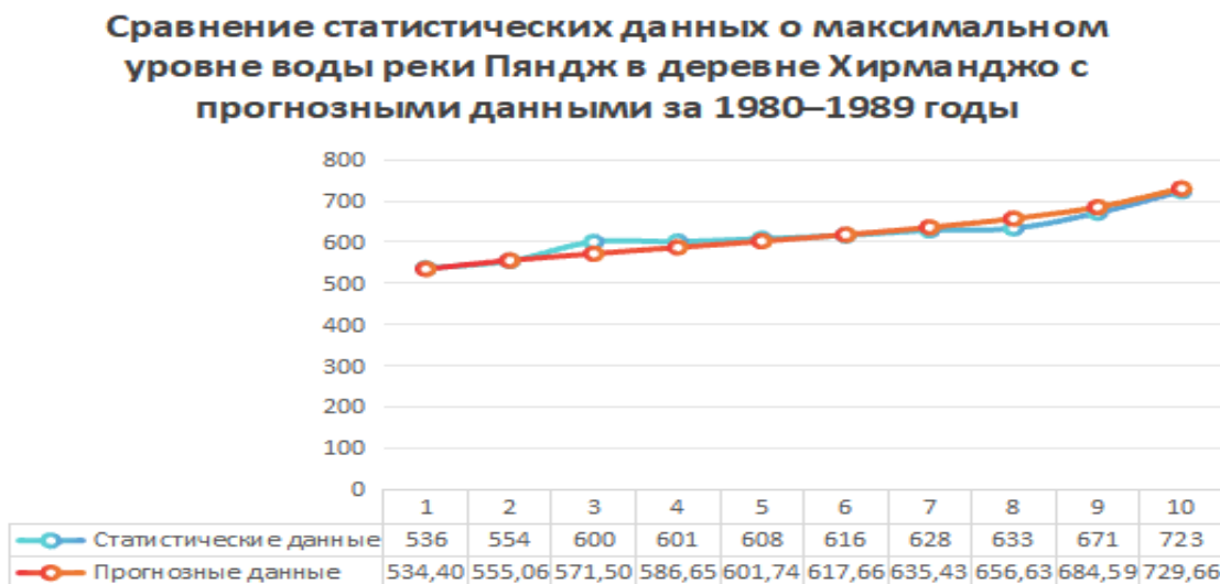
Рисунок 2.6.4. - Сравнение максимальных уровней воды реки Пяндж на основе статистических данных и распределения Гумбеля
