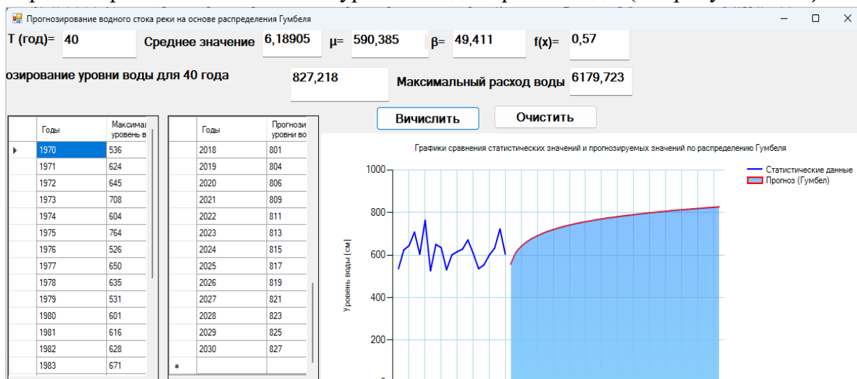
Рисунок 3.1.4. - Прогноз уровней воды в реках на 50-летний период (1990–2040 гг.)
