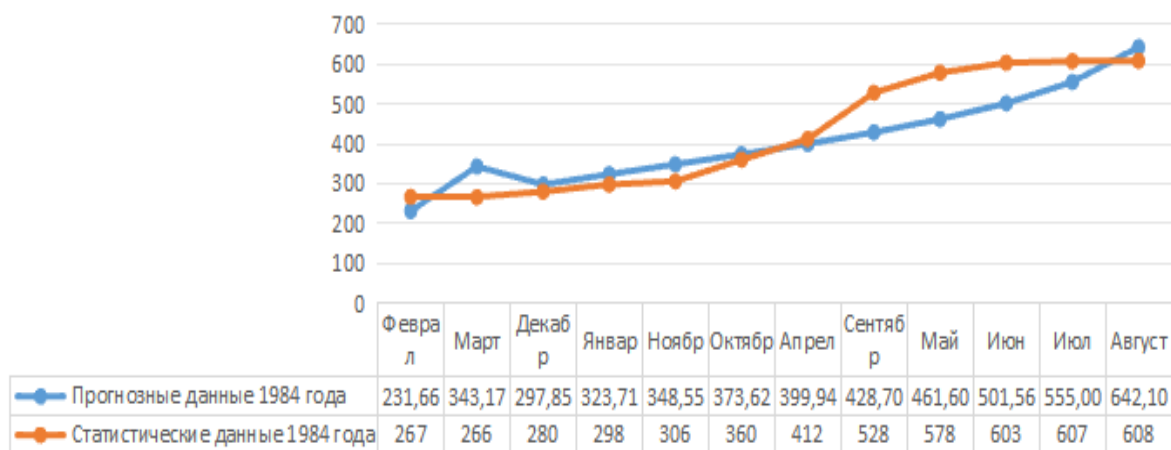
Рисунок 2.6.2. -Сравнение статистических данных и данных, рассчитанных по методу Гумбеля, за 1984 год
