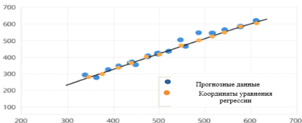
Рисунок 2.6.3. -Сравнение статистических и прогнозных данных, полученных с использованием метода Гумбеля, за 1984 года
