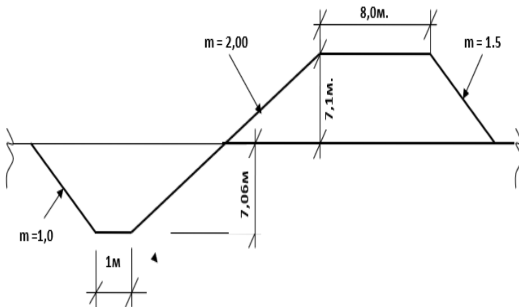
Рисунок 3.1.2. - Проектные параметры плотины
