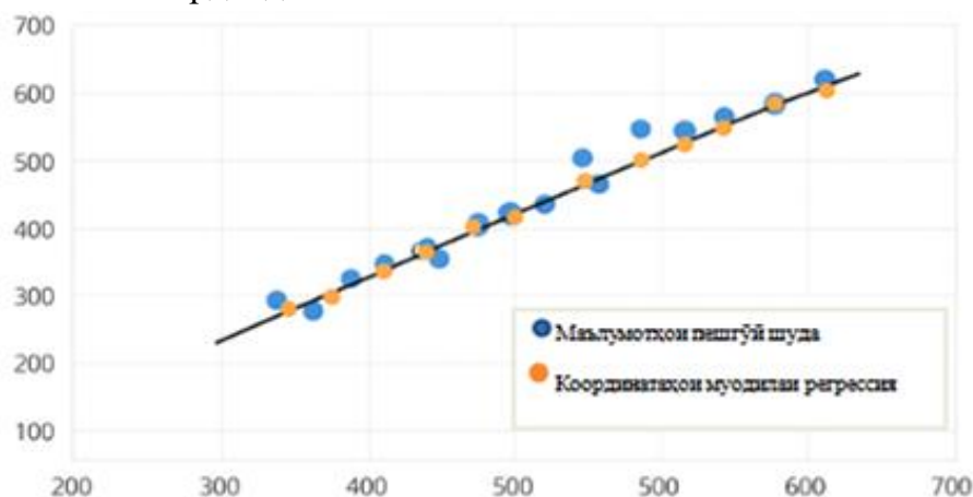
Расми 2.6.3. - Муқоисаи маълумотҳои оморӣ ва маълумотҳои пешгӯишуда бо истифода аз усули Гумбел барои соли 1984
