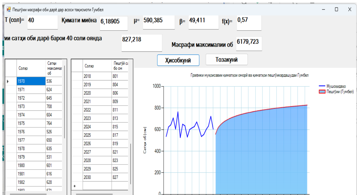
Расми 3.1.4. - Натиҷаи пешгӯии сатҳи оби дарё пас аз 50 сол (1990-2040)
