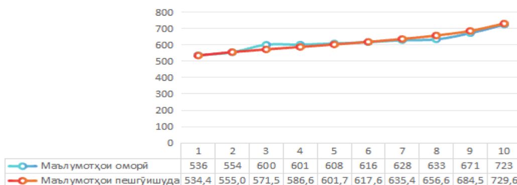
Расми 2.6.4. -Муқоисаи сатҳи максималии оби дарёи Панҷ дар асоси маълумотҳои оморӣ ва тақсироти Гумбел
