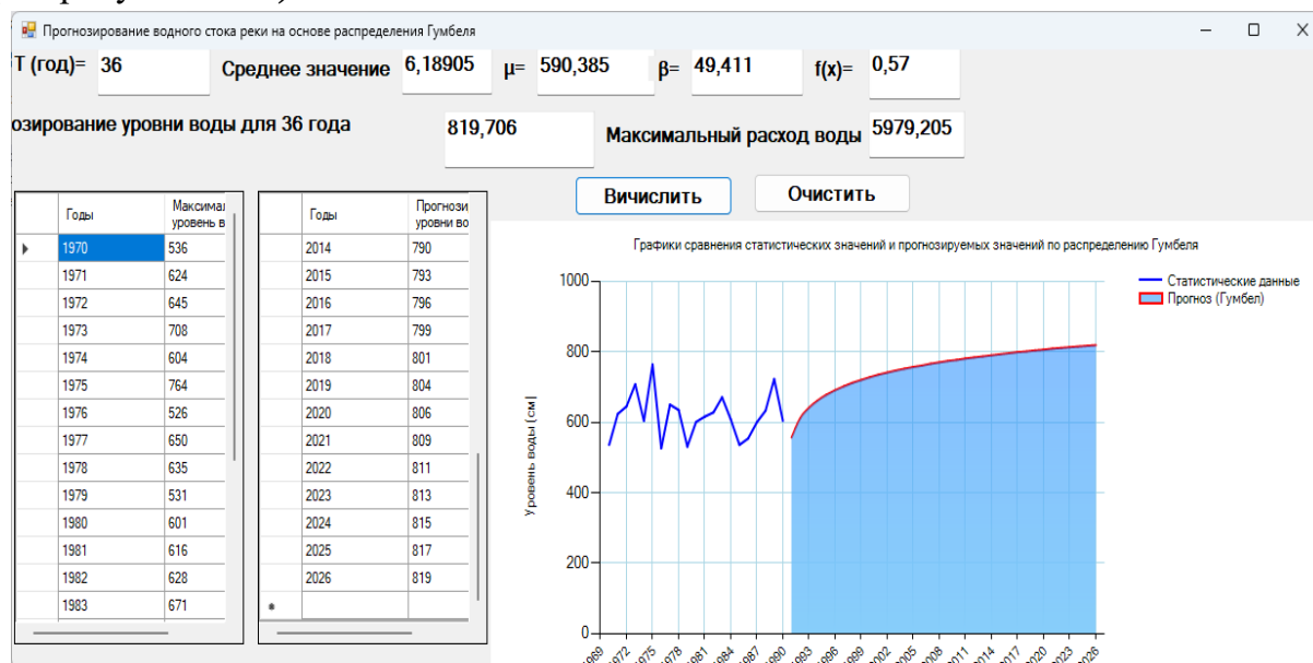
Рисунок 3.1.3. - Результат прогноза уровня воды в реке на 2026 год
