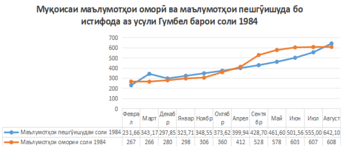
Расми 2.6.2. - Муқоисаи маълумотҳои оморӣ ва маълумотҳои пешгӯӣшуда бо истифода аз усули Гумбел барои соли 1984
