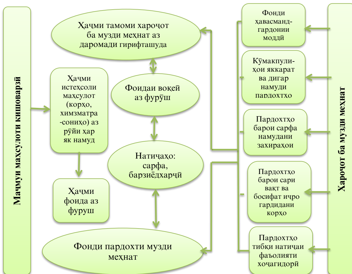
Расми 1. – Амсилаи вобастагии ҳаҷми истеҳсоли маҳсулот ва ташаккули фонди музди меҳнат дар корхонаҳои кишоварзӣ
