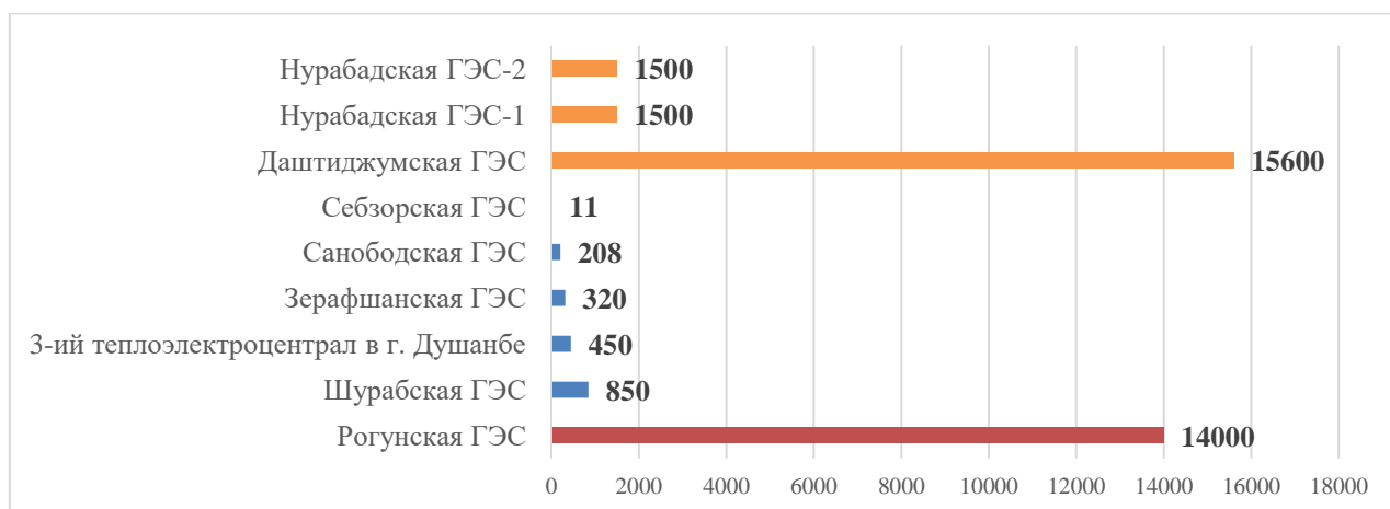
Диаграмма 4.1.2. – Мощности строящихся, планируемые и прогнозируемые на перспективу энергетические проекты, млн. квт. ч./год*
