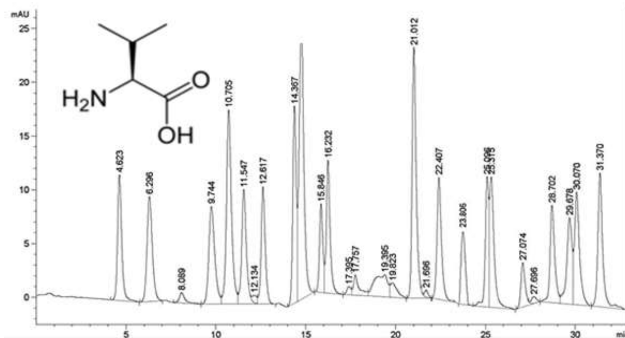
Расми 18. Хроматограммаи (S)-2-амино-3-кислотаи метилбутан (валин)-и аз таркиби мармараки мускатӣ ҷудошуда
