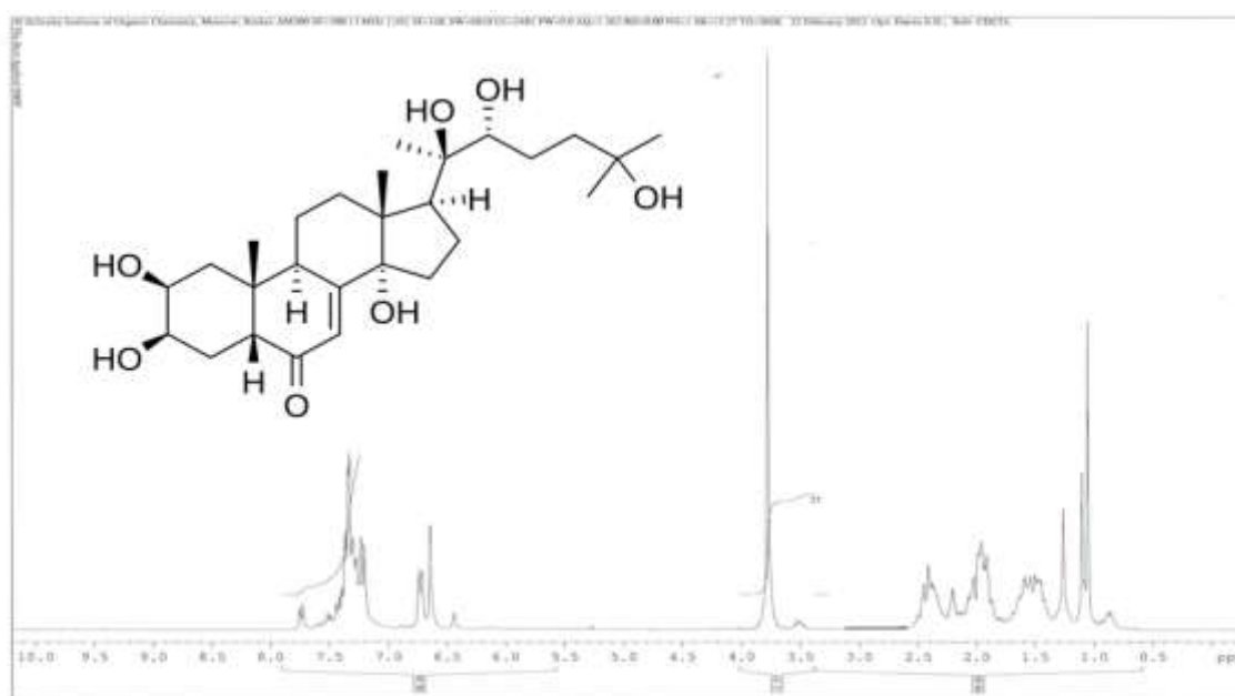
Расми 34- РМП - ки аз таркиби мармараки мускатӣ гирифта шудааст
