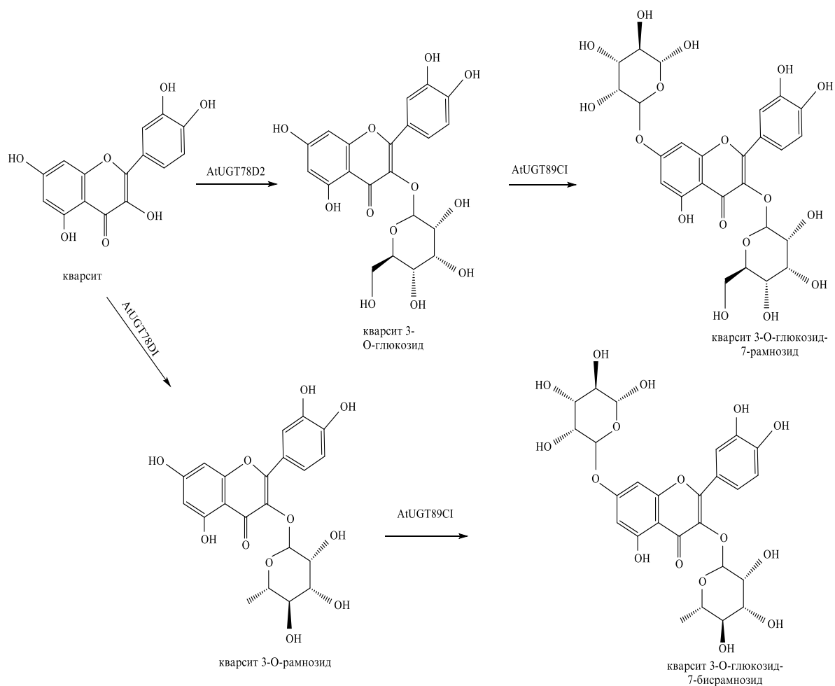
Расми 8. Механизми ҳосилшавии кверсетин-3-О-глюкозид.
