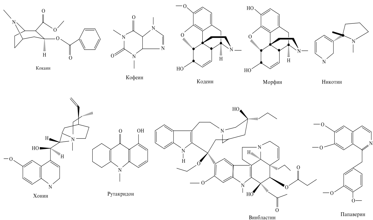
Расми 2. Сохти химиявии алкалоидҳои дар таркиби мармараки мускатӣ мавҷуда
