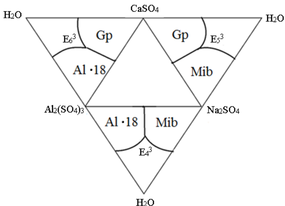
Расми 3. – Диаграммаи «Кушода»-и фазаҳосилшавии системаи \text{Na}^+ , \text{Ca}^{2+} , \text{Al}^{3+} \parallel \text{SO}_4^{2-} - \text{H}_2\text{O} дар сатҳи секомпонентагӣ
