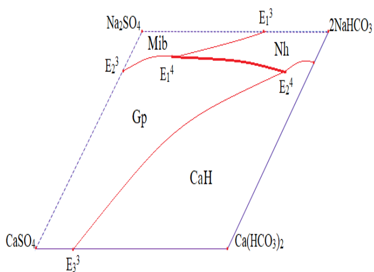
Расми 26. – Системаи тартиби дуҷусти \text{Na}^+ , \text{Ca}^{2+} \parallel \text{SO}_4^{2-} , \text{HCO}_3^- - \text{H}_2\text{O} . Диаграммаи ҳалшавандагӣ дар изотермаи 273 К: а) қисми обӣ-намакӣ; б) қисми намакӣ.
