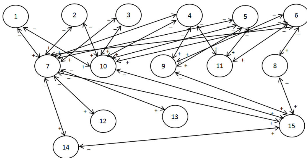
Расми 1.3.3 – ГСА-и экосистемаи бисёрсатҳа «олами растаниҳо - 1, олами алафхӯрҳо - 2, парандагон - 3, моҳиҳо - 4, хазандагон - 5, ҳашарот - 6, ҳояндаҳо - 7, ҳашаротхӯрҳо - 8, тортанакшаклҳо - 9, обҳоиҳо - 10, қанотдастон - 11, пишаки қамишзорӣ - 12, шағол - 13, рӯбоҳ - 14, гург - 15»
