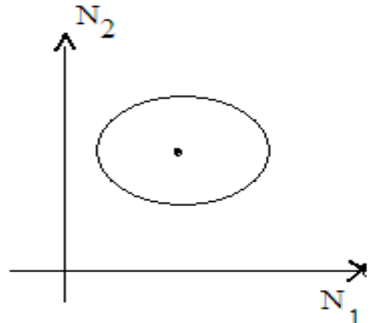
Расми 3.1.1. Тасвири геометрии амсилаи «даранда ва сайди ӯ».
