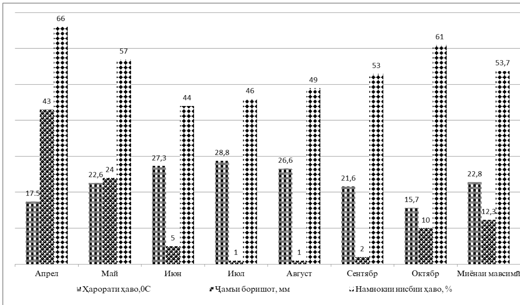
Расми 2.1.-Маълумотҳои миёнаи бисёрсолаи вазъи ӯбу ҳавои минтақаи Вахш дар давоми солҳои таҳқиқот
