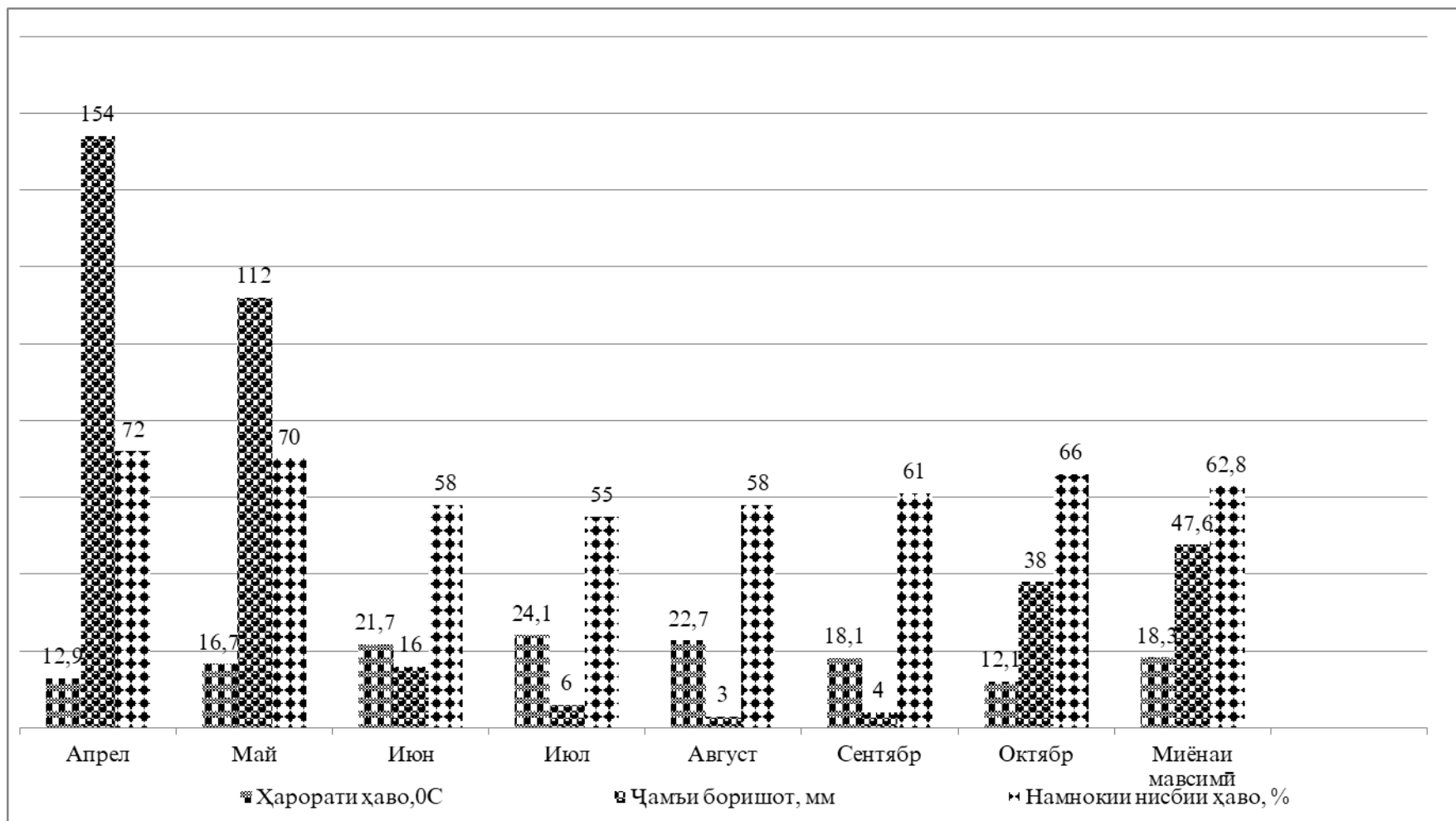
Расми 2.3. -Маълумотҳои миёнаи бисёрсолаи минтақаи Мӯъминобод
