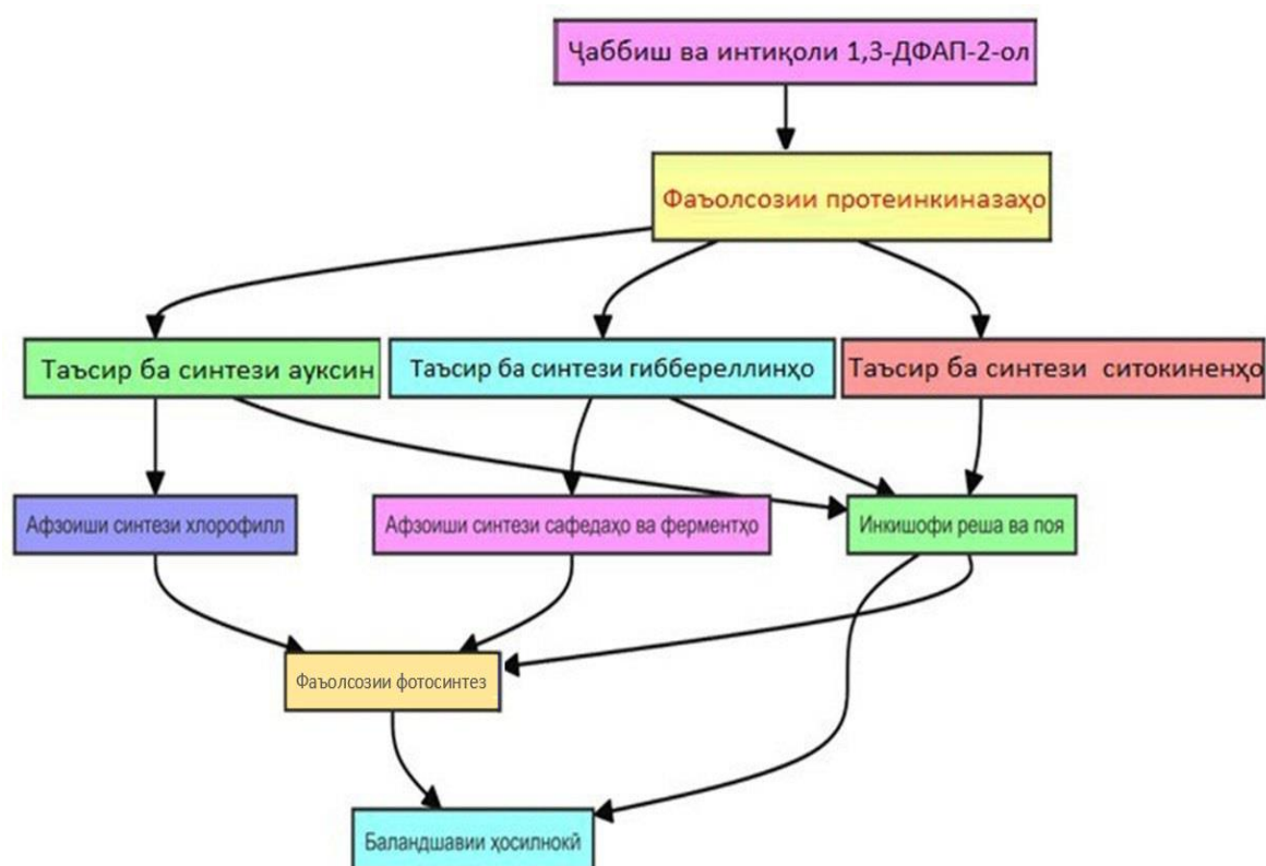
Расми 3.20. Нақшаи механизми таъсири 1,3-дифталила- ланилопропан–2–ол ба лӯбиё ( Phaseolus vulgaris L.) ҳамчун афзоиштанзимкунанда
