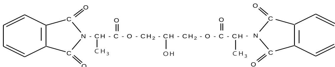
Расми 2.12. Формулаи химиявии 1,3–дифталилаланилопропан–2–ол
