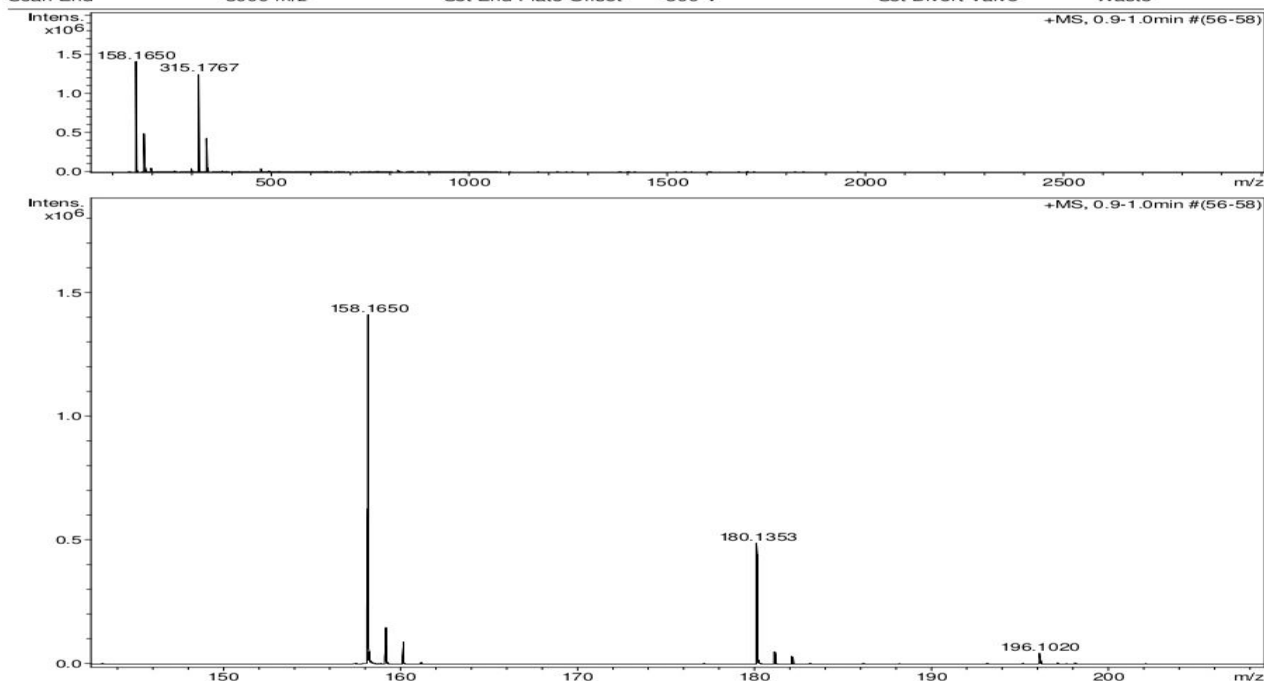
Расми 3.19. Масс–спекторӣ лӯбиё ( Phaseolus vulgaris L.) баъд аз коркард бо 1,3–дифталилаланилопропан–2–ол
