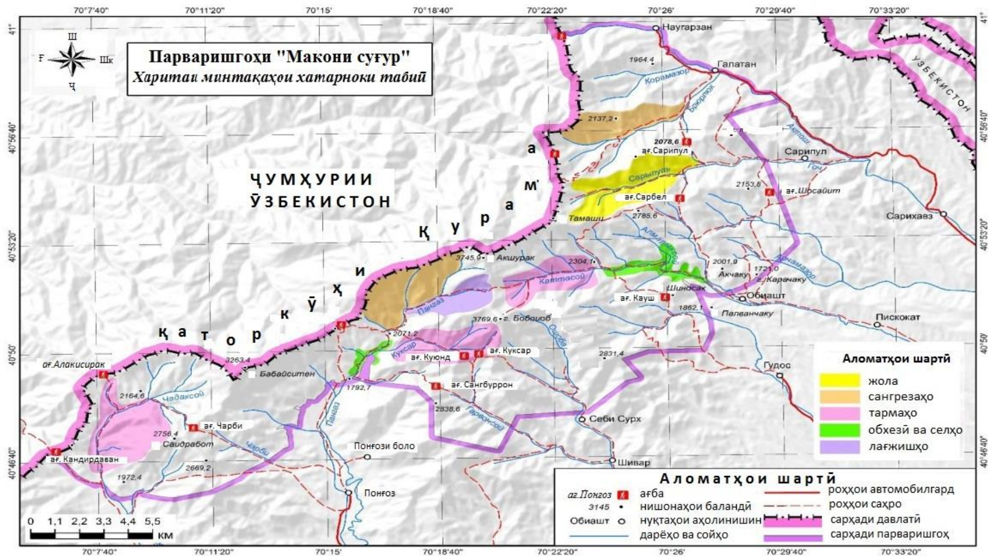
Расми 3.7. - Харитаи хатарҳои табиӣ дар парваришгоҳи «Макони суғур»
