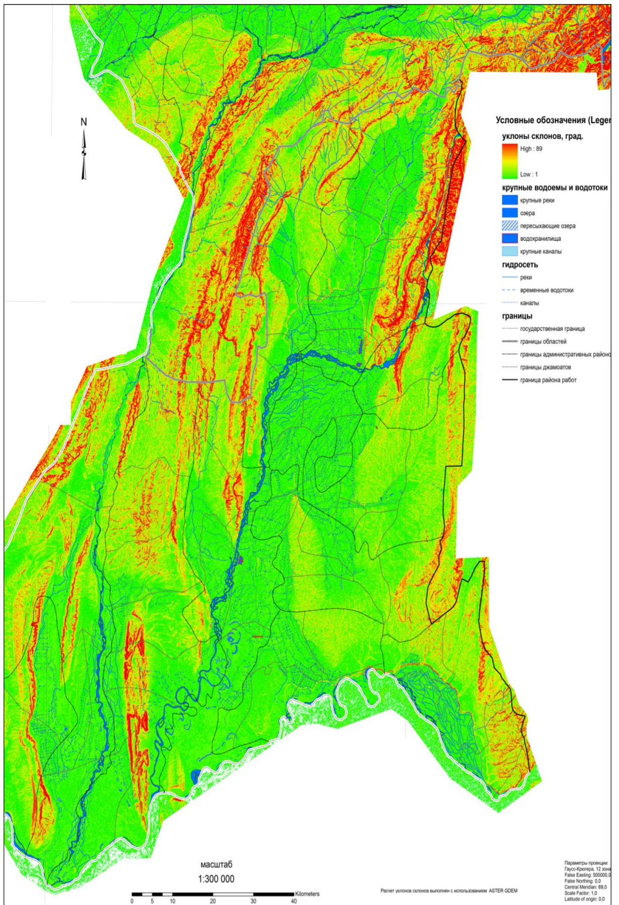
Рисунок 2.1.5.1. - Карта уклонов склонов Вахш-Кафирниганской зоны (Шарифзода М.И.)
