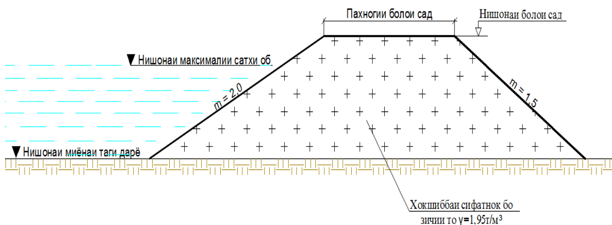
Расми 1.3.1. - Бурриши кундалангии мустаҳкамкунӣ бо усули қуму шағал
