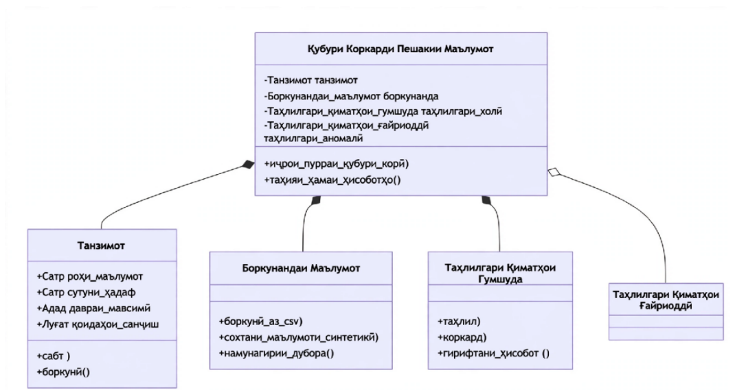
Расми 1.1.7. - Диаграммаи UML-и синфҳо, ки чузъҳои калидии система ва робитаҳои онҳо ро инъикос менамояд
