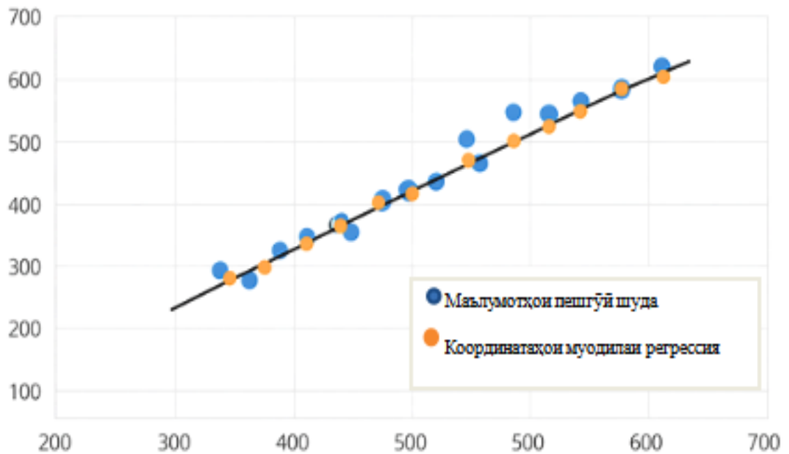
Расми 2.6.2. - Муқоисаи маълумотҳои оморӣ ва маълумотҳои пешгӯишуда бо истифода аз усули Гумбел барои соли 1984
