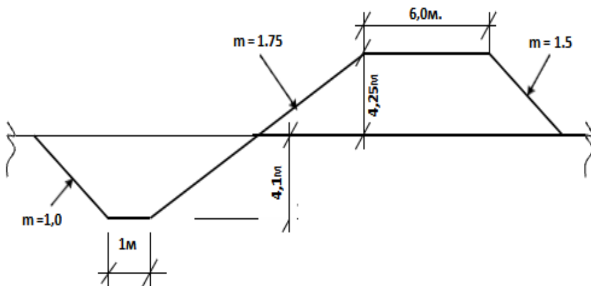
Расми 3.3.1. - Параметрҳои лоиҳавии садд
