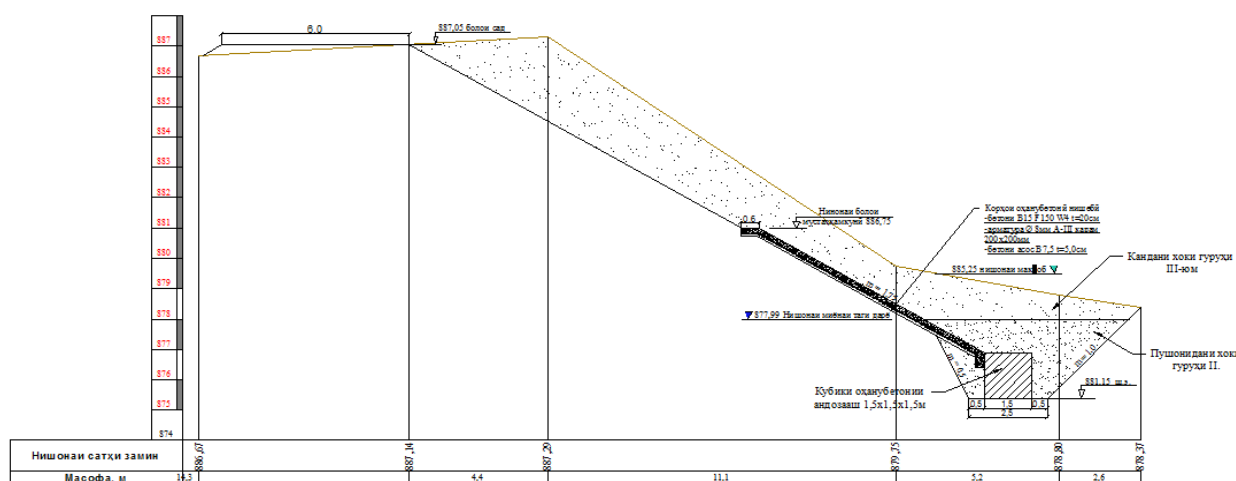
Расми 1.2.5. - Бурриши кундалангии минтақа дар дарёи Лучоб (ноҳияи Рудақӣ)
