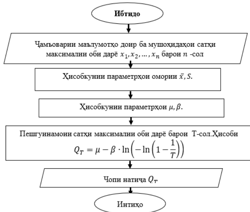
Расми 3.1.2. - Блок-схемаи алгоритми пешгӯии сатҳи экстремалии оби дарё бо истифода аз модели Гумбел дар асоси мушоҳидаҳои сатҳи максималии солҳои оби дарёи Панҷ дар дидбонгоҳи деҳаи Хирманчо
