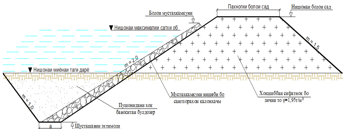
Расми 1.3.2.- Бурриши кундалангии мустаҳкамкунӣ бо усули сангҳои калонҳаҷм
