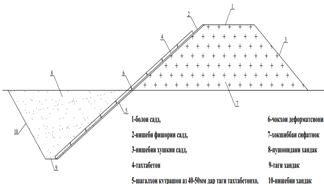
Расми 3.5.4. - Бурриши кундалангии канструксияи қабулкардашуда
