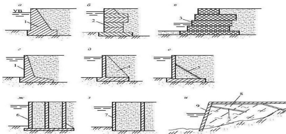
Расми 1.2.2. - Деворҳои вертикалӣ
