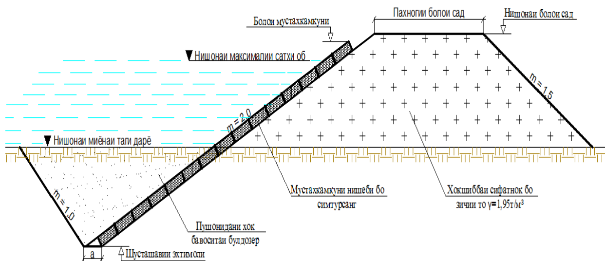
Расми 1.3.5. - Бурриши кундалангии мустаҳкамкунӣ бо усули симтурсанг
