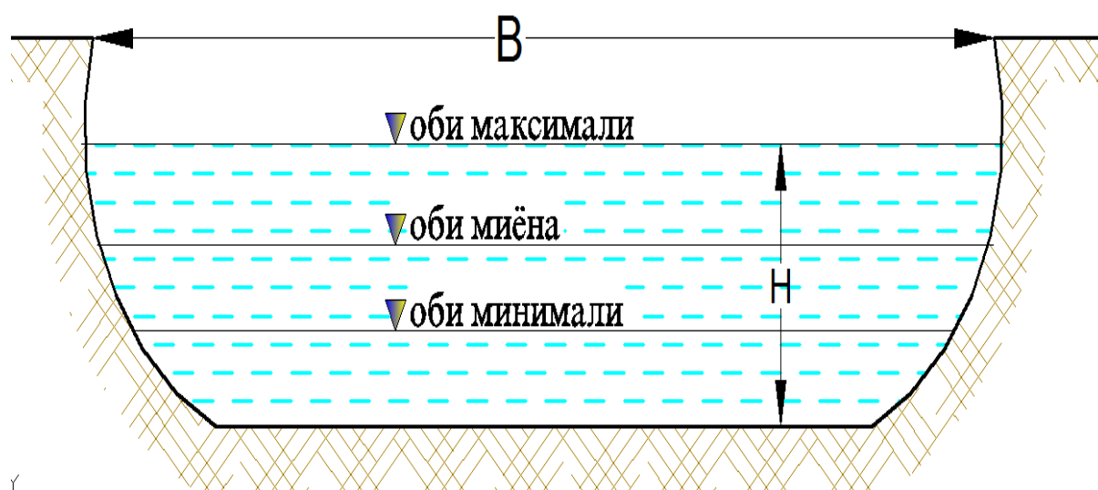
Расми 3.4.1. - Бурриши кундалангии дарё, ки ду тарафи он мустаҳкам карда шудааст
