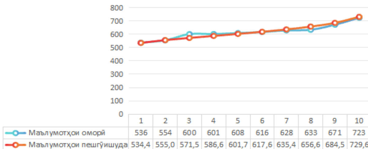
Расми 2.6.3. - Муқоисаи сатҳи максималии оби дарёи Панҷ дар асоси маълумотҳои оморӣ ва тақсими Гумбел
