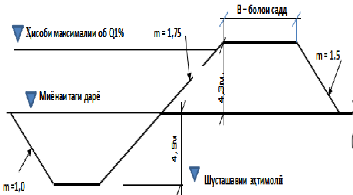
Расми 3.4.3. - Параметрҳои лоиҳавии садд дар минтақаи мазкур
