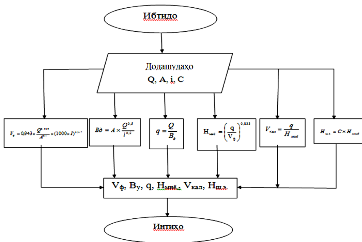
Расми 3.1.5. -Блок-схемаи ҳисоби масрафи масолеҳи соҳилмустаҳкамкунӣ
