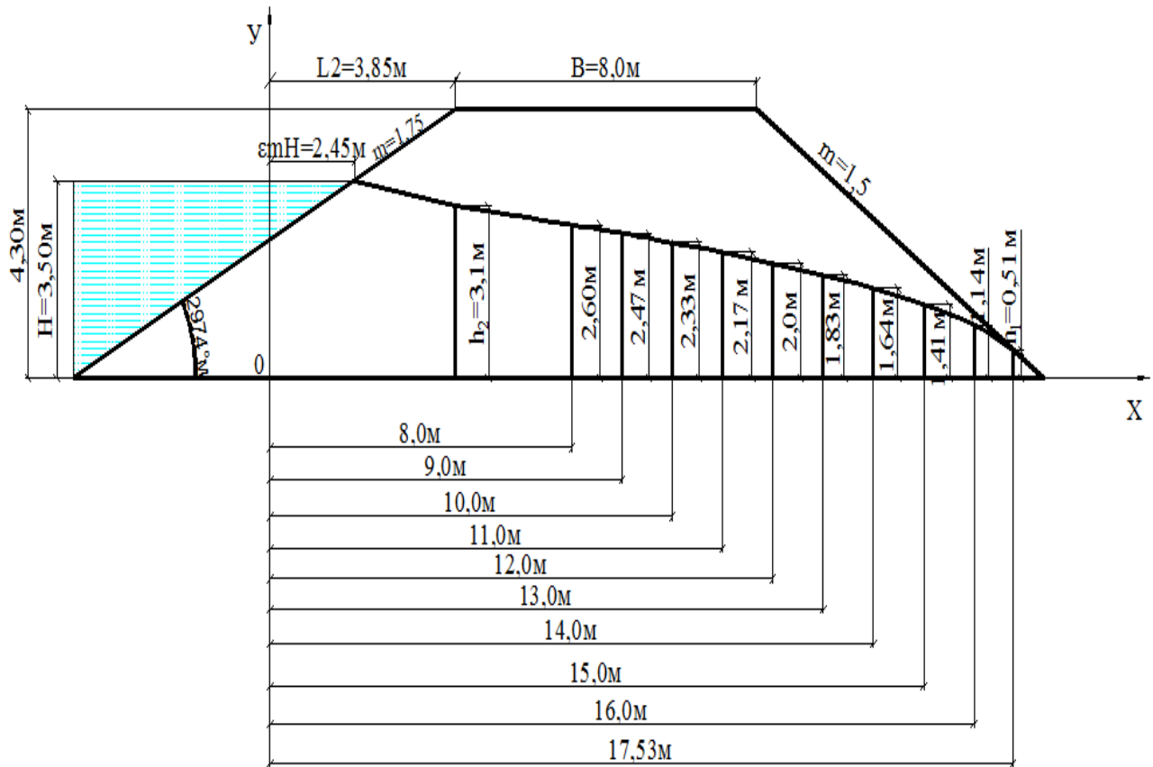
Расми 3.5.1. - Полоиш дар садд
