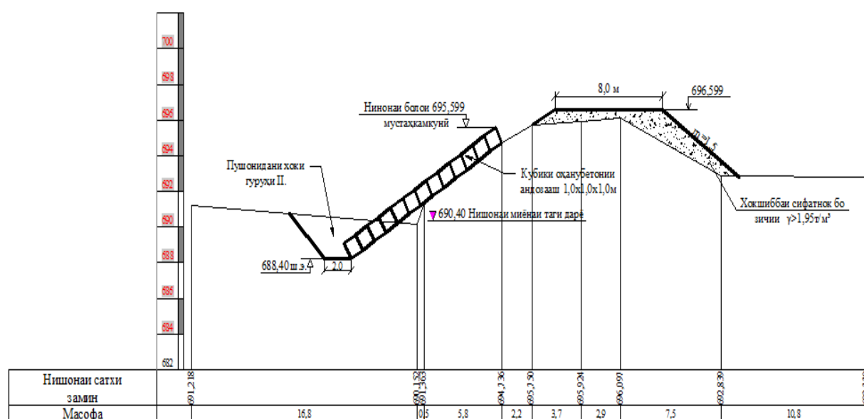
Расми 1.2.10. -Бурриши кундалангии минтақаи деҳаи Хиртароши ҷамоати Зайнабободи ноҳияи Рӯдакӣ
