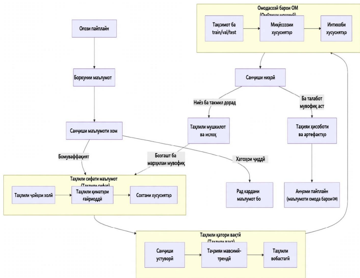
Расми 1.1.6. - Блок-нақшаи муфассали алгоритми кори раванди коркард бо нуқтаҳои назорати сифат
