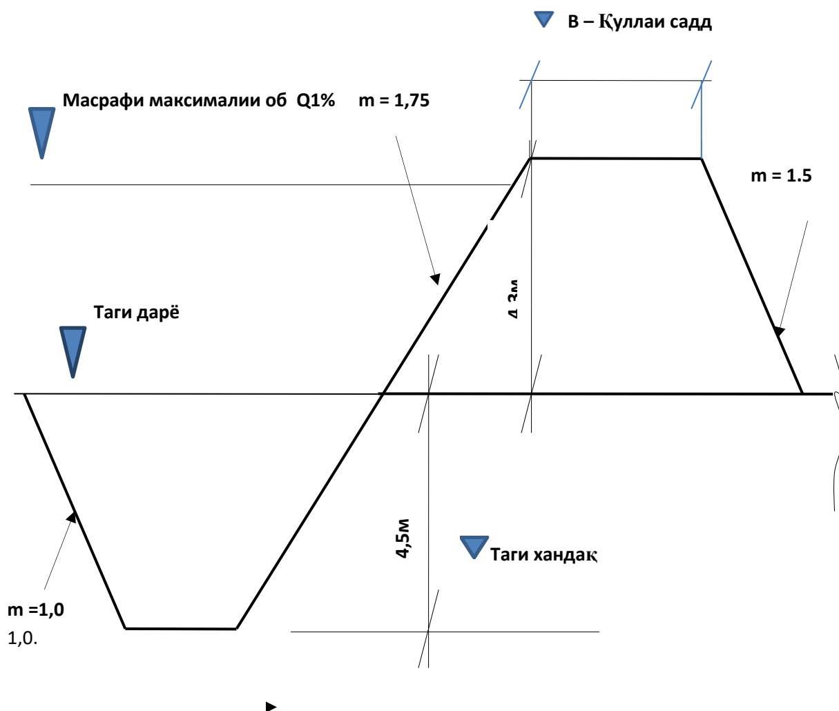
Расми 3.5.3. - Параметрҳои лоиҳавии садд
