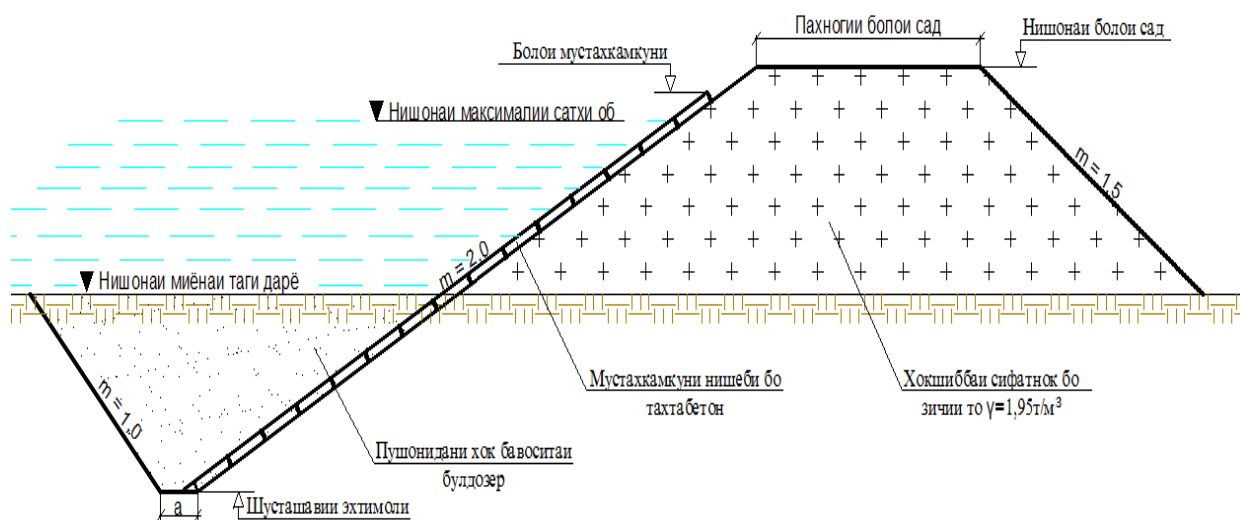
Расми 1.3.4. - Бурриши кундаланги мустаҳкамкунӣ бо усули тахтабетон
