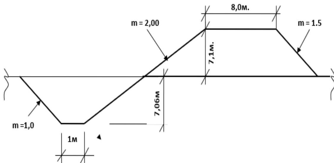
Расми 3.1.2. - Параметрҳои лоиҳавии садд
