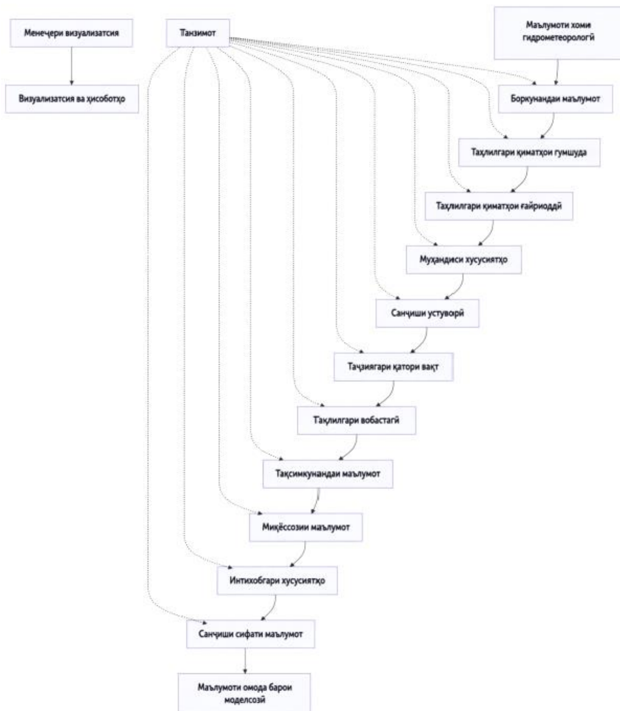
Расми 1.1.5. - Архитектураи умумии раванди пайдарпайи модули пешкоркарди қаторҳои замони гидрометеорологӣ
