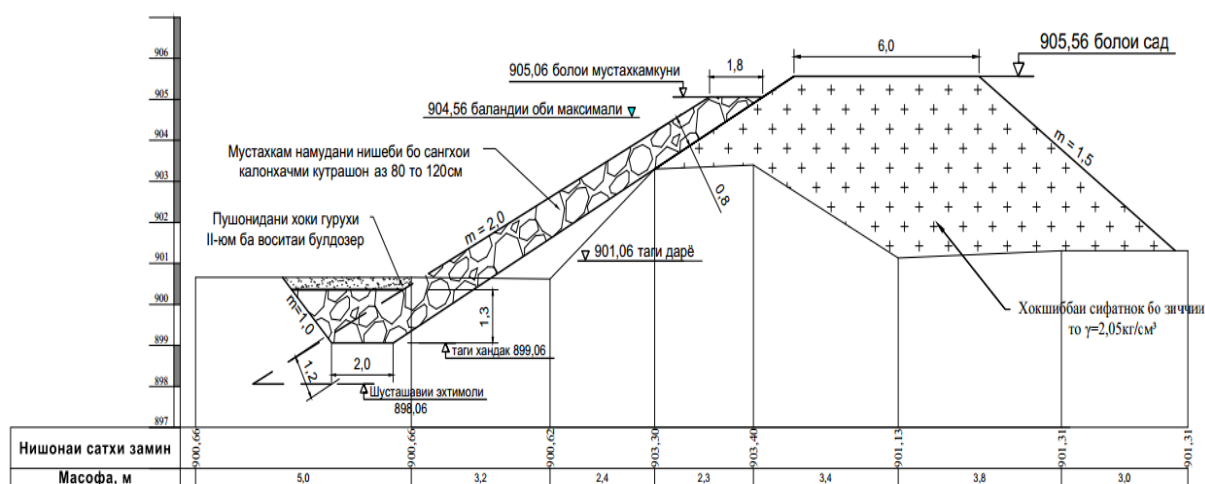
Расми 1.2.4. - Бурриши кундалангии минтақа дар дарёи Зарафшон
