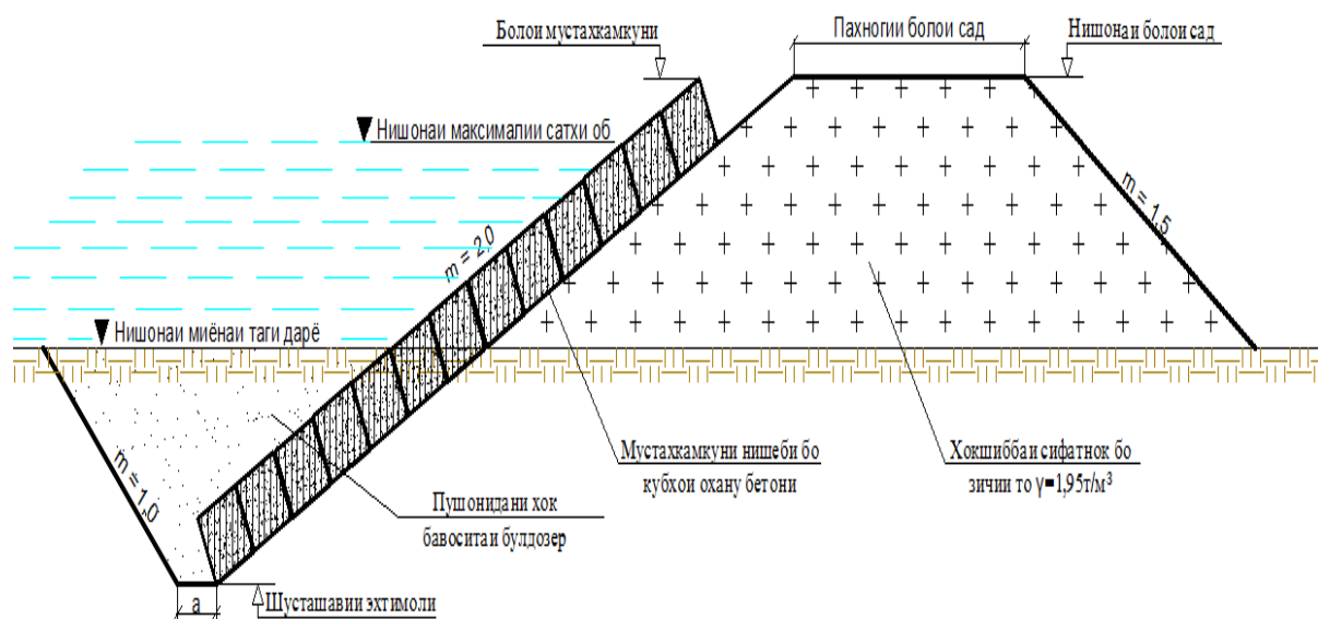
Расми 1.3.3. - Бурриши кундалангии мустаҳкамкунӣ бо усули кубикҳои оҳанубетонӣ
