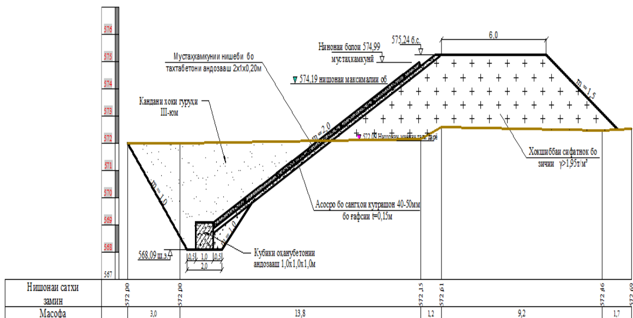
Расми 1.2.6. - Бурриши кундалангии минтақа дар дарёи Қизилсу дар деҳаи Кӯчабоғи ноҳияи Восеъ
