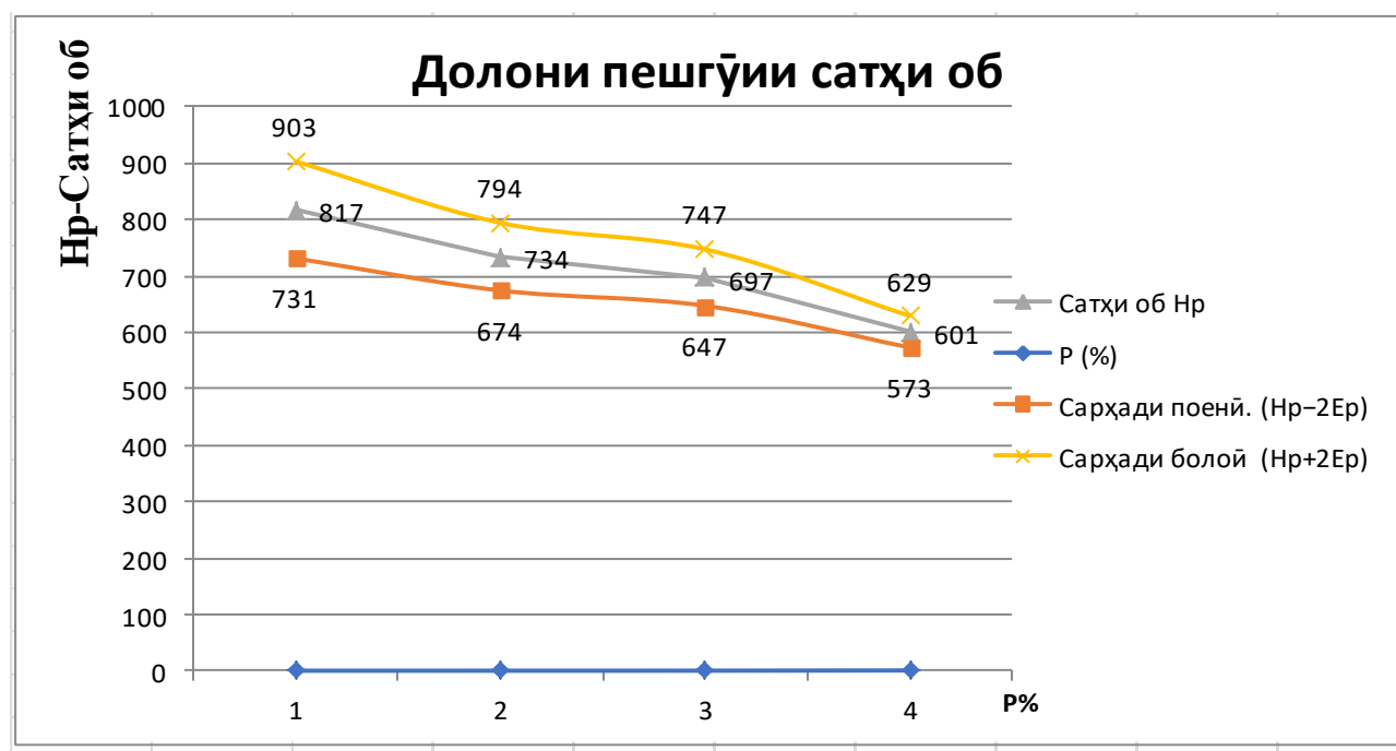
Расми 2.5.1. - Сарҳадҳои поёӣ ва болоӣ сатҳи об
