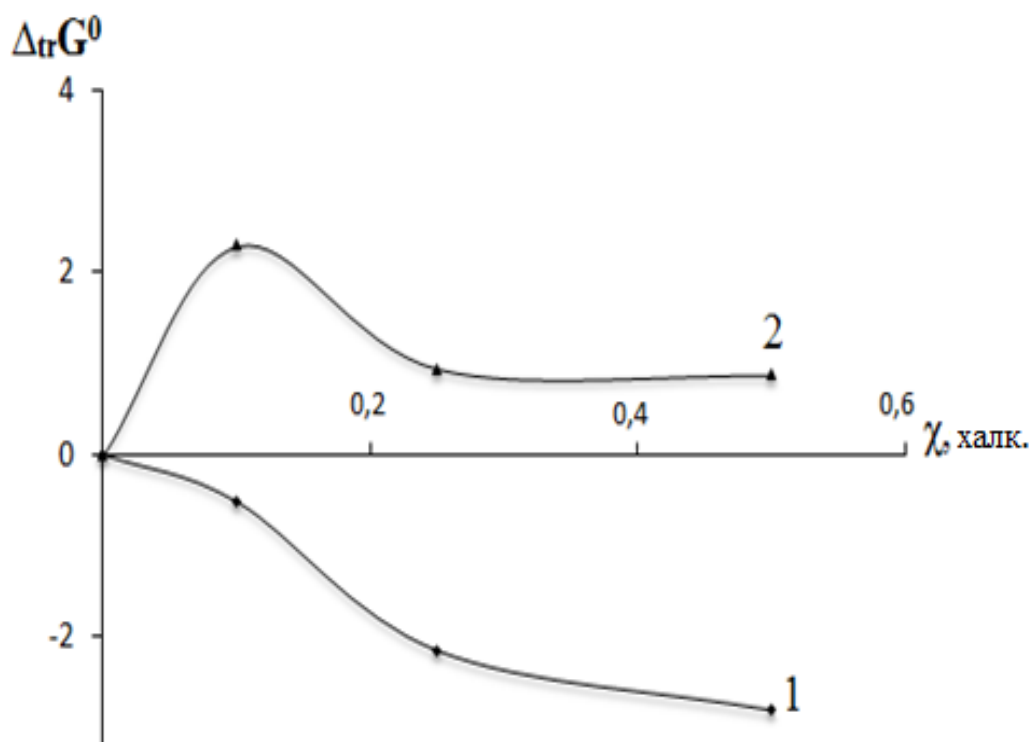
Расми 2.5. - Вобастагии \Delta_{tr}G^0 1МИ дар ҳалкунандаи обӣ-ДМСО (1) ва обӣ-этанолӣ (2)
