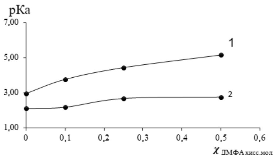
Расми 2.13. -Вобастагии pK_a=f(\chi_{\text{ДМФА}}) : 2-меркаптоимидазол (1), 1-метил-2-меркаптоимидазол (2)
