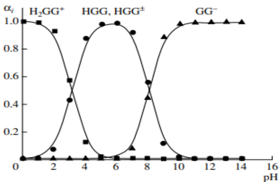
Расми 1.7. - Диаграммаи тақсимшавии глитсинглитсин аз рН
