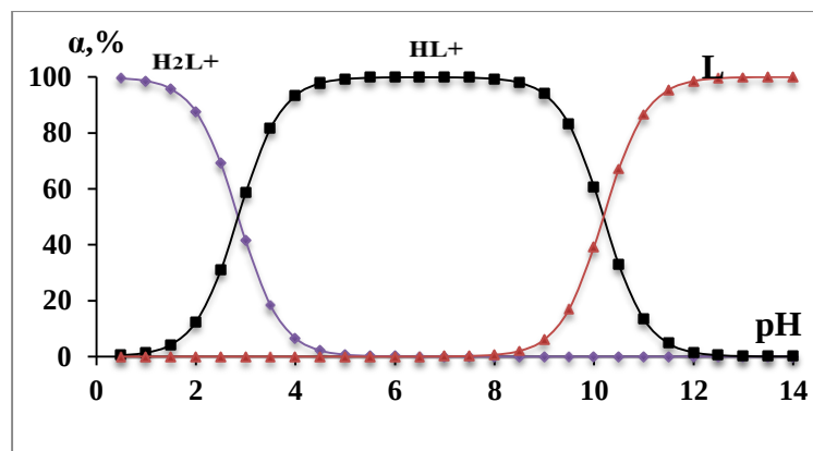
Расми 1.5. -Диаграммаи тақсимшавии метилгитсин дар ҳарорати 298,15К
