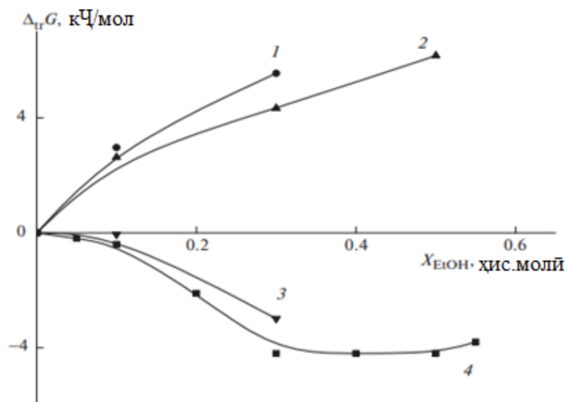
Расми 1.3. -Таъсири ҳалқунандаи обӣ-этанолӣ ба тағйирёбии энергияи Гиббси гузариши реаксия ва солвататсияи реагентҳо, диссоциатсияи триглицин 1- \Delta_{tr}G(HL) ; 2- \Delta_{tr}G_r ); 3- \Delta_{tr}G_r(H_2L^+) ; \Delta_{tr}G(H^+) ;
