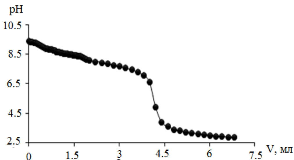
Расми 2.6. - Вобастагии pH аз V_{HCl} барои маҳлули обии 2-этилимидазол дар 298,1К
