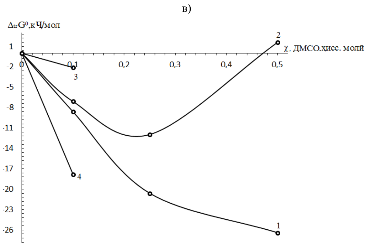
Расми 4.3. (а, б, в) -Саҳми солвататсияи реагентҳо дар тағйирёбии энергияи Гиббси гузариши реаксияи комплексҳосилшавии нуқра (I) бо 2МИ дар ҳалқунанда обӣ-ДМСО
