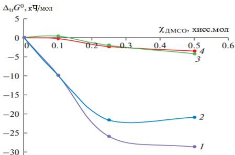
Расми 2.16. - Тағйирёбии энергияи Гиббси гузариш аз об ба ҳалкунандаи обӣ-ДМСО барои 1- \Delta_{tr}G^0 [1MI] + ; 2- \Delta_{tr}G^0 H + ; 3- \Delta_{tr}G^0 ; 4- \Delta_{tr}G^0 1MI
