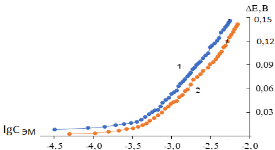
Расми 4.9. -Вобастагии \Delta E аз \lg C_{\text{ЭМ}} барои комплексҳои нукра (I) бо 2-этилимидазол дар об: 1-298,15 2-308,15K
