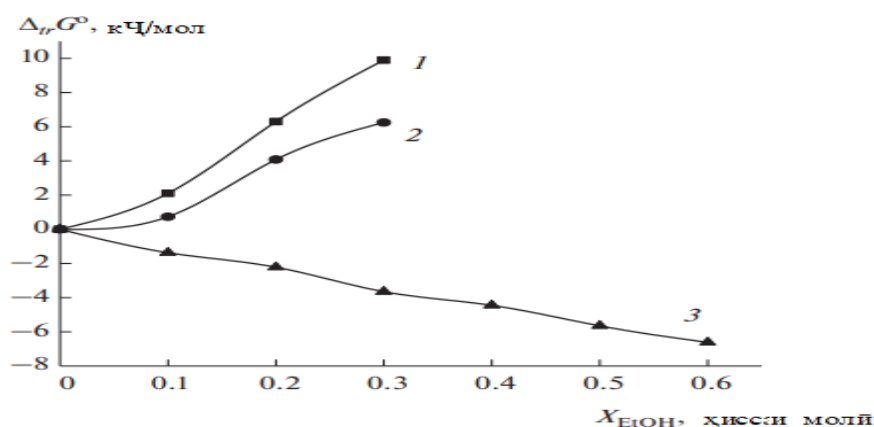
Расми 1.10. -Таъсири таркиби ҳалкунандаи обӣ-этанолӣ ба энергияи Гиббси гузариши реаксияи ҳосилшавии глитсинглитсинати кобалт(II):
