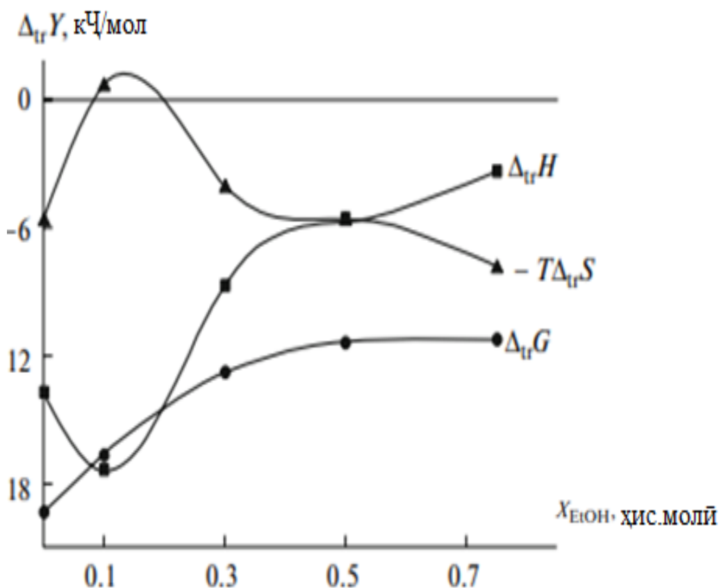
Расми 1.4. -Тағйирёбии энергияи Гиббс, энатлпия ва энтропия барои реаксияи протонизатсияи никатинамид дар маҳлули обӣ-этанолӣ
