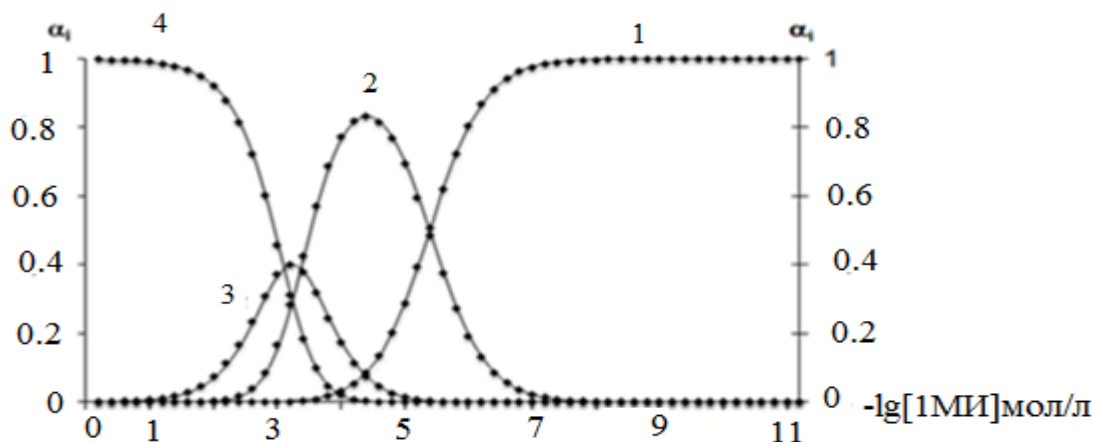
Расми 3.5. - Качаттаҳои тақсимоти комплексҳои 1-метил-2-меркаптоимидазолии нукра (I) дар ҳалкунандаи оби-этанолӣ, ки 0,10 ҳиссаи молии этанол дорад: 1- [\text{Ag}]^+ ; 2- [\text{Ag}(\text{1МИ})]^+ ; 3- [\text{Ag}(\text{1МИ})_2]^{2+} ; 4- [\text{Ag}(\text{1МИ})_3]^{3+} . T=298,15\text{K}
