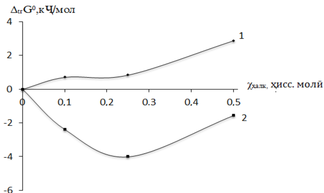
Расми 4.2. -Солвататсияи 2МИ дар ҳалқунандаи 1-обӣ-этанолӣ; 2-обӣ-ДМСО
