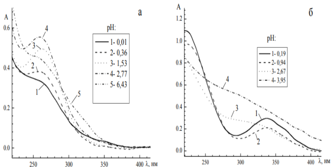
Расми 1.1. - Спектри фурубавии пайвасти Fe(III)-ОЭДФ (а) ва Fe(III) дар ҳудуди гуногуни рН
