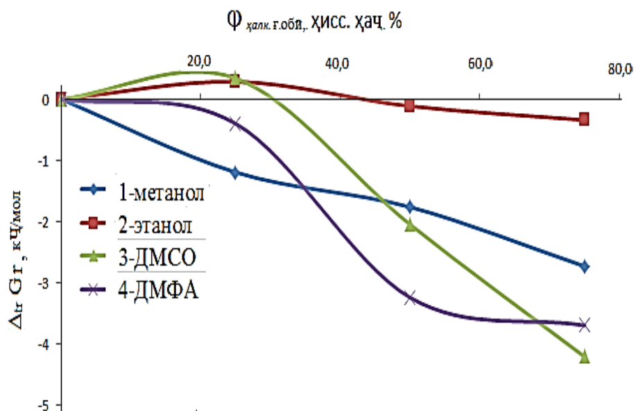
Расми 2.14. -Тағйирёбии энергияи Гиббси ( \Delta_{tr}G^0 ) гузариши реаксияи протонпайвастунии 1МИ ҳангоми гузаштан аз об ба ҳалқунандаи обӣ-органикӣ
