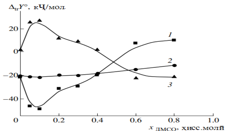
Расми 1.11. -Тавсифҳои термодинамикии реаксияи ҳосилшавии монокомплексии нукра(П) бо 2,2-дипиридил дар ҳалқунандаи обӣ-ДМСО. 1- \Delta_{r1} H^\circ , 2-- \Delta_{r1} G^\circ , 3- T\Delta_{r1} S^\circ
