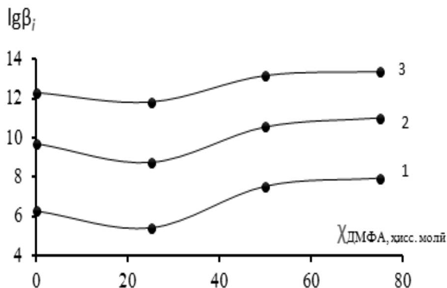
Расми 3.6. –Вобастагии \lg\beta_i аз \chi_{\text{ДМФА}} барои комплексҳосилшавии нукраи (I) бо 1-метил-2-меркаптоимидазол дар маҳлули обӣ ва консентратсияҳои гуногуни ДМФА: 1-[Ag(1МИ)] + , 2-[Ag(1МИ) 2 ] + ва 3-[Ag(1МИ) 3 ] +
