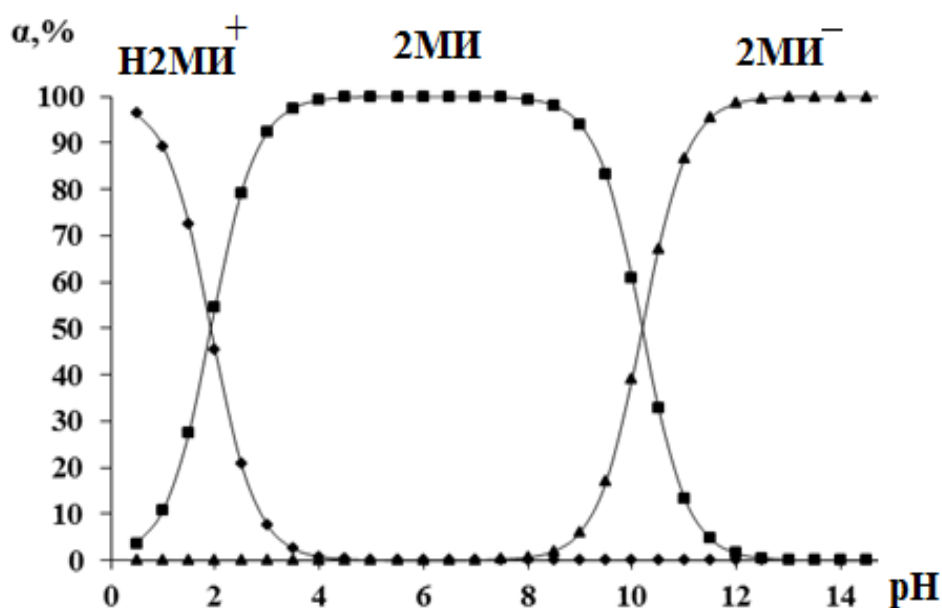
Расми 2.8. -Ҳиссаи тақсимшавии шаклҳои гуногуни 2МИ (молекулавӣ, протонизатсияшуда ва депротонизатсияшуда) дар маҳлули обӣ. T=298\text{K}
