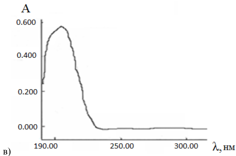
Расми 2.1. - Спектри фурӯбарии: а) 2-меркаптоимидазол; б) 1-метил-2-меркаптоимидазол; в) 2-метиylimидазол; C_L=0.0001 мол/л. pH=6,94
