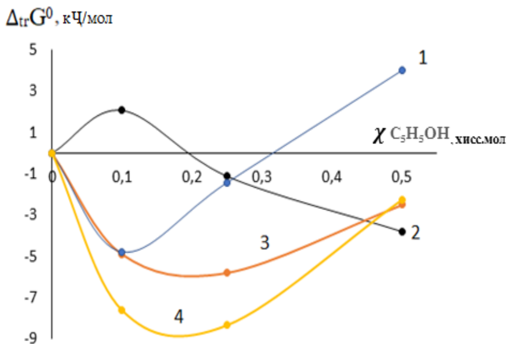
Расми 2.20. -Тағйирёбии энергияи Гиббси гузариш аз об ба ҳалқунандаи обӣ-спиртӣ барои 1- \Delta_{tr}G^0 ; 2- \Delta_{tr}G^0_{2ЭИМ} ; 3- \Delta_{tr}G^0_{H^+} ; 4- \Delta_{tr}G^0_{[H_2ЭИМ]^+}
