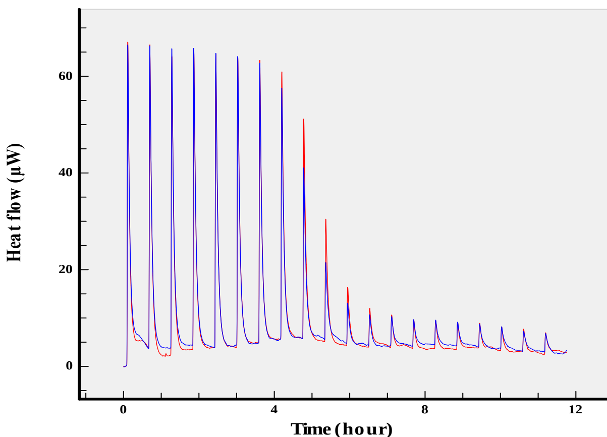
Расми 3.3. - Графики калиборвӣ. Вобастагии миқдори гармӣ аз вақт
