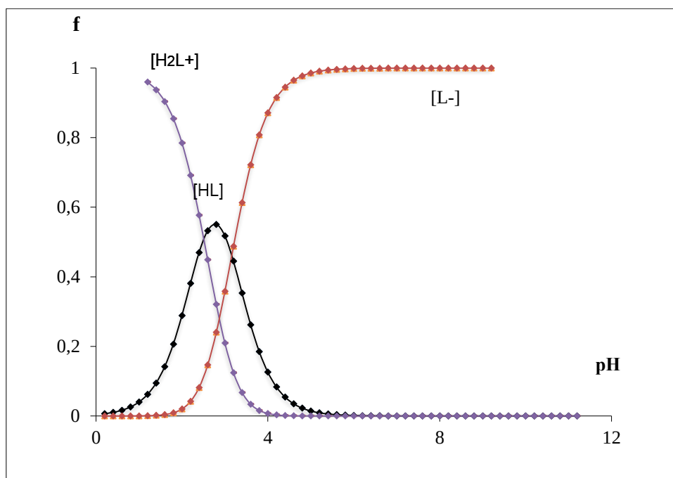
Расми 1.2. - Диаграммаи тақсимшавии 10-карбоксиметил-9-акридон дар ҳудудҳои гуногуни рН
