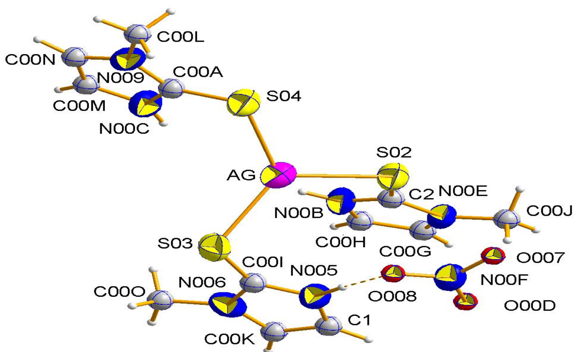
Расми 5.2. - Сохтори молекулавии [Ag(1MI)_3]NO_3 бо схемаи рақамгузории атомҳо
