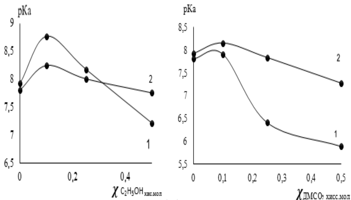
Расми 2.11. -Вобастагии pK_a = f(\chi_{\text{ҳалқунанда}}) : 2-метилимидазол (1), этилимидазол (2)
