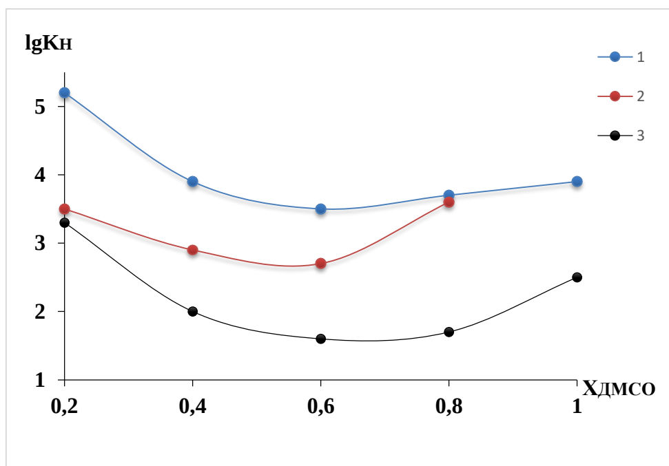
Расми 1.6. - Таъсири ҳалкунандаи обӣ-ДМСО ба собитаи протонизатсияи 1-придин, 2-кислотаи изоникатинат ва 3-никатинамид
