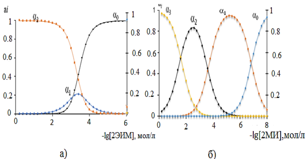
Расми 3.2. -Диаграммаи тақсимшавии пайвастиҳои комплекси нукра(І) бо ҳосилаҳои имидазол дар 298,15К:
