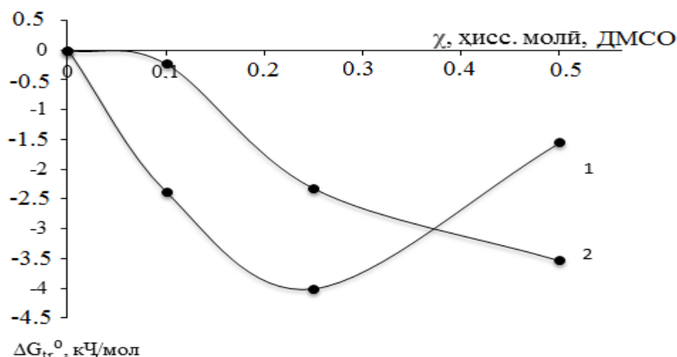
Расми 4.6. -Тағйирёбии энергияи Гиббс ҳангоми гузариши 2-меркаптомидазол (1) ва 1-метил-2-меркаптомидазол (2), аз об ба ҳалқунандаҳои обӣ-диметилсулфоксидӣ дар 298,15K
