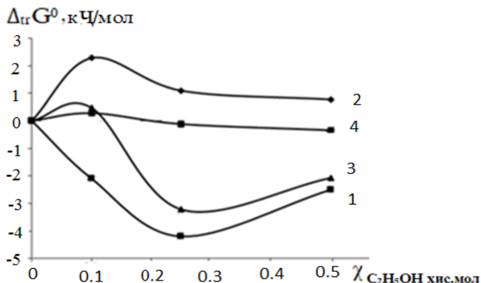
Расми 2.15. - Тағйирёбии энергияи Гиббси гузариш аз об ба ҳалқунандаи обӣ-этанолӣ барои: 1- \Delta_{tr}G^0_{H^+} ; 2- \Delta_{tr}G^0_{1MI} ; 3- \Delta_{tr}G^0_{[H1MI]^+} ; 4- \Delta_{tr}G^0_I
