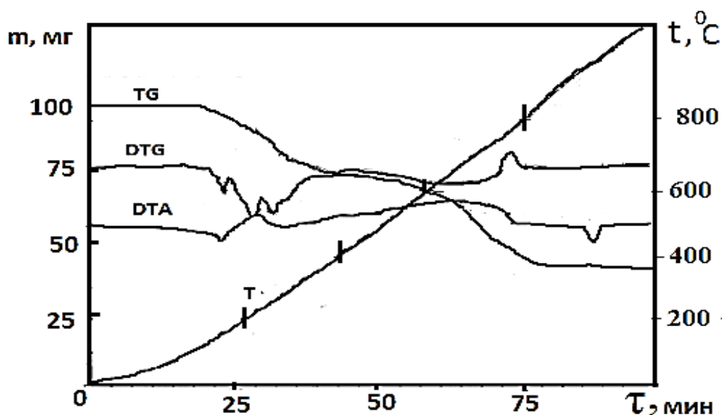
Расми 5.3. - Термогравиграммаи пайвасти комплекси таркибаш [Ag(1-МИ)_2]NO_3 \cdot H_2O
