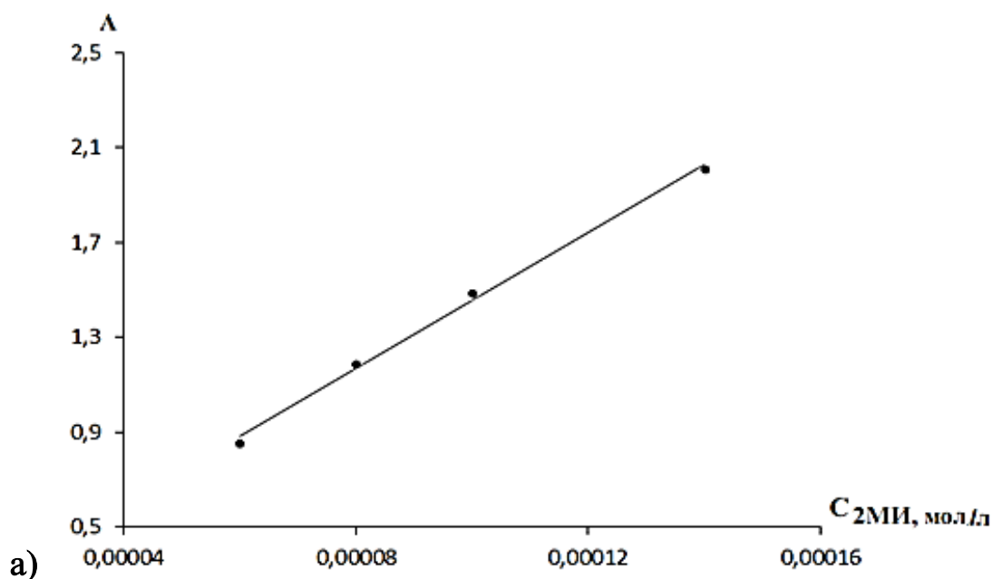
Расми 2.2. -Графики вобастагии зичии оптикӣ аз консентратсияи 2МИ. T=298K . pH=6.94
