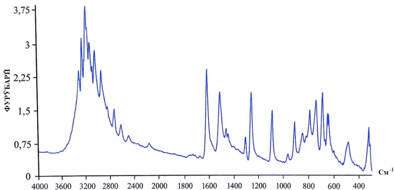
Расми 5.1. - Спектри ИС-и 2-меркаптоимидазол
