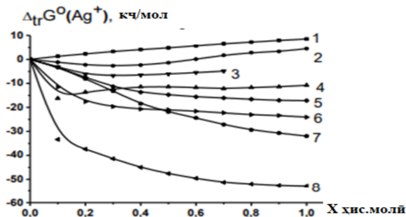
Расми 1.8. -Тағйирёбии энергияи Гиббси гузариши иони Ag^+ аз об ба ҳалкунандаҳои 1-обӣ-метанолӣ, 2-этанолӣ, 3-атсетонӣ, 4-пропиленгликолӣ, 5-диметилформамидӣ, 6-атсетонитрилӣ, 7-ДМСО-ӣ, 8-придинӣ
