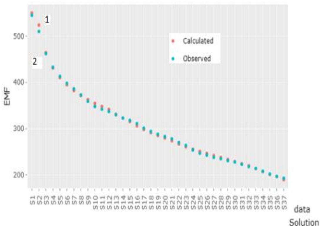
Расми 3.1. - Вобастагии потенциали системаи Ag^+/Ag^0 аз консентратсияи 2-меркаптоимидазол ҳангоми комплексҳосилшавии нукраи (I) бо ин лиганд 1- E_{таҷр.} ; 2- E_{назар.}
