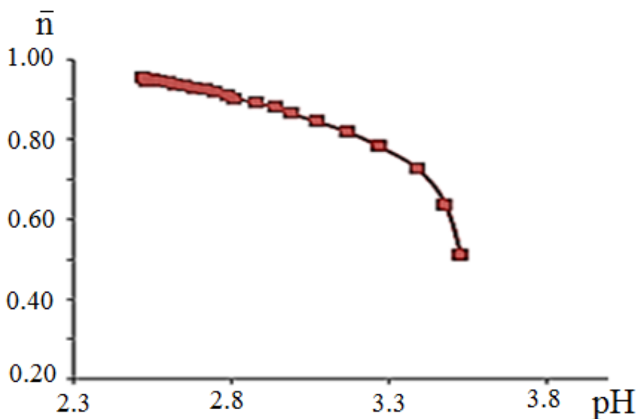
Расми 2.7. - Вобастагии функсияи Беррум аз pH барои маҳлули обии 1-метил-2-меркаптоимидазол дар 298,15К
