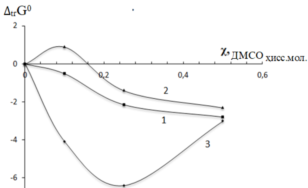
Расми 2.4. -Тағйирёбии энергияи Гиббси 1-метил-2-меркаптоимидазол (1), никатинамид (2), кварсетин (3) ҳангоми гузариш аз об ба ҳалкунандаи обӣ-ДМСО
