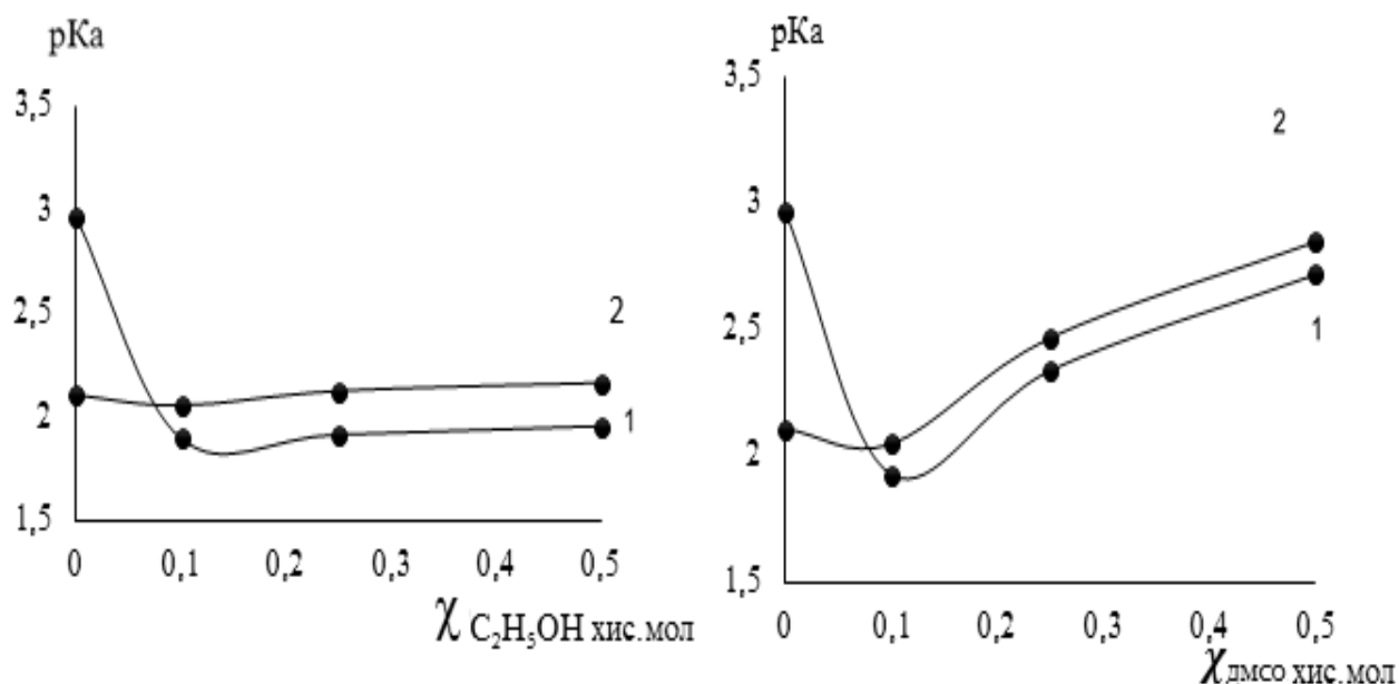
Расми 2.12. -Вобастагии pK_a = f(\chi_{\text{ҳалқунанда}}) : 2меркаптоимидазол (1), 1-метил-2-меркаптоимидазол (2)
