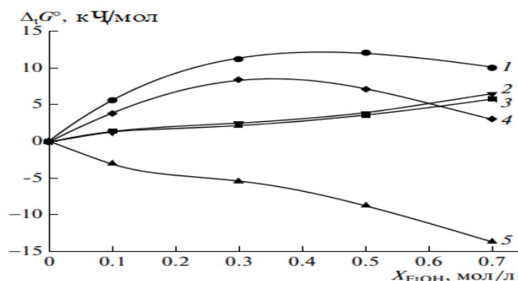
Расми 1.9. -Тағйирёбии энергияи Гиббси гузариш аз маҳлули обӣ ба ҳалқунандаи обӣ-этанолӣ. 1-Phe-, 2-Cu 2+ , 3-фенилаланин, 4-[CuPhe] + , 5-реаксияи комплексҳосилшавӣ
