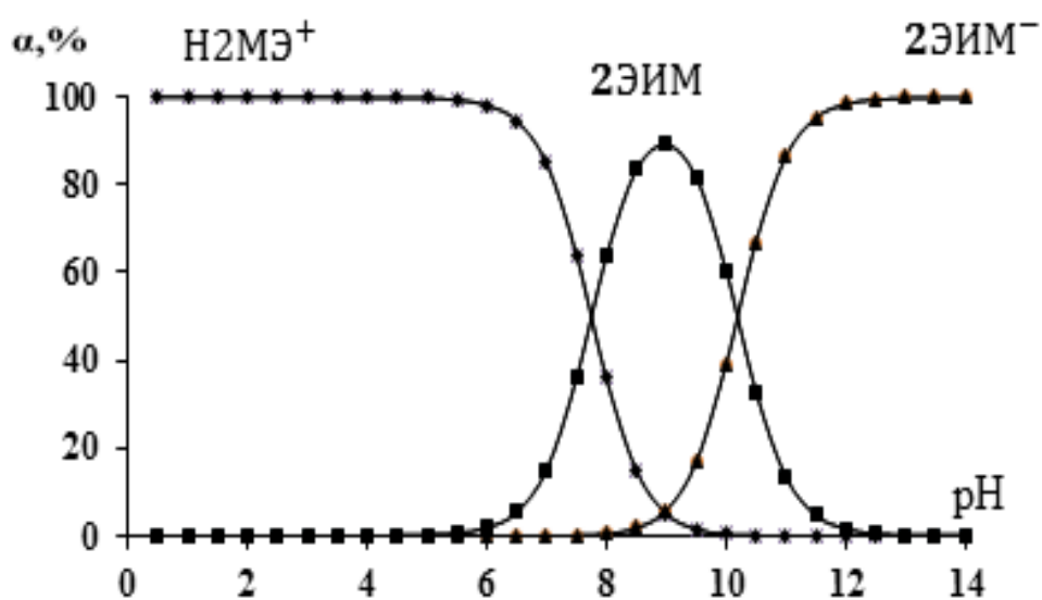
Расми 2.10. - Ҳиссаи тақсимшавии шаклҳои гуногуни 2ЭИМ (молекулавӣ, протонизатсияшуда ва депротонизатсияшуда) дар маҳлули обӣ. T=298,15\text{K}
