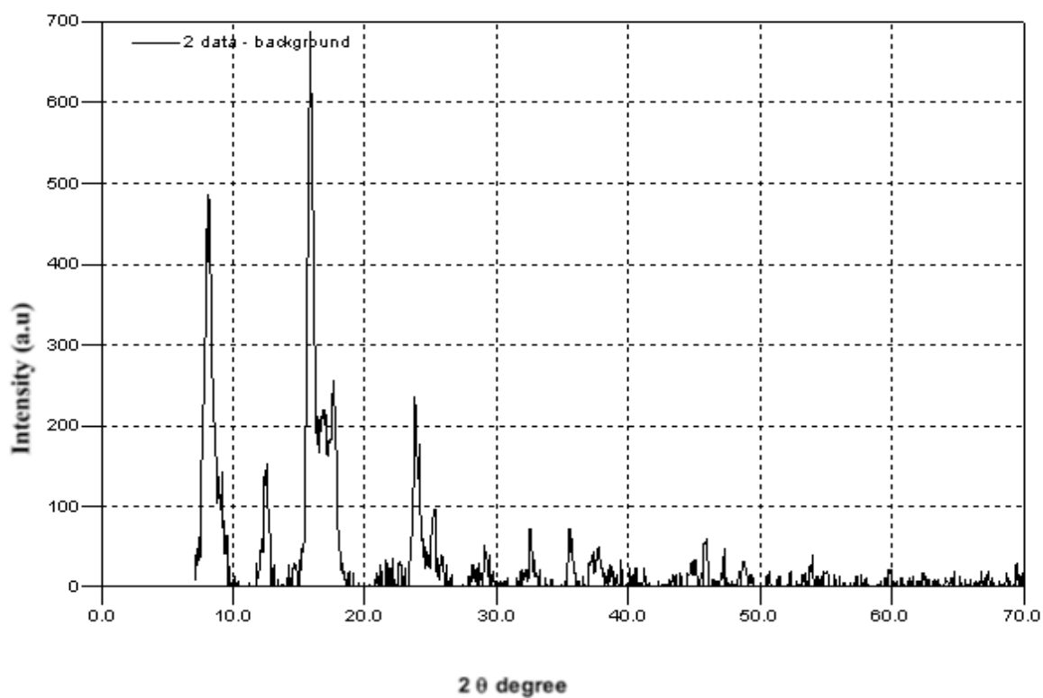
Рисунок 4.8. - Рентгенограмма комплекса [\text{Ag}(\text{2MBI})_2(\text{H}_2\text{O})\text{NO}_3]
