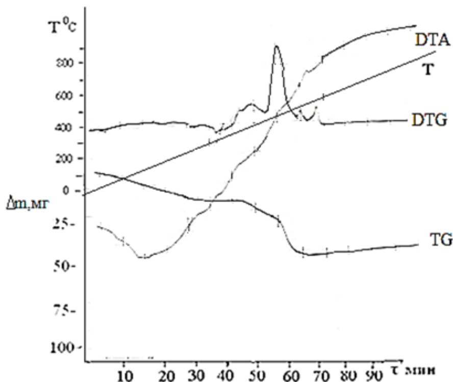
Рисунок 4.7. - Дериватограмма комплекса [\text{Ag}(\text{2MBI})(\text{H}_2\text{O})_2\text{NO}_3]
