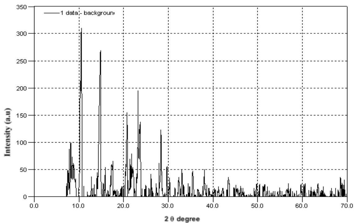
Рисунок 4.9. - Рентгенограмма комплекса [\text{Ag}(\text{2MBI})(\text{H}_2\text{O})_2\text{NO}_3]
