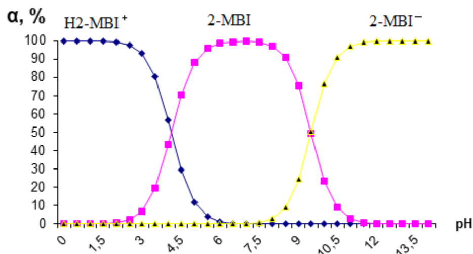
Рисунок 3.3. - Диаграмма распределения 2-МБИ в растворе, содержащий 10 об.% ДМФА.
