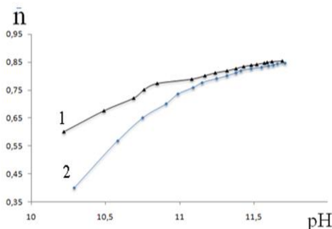
Рисунок 3.1. - Зависимость \bar{n} от рН при 1-10 и 2-25 об.% метанола при 298К.
