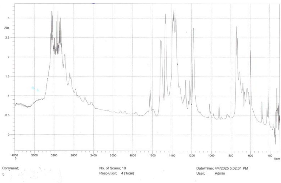
Рисунок 4.3. - ИК-спектр комплекса состава [\text{Ag}(\text{2MBI})_2(\text{H}_2\text{O})\text{NO}_3]
