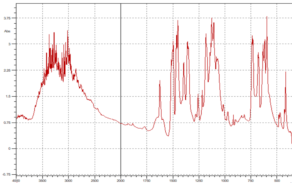
Рисунок 4.2. - ИК-спектр некоординированного 2-меркаптобензимидазола
