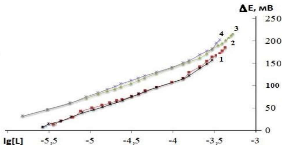
Рисунок 3.7. – Зависимость \Delta E от -\lg C_L для комплексов \text{Ag(I)} с 2-MBI при различных концентрациях этанола: 1 – 25%, 2 – 35%, 3 – 45%, 4 – 55% и температуре 298К. Ионная сила раствора составляла 0,1 моль/л
