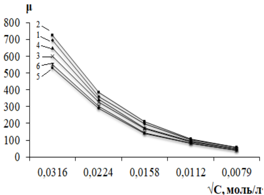
Рисунок 4.6. - Зависимость молярной электрической проводимости ( \mu ) от \sqrt{C} , где кривые относятся 1-[Ag(C 7 H 6 N 2 S)(H 2 O) 3 NO 3 ]; 2-[Ag (C 7 H 6 N 2 S) 2 (H 2 O) 2 NO 3 ]; 3-[Ag (C 7 H 6 N 2 S) 2 Cl]; 4-[Ag (C 7 H 6 N 2 S) 2 Br]; 5-[Ag(C 7 H 6 N 2 S) 2 (H 2 O) 2 SO 4 и 6-[Ag (C 7 H 6 N 2 S) 2 (H 2 O) SCN]
