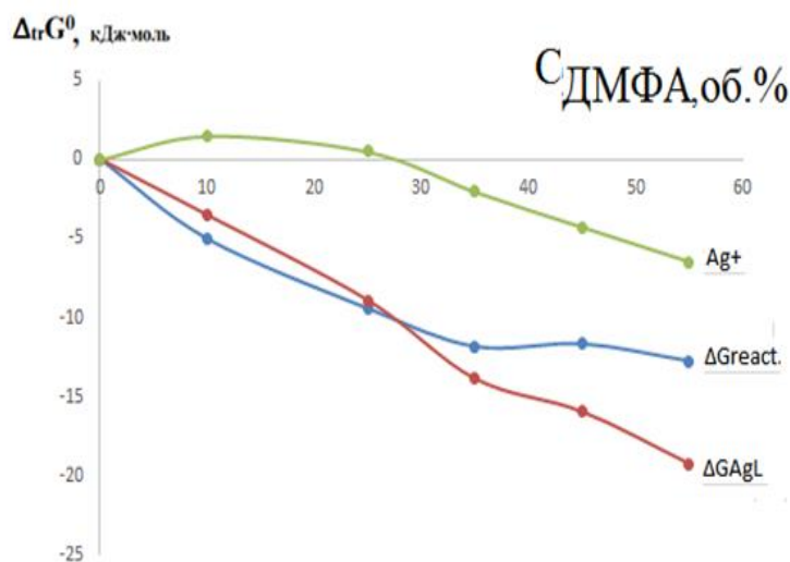
Рисунок 3.11. – Изменение энергии Гиббса образования комплексов серебра с 2-меркаптобензимидазолом в растворе вода-ДМФА
