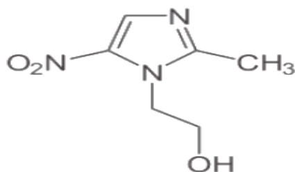
Схема 1.3. - 2-метил-5-нитро-1Н-имидазол-1-этанол
