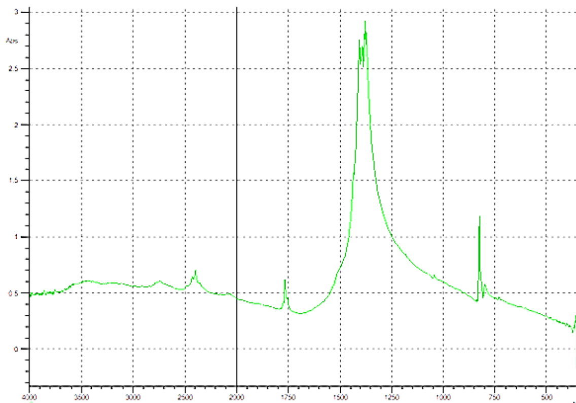
Рисунок 4.1. - ИК-спектр AgNO 3
