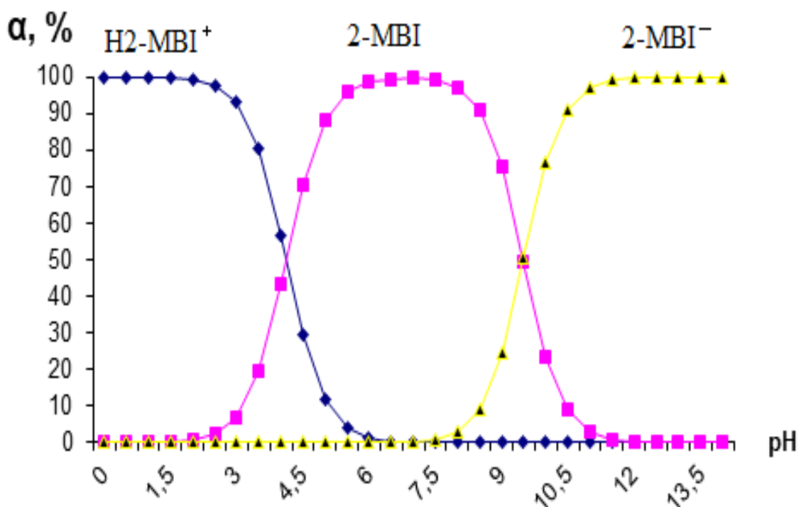
Рисунок 3.2. - Диаграмма распределения 2-MBI в растворе, содержащий 10об.% этанола.
