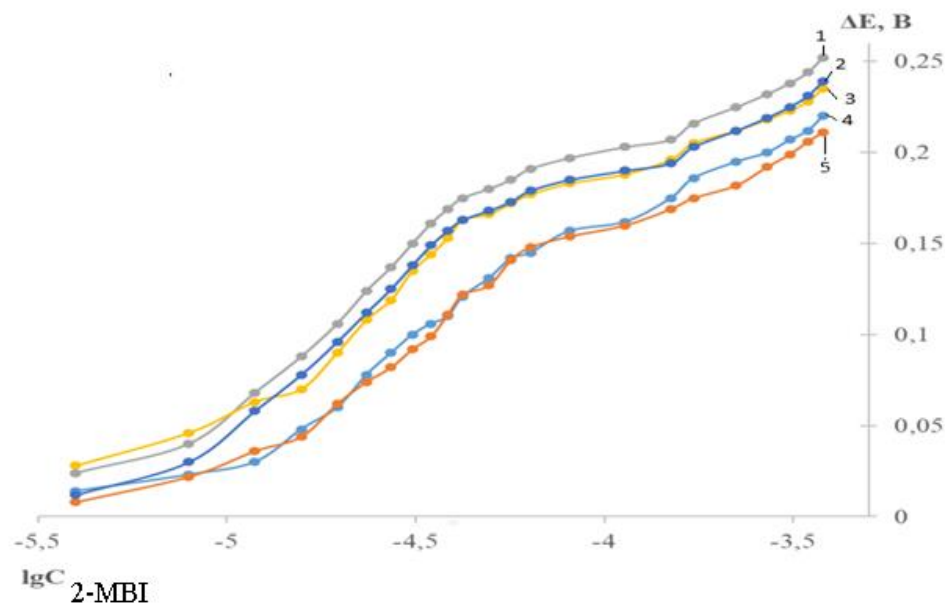
Рисунок. 3.8. – Зависимость \Delta E, В от -lgC_L для комплексов Ag(I) с 2-МБИ при различных концентрациях ДМФА: 1 – 55%, 2 – 45%, 3 – 35%, 4 – 25% и 5 – 10% температуре 298К. Ионная сила раствора составляла 0,1 моль/л.
