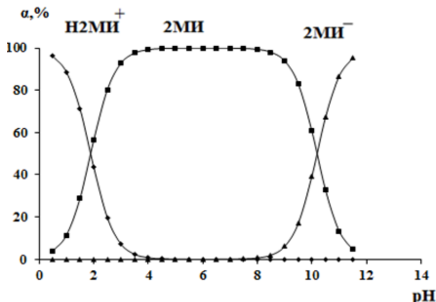
Рисунок. 1.2. - Распределительные диаграммы доминирования протонированных, молекулярных и депротонированных форм 2-меркаптоимидазола
