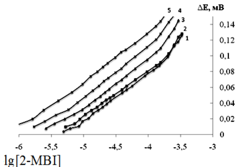
Рисунок 3.5. - Зависимость \Delta E от -\lg[2\text{-MBI}] для процесса комплексообразования \text{Ag(I)} с 2-MBI при: 1-298, 2-288, 3-298, 4-308 и 5-318K
