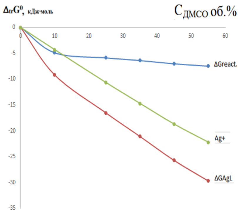
Рисунок 3.12. Изменение энергии Гиббса образования комплексов серебра с 2-меркаптобензимидазолом в растворе вода-ДМСО
