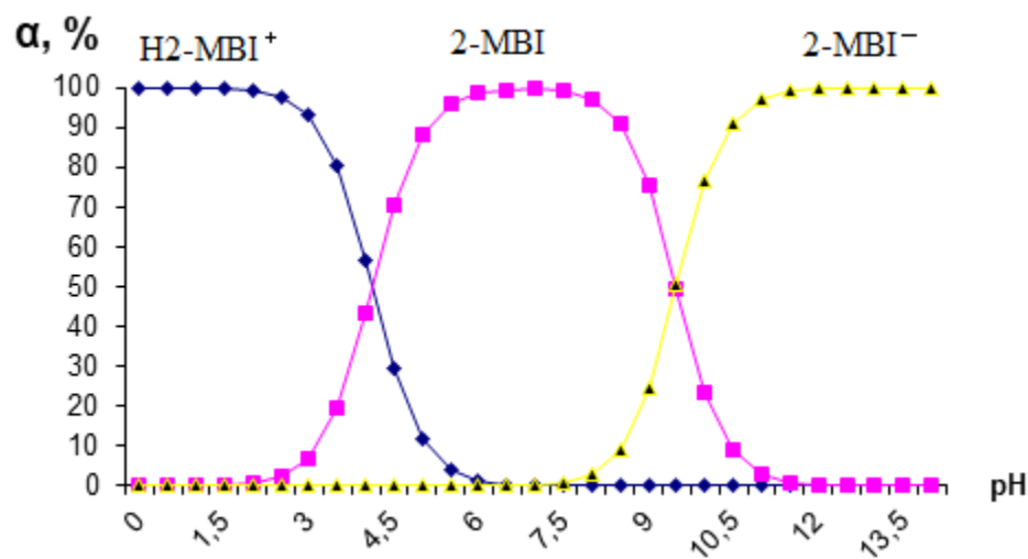
Рисунок 3.4. - Диаграмма распределения 2-МБИ в растворе, содержащий 10 об.% ДМСО.
