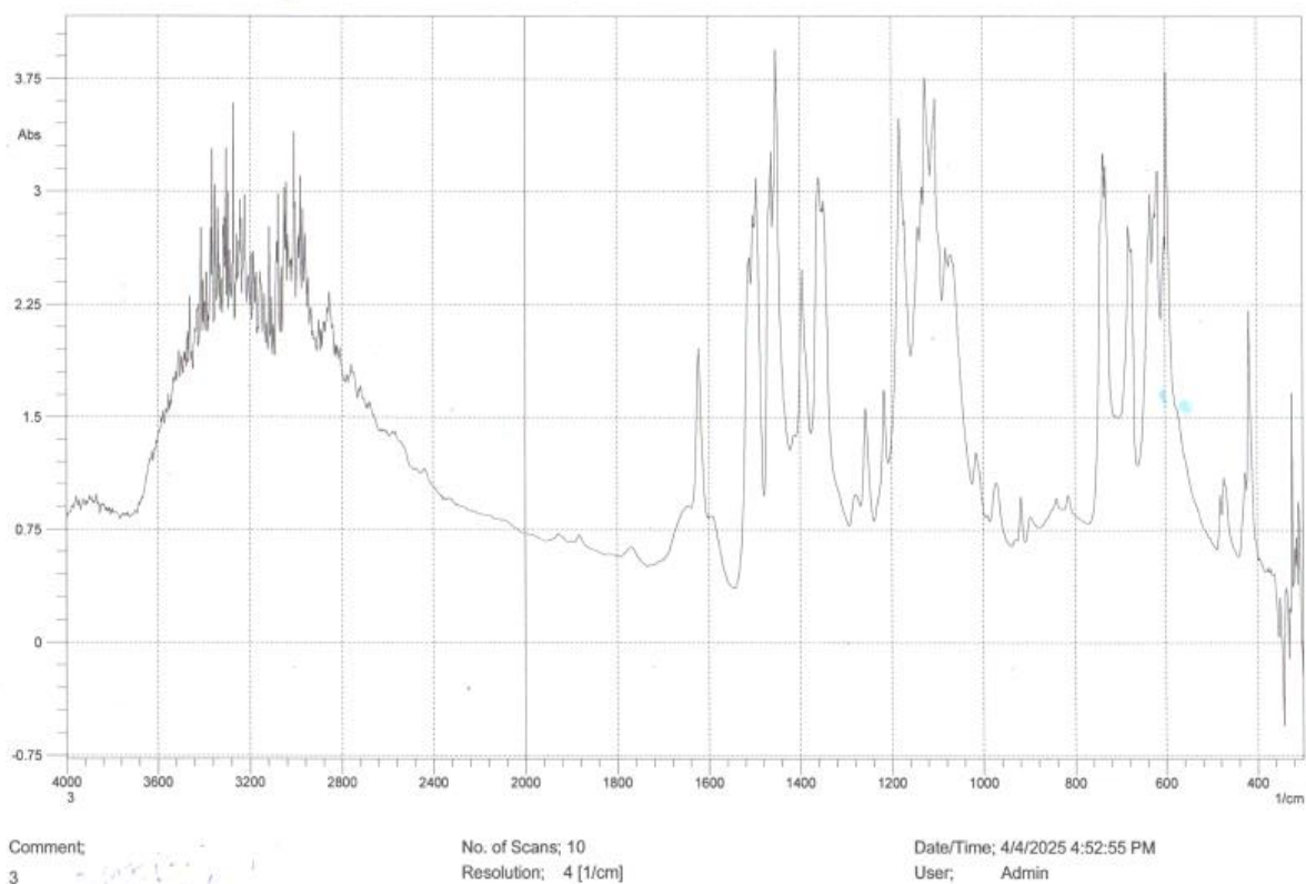
Рисунок 4.4. - ИК-спектр комплекса состава [Ag(2MBI)_2(H_2O)_2]_2SO_4
