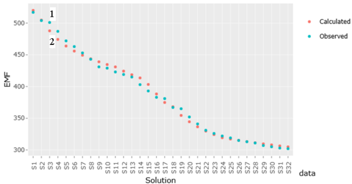
Рисунок 3.9. – Изменение потенциал системы \text{Ag}^+/\text{Ag}^0 для образования комплексных форм (I) с 2-меркаптобензимидазолом: 1-Obs.-экспериментальный и 2-Calc-теоретический.
