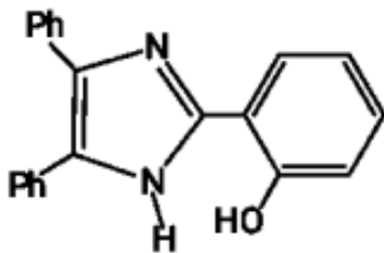
Схема 1.4. - 2-(2-гирофенил)-4,5-дифенил-1Н-имидазол
