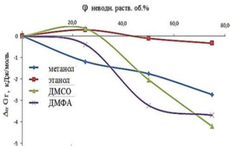
Рисунок 1.1. - Влияние концентрации неводных растворителей на величину энергии Гиббса ( \Delta G_r , kJ/mol)
