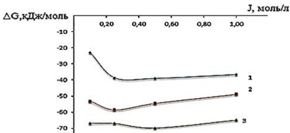
Рисунок 1.3. - Зависимость свободной энергии Гиббса от изменения состава ионной силы.
