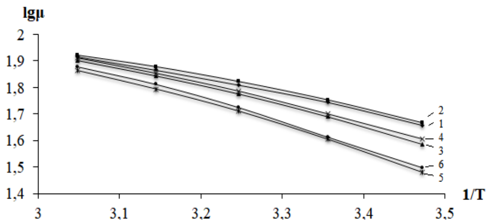
Рисунок 4.5. - Температурные зависимости молярной электропроводности \lg \mu от 1/T , 1-[ \text{Ag}(\text{C}_7\text{H}_6\text{N}_2\text{S})(\text{H}_2\text{O})_3 \text{NO}_3 ]; 2-[ \text{Ag}(\text{C}_7\text{H}_6\text{N}_2\text{S})_2(\text{H}_2\text{O})_2\text{NO}_3 ]; 3-[ \text{Ag}(\text{C}_7\text{H}_6\text{N}_2\text{S})_2\text{Cl} ]; 4-[ \text{Ag}(\text{C}_7\text{H}_6\text{N}_2\text{S})_2\text{Br} ]; 5-[ \text{Ag}(\text{C}_7\text{H}_6\text{N}_2\text{S})_2(\text{H}_2\text{O})_2\text{SO}_4 ] и 6-[ \text{Ag}(\text{C}_7\text{H}_6\text{N}_2\text{S})_2(\text{H}_2\text{O})\text{SCN} ]
