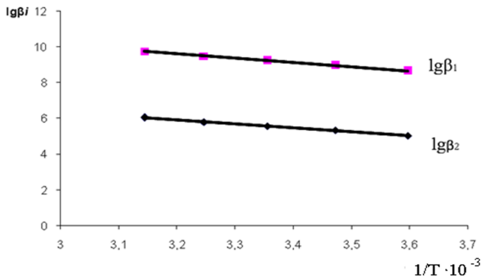
Рисунок 3.6. – Температурная зависимость общей констант устойчивости для 2-меркаптобензимидазольных комплексов Ag(I)
