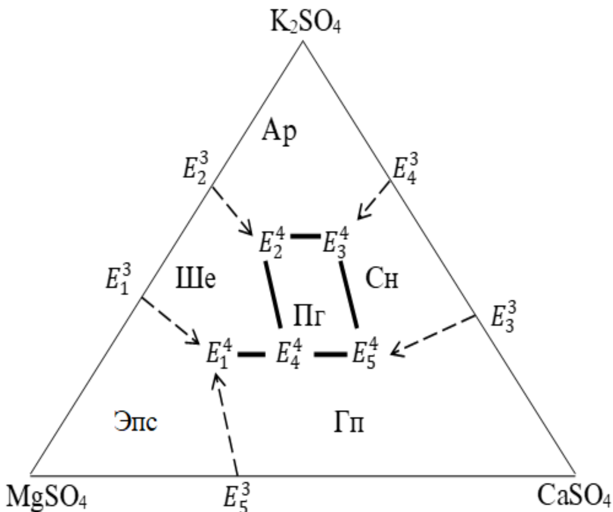
Расми 3.2. – Диаграммаи мувозинатҳои фазагии системаи \text{K}_2\text{SO}_4\text{-MgSO}_4\text{-CaSO}_4\text{-H}_2\text{O} дар ҳарорати 25 °C дар сатҳи чоркомпонентагӣ
