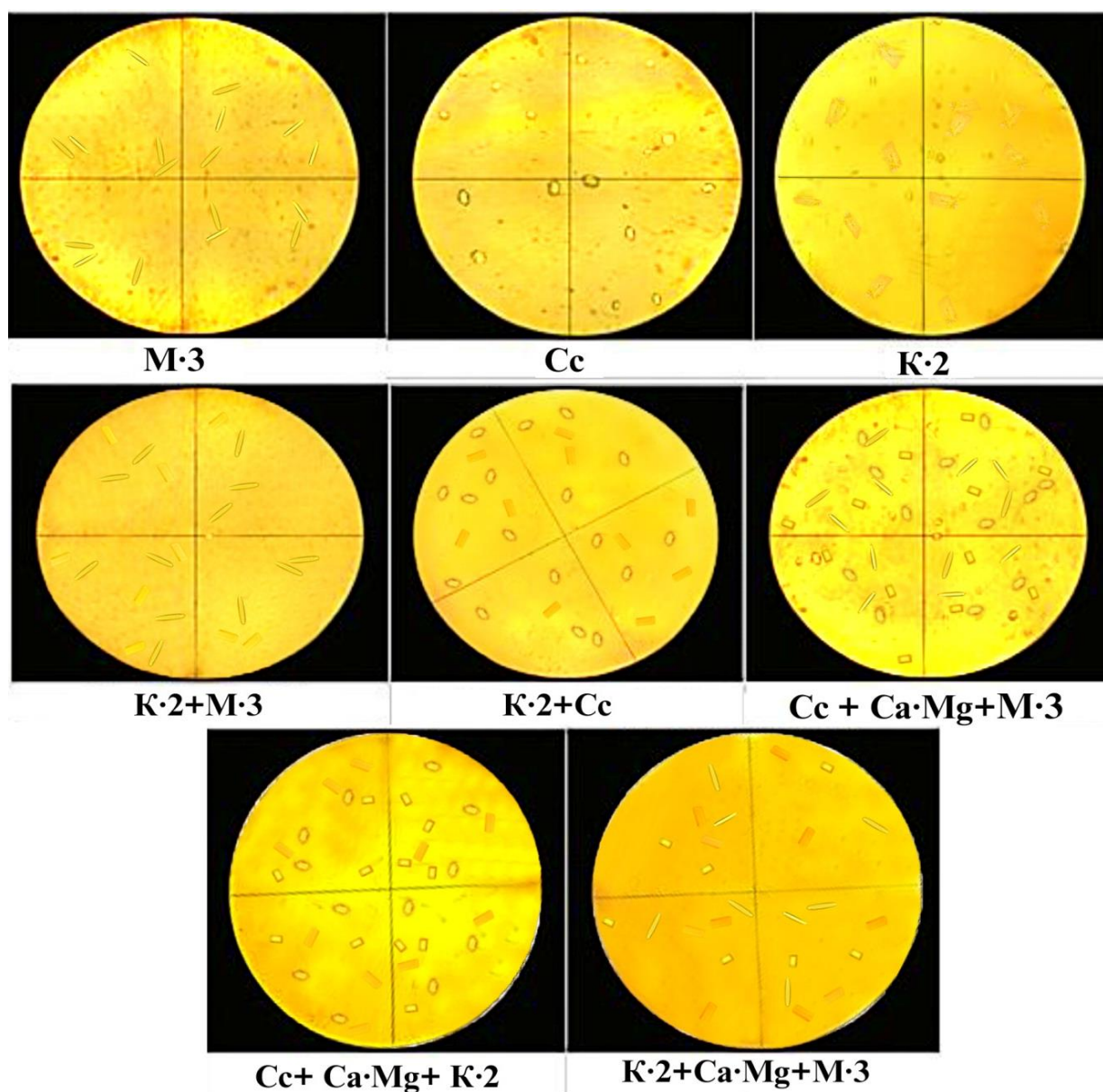
Расми 2.18. – Микроакси фазаҳои саҳти мувозинатии системаи K,Mg,Ca//CO 3 -H 2 O, барои ҳарорати 0°C
