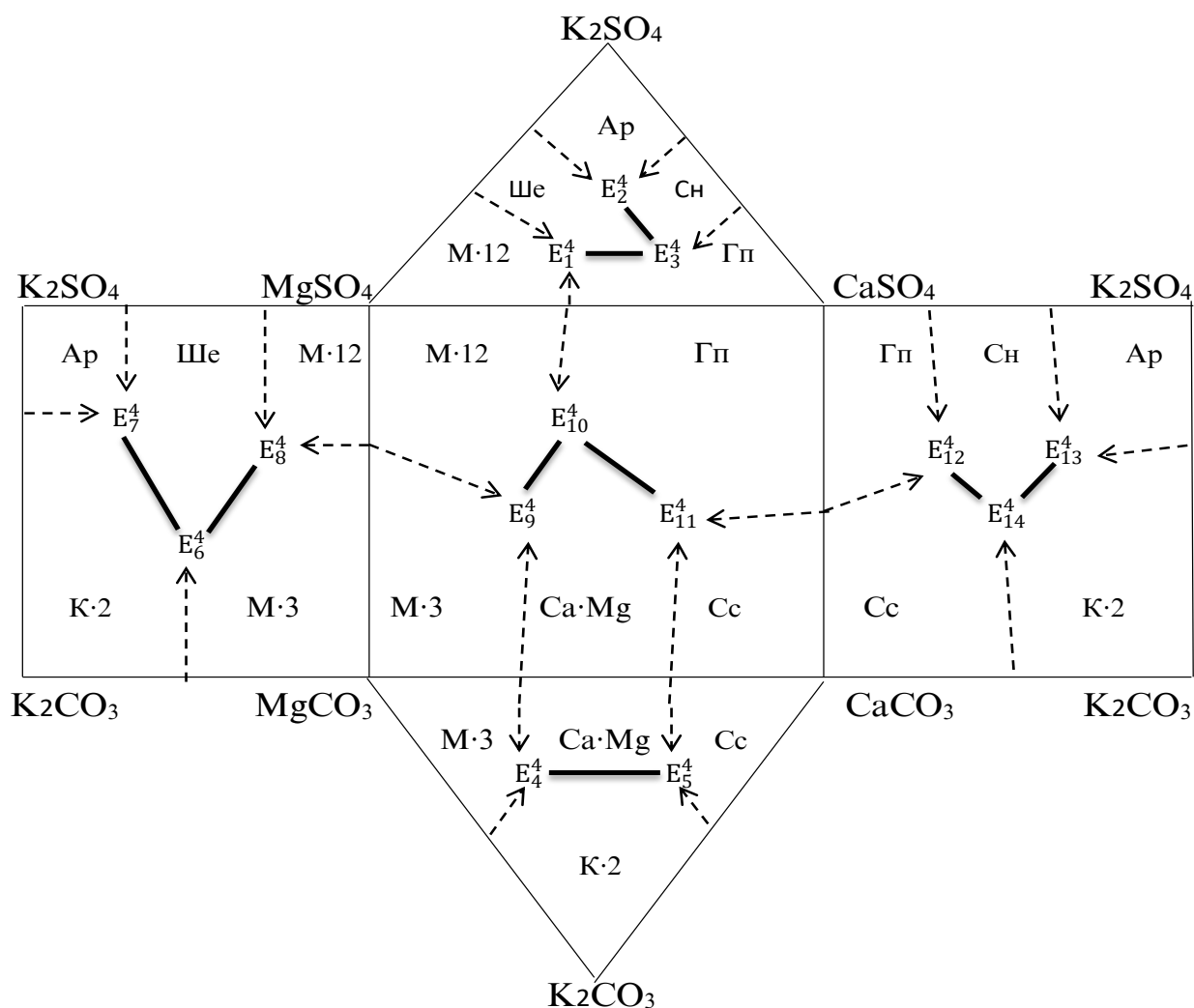
Расми 2.11. – Диаграмаи мувозинатҳои фазагии системаи K, Mg, Ca / SO_4, CO_3 - H_2O барои ҳарорати 0^\circ C , дар сатҳи чоркомпонентагӣ
