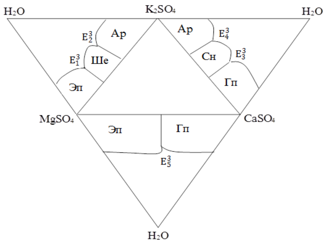
Расми 3.1. – Диаграммаи мувозинатҳои фазагии системаи K_2SO_4-MgSO_4-CaSO_4-H_2O барои ҳарорати 25 °C дар сатҳи секомпонентагӣ
