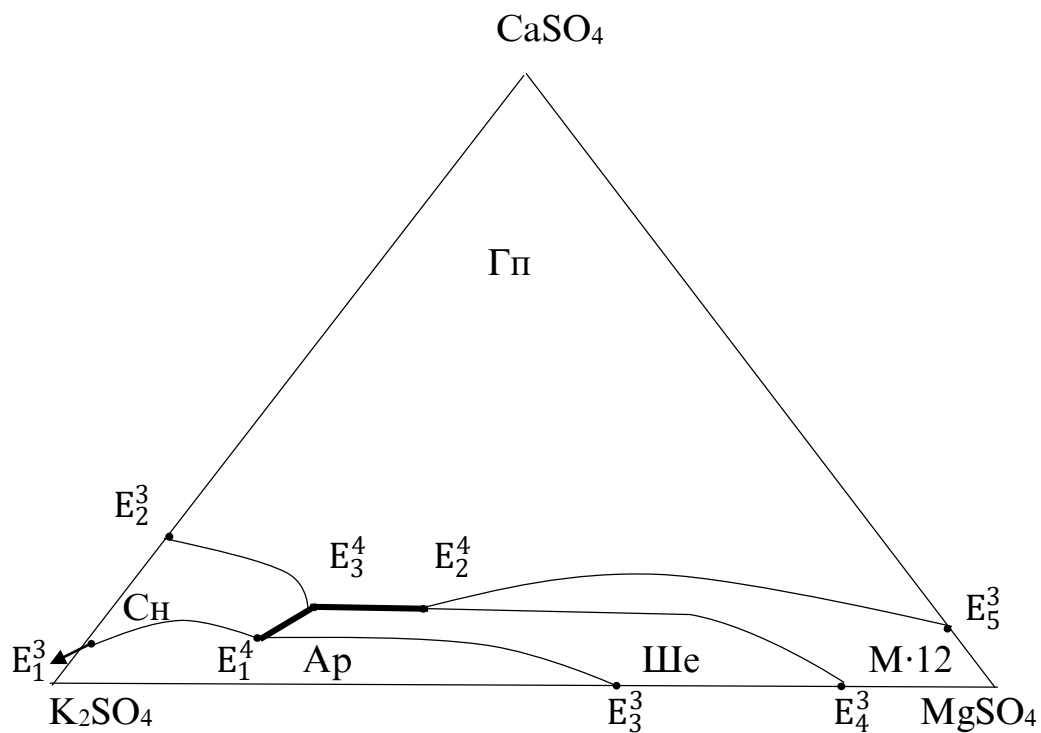
Расми 2.17. – Қисми намакии диаграммаи ҳалшавандагии системаи К,Мg,Са//SO 4 -Н 2 О барои ҳарорати 0 °С
