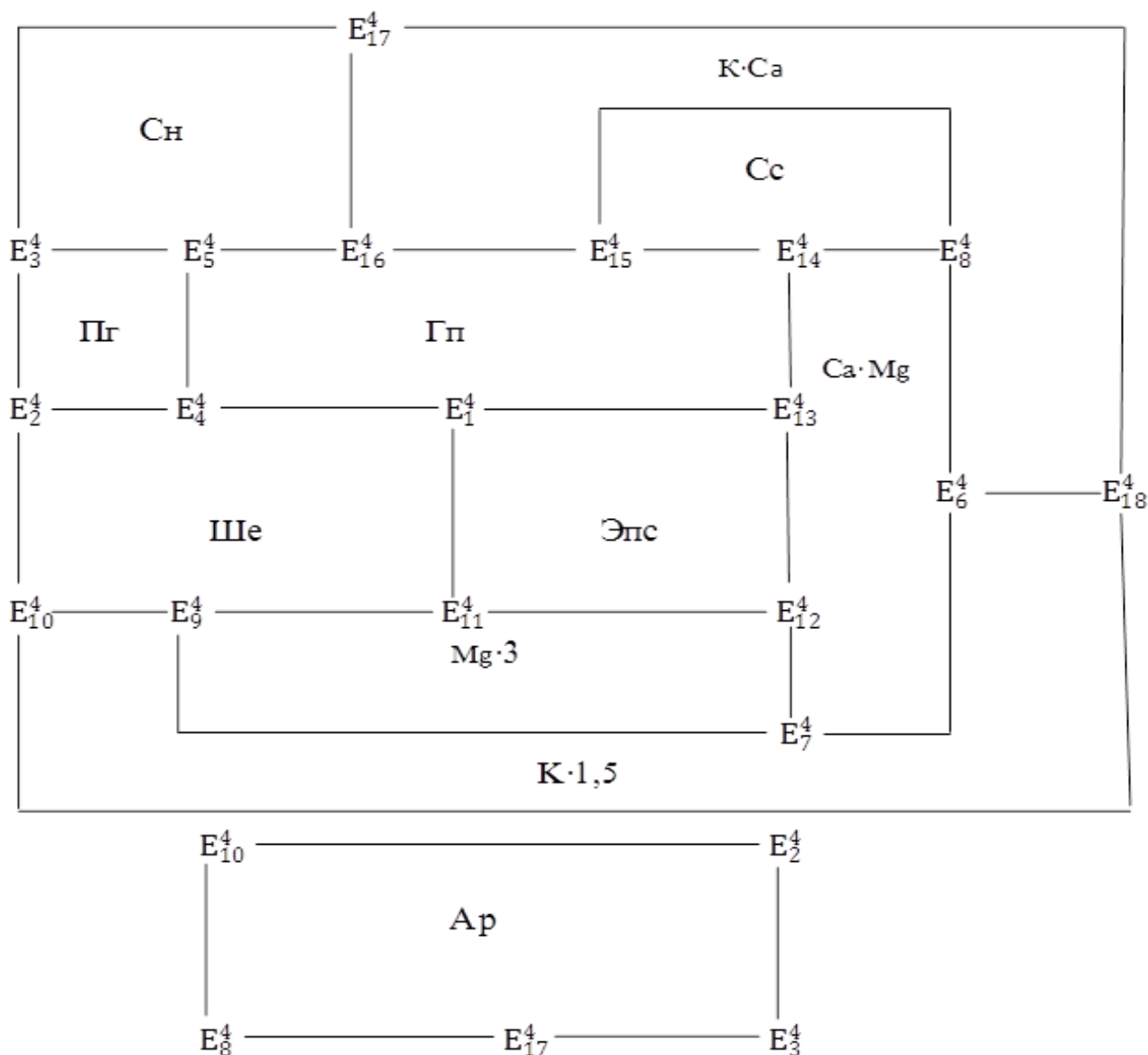
Расми 3.12. – Диаграммаи мувозинатҳои фазагии системаи K, Mg, Ca//SO_4, CO_3-H_2O дар сатҳи чоркомпонентагӣ барои ҳарорати 25^\circ C
