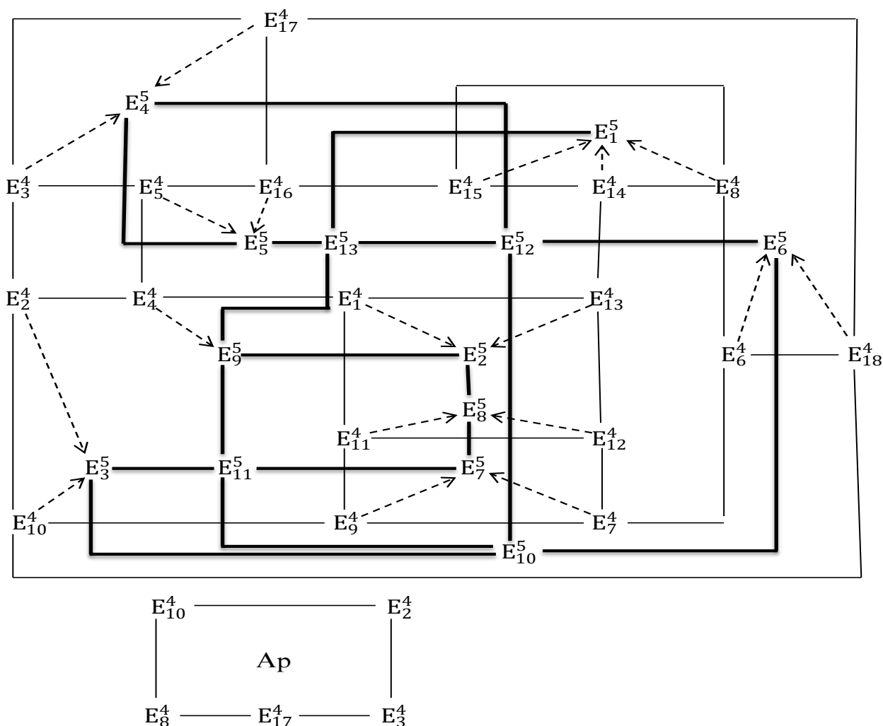
Расми 3.13. – Диаграмма мувозинатҳои фазагии системаи K, Mg, Ca//SO_4, CO_3-H_2O барои ҳарорати 25\text{ }^\circ\text{C} , ки бо усули транслятсия сохта шудааст
