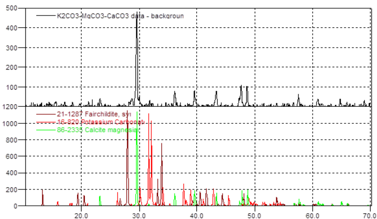
Расми 3.16. – Дифрактограммаи фазаҳои сахти дар мувозинатбудаи системаи K,Mg,Ca//CO 3 -H 2 O барои ҳарорати 25 °C
