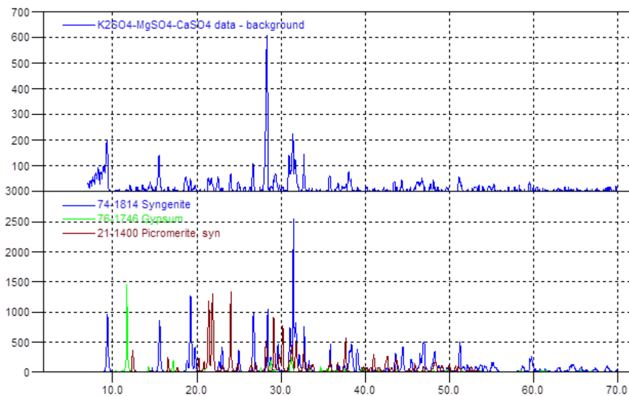
Расми 2.15. – Дифратограммаи фазаҳои саҳти дармувозинатбудаи системаи K, Mg, Ca//SO_4-H_2O барои ҳарорати 0\text{ }^{\circ}C
