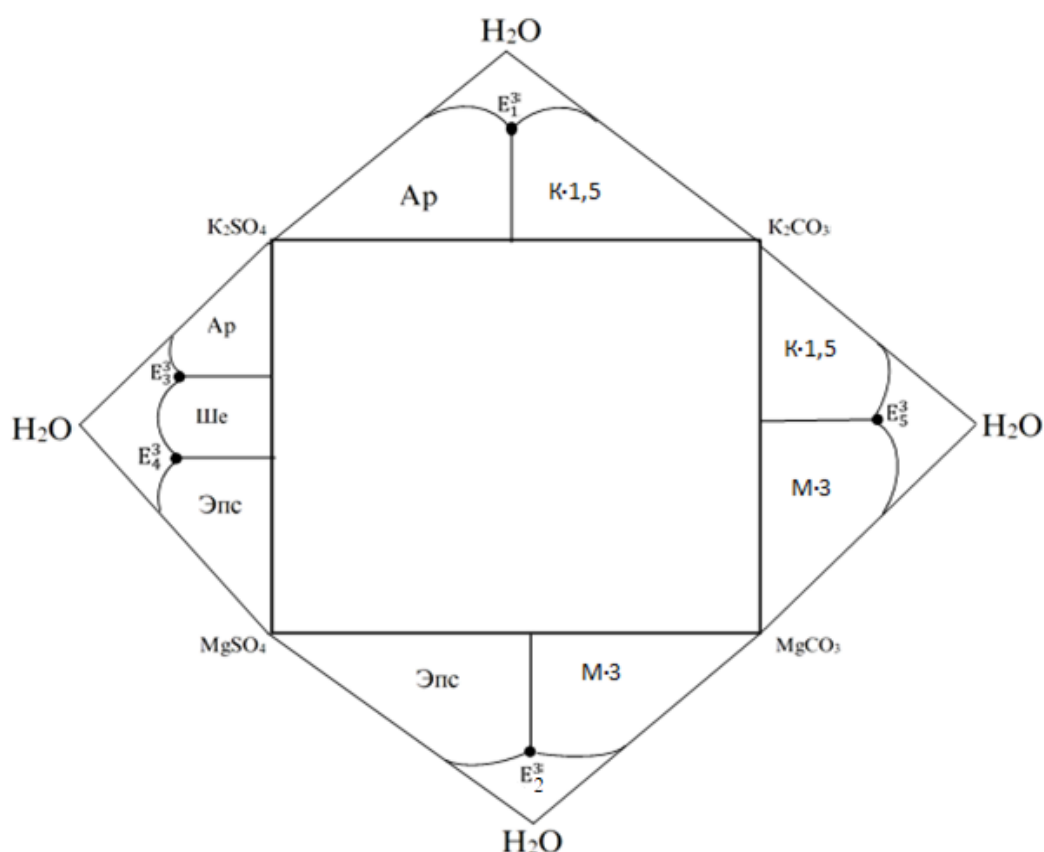
Расми 3.5. – Диаграмма мувозинатҳои фазагии системаи К,Мg//SO 4 ,CO 3 -H 2 O барои ҳарорати 25 °C дар сатҳи секомпонентагӣ
