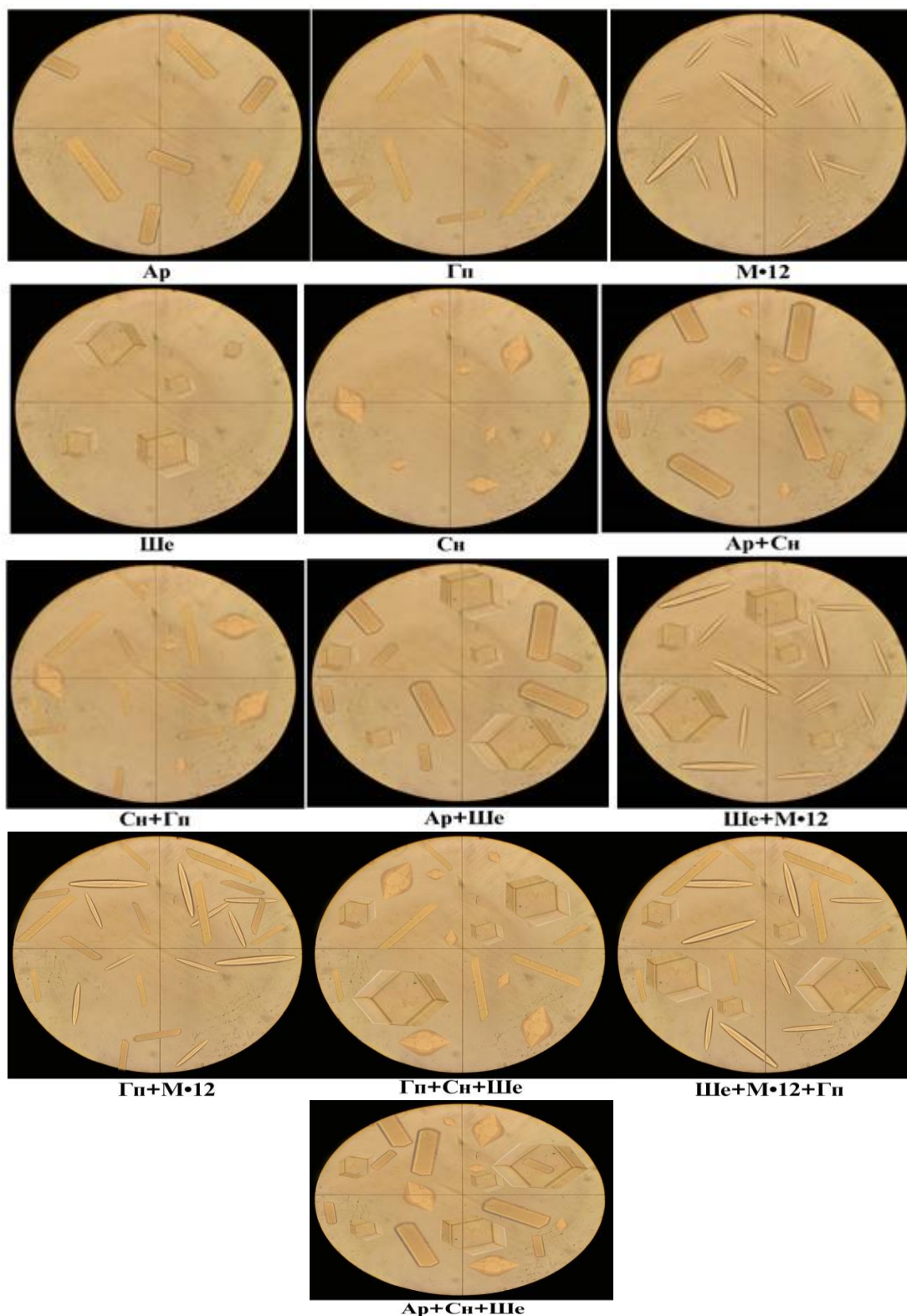
Расми 2.14. – Микроакси фазаҳои саҳти мувозинатии системаи K, Mg, Ca//SO_4-H_2O , барои ҳарорати 0\text{ }^{\circ}C
