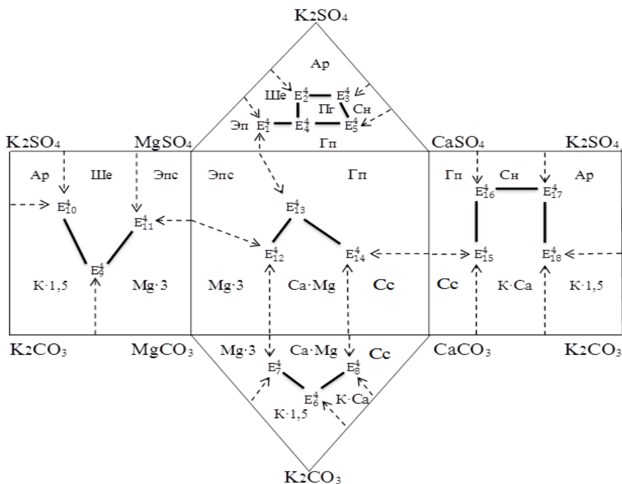
Расми 3.11. – Сохтори геометрии изотермаи 25°C – и системаи K, Mg, Ca//SO_4, CO_3-H_2O дар сатҳи чоркомпонентагӣ
