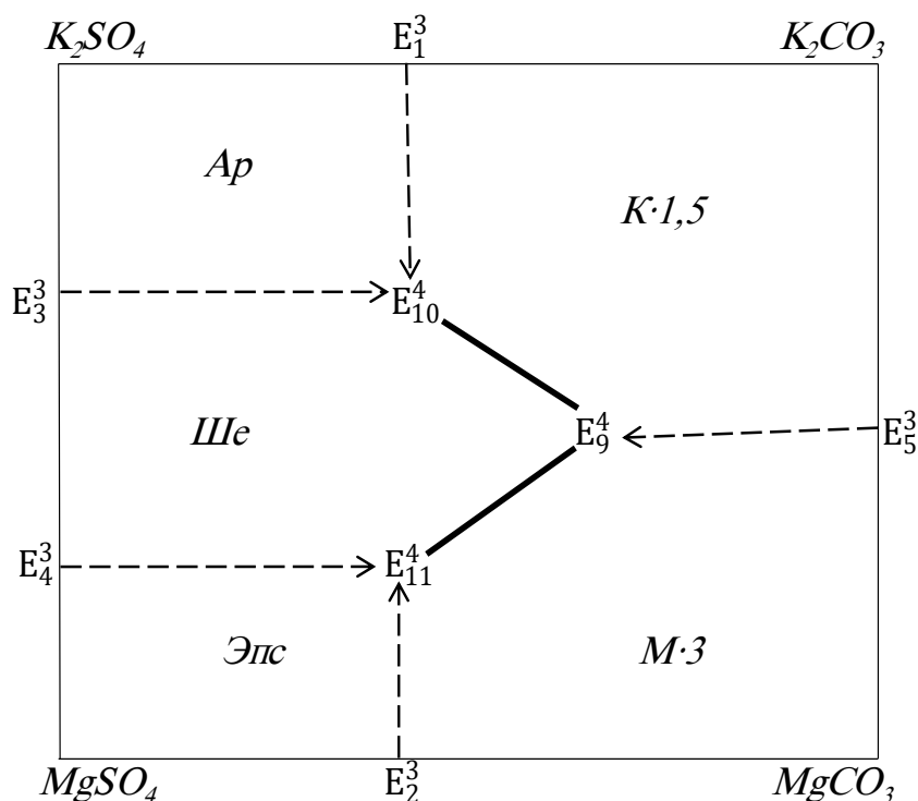
Расми 3.6. – Диаграммаи схемагии мувозинатҳои фазагии системаи K, Mg//SO_4, CO_3-H_2O дар ҳарорати 25\text{ }^{\circ}C дар сатҳи чоркомпонентагӣ
