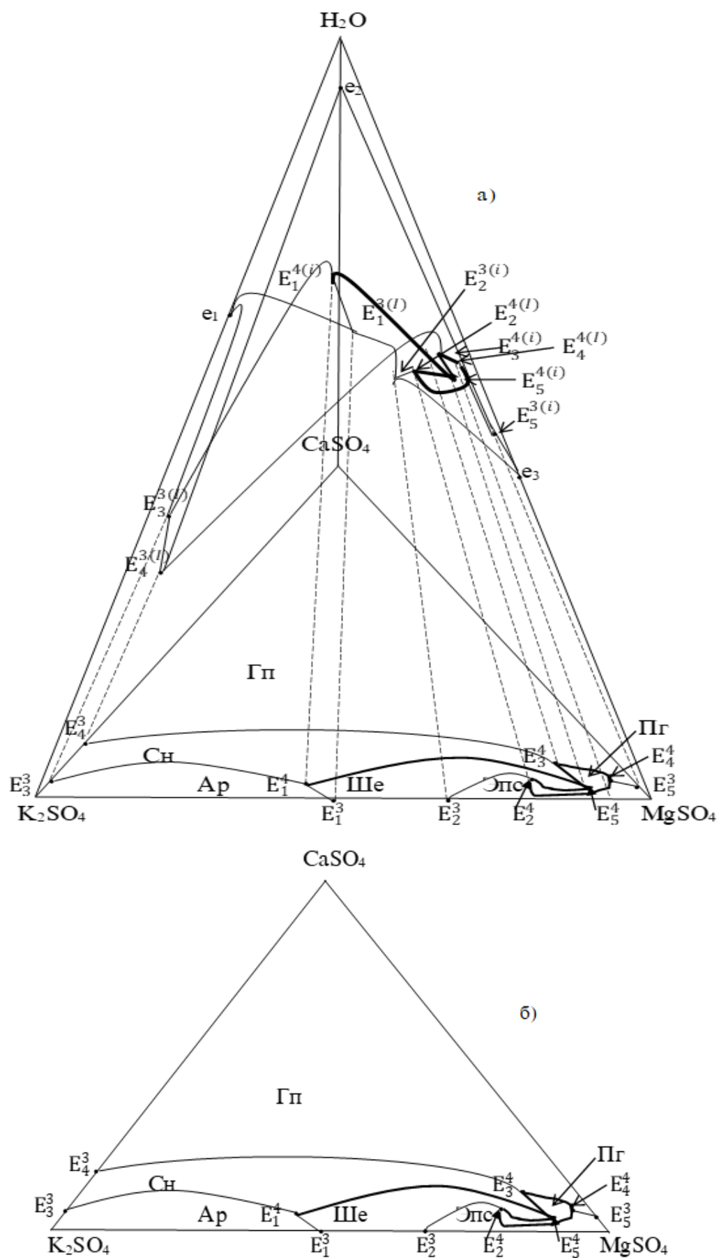
Расми 3.14. – Диаграммаи ҳалшавандагии системаи K, Mg, Ca//SO_4-H_2O барои ҳарорати 25\text{ }^{\circ}C ) а) қисми обӣ -намакӣ б) қисми намакӣ
