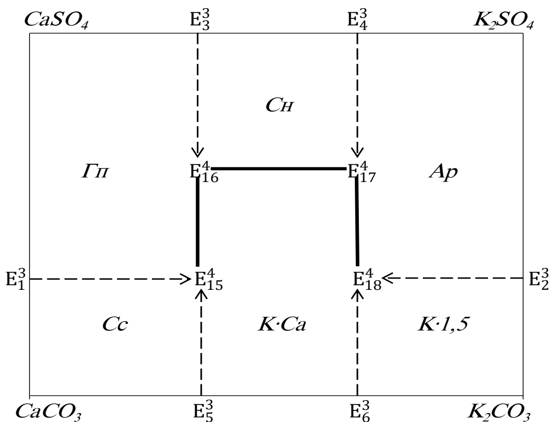
Расми 3.10. – Диаграммаи мувозинатҳои фазагии системаи K, Ca//SO_4, CO_3-H_2O барои ҳарорати 25^\circ C , ки бо усули транслятсия сохта шудааст
