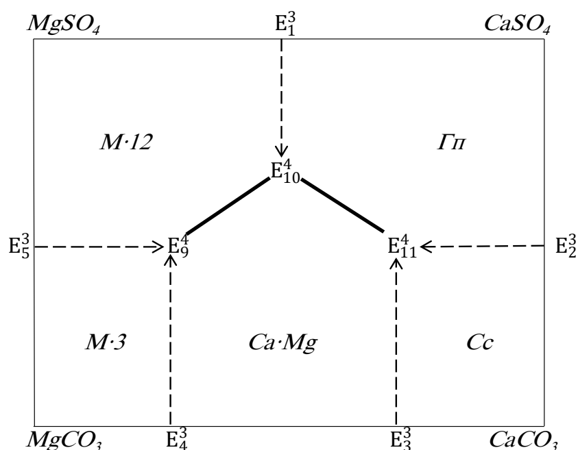
Расми 2.8. – Диаграммаи мувозинатҳои фазагии системаи Ca, Mg//SO_4, CO_3-H_2O дар ҳарорати 0^\circ C дар сатҳи чоркомпонентагӣ
