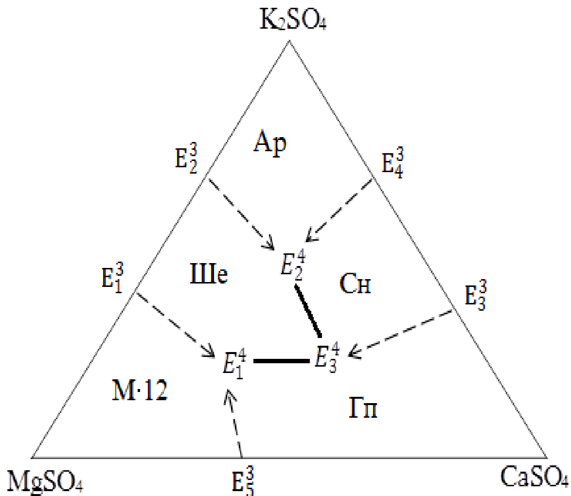
Расми 2.2. – Диаграммаи мувозинатҳои фазагии системаи \text{K, Mg, Ca//SO}_4 - \text{H}_2\text{O} дар ҳарорати 0\text{ }^\circ\text{C} , дар сатҳи чоркомпонентагӣ
