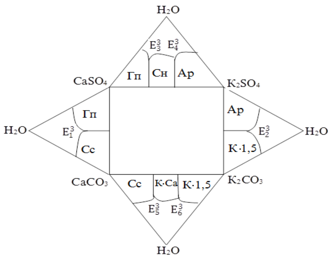
Расми 3.9. – Диаграммаи мувозинатҳои фазагии системаи K, Ca//SO_4, CO_3-H_2O барои ҳарорати 25 °C дар сатҳи секомпонентагӣ
