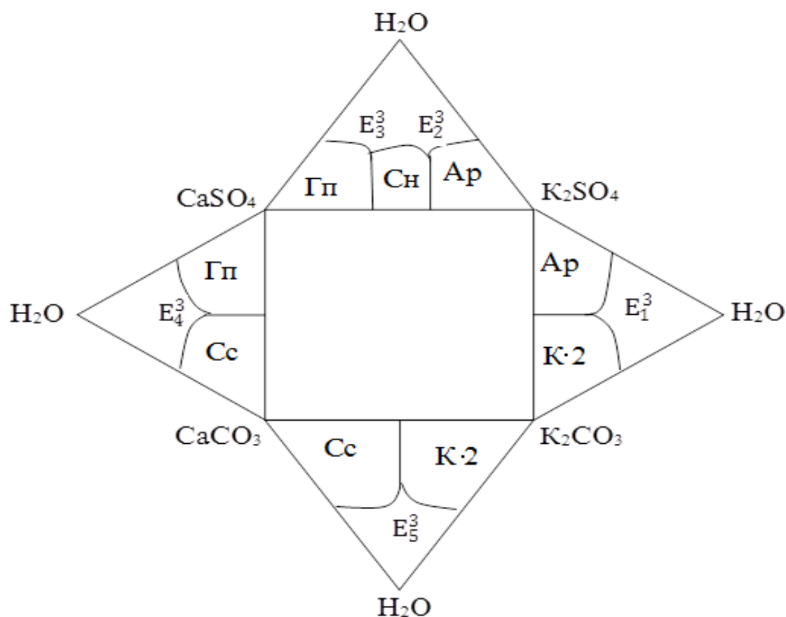
Расми 2.9. – Диаграммаи мувозинатҳои фазагии системаи K, Ca//SO_4, CO_3-H_2O барои ҳарорати 0\text{ }^{\circ}C дар сатҳи секомпонентагӣ
