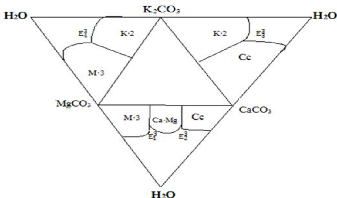
Расми 2.3. – Диаграммаи мувозинатҳои фазагии системаи K,Mg,Ca//CO 3 -H 2 O барои ҳарорати 0 °C, дар сатҳи секомпонентагӣ
