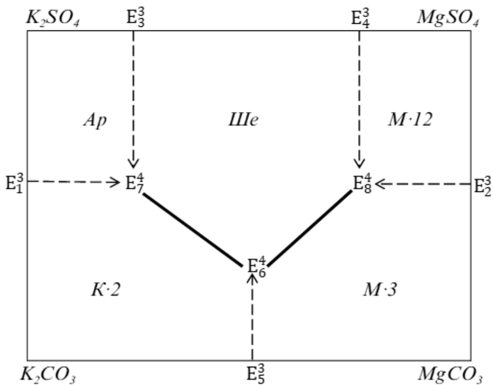
Расми 2.6. – Диаграмма мувозинатҳои фазагии системаи K, Mg//SO_4, CO_3-H_2O дар ҳарорати 0\text{ }^{\circ}C , дар сатҳи чоркомпонентагӣ
