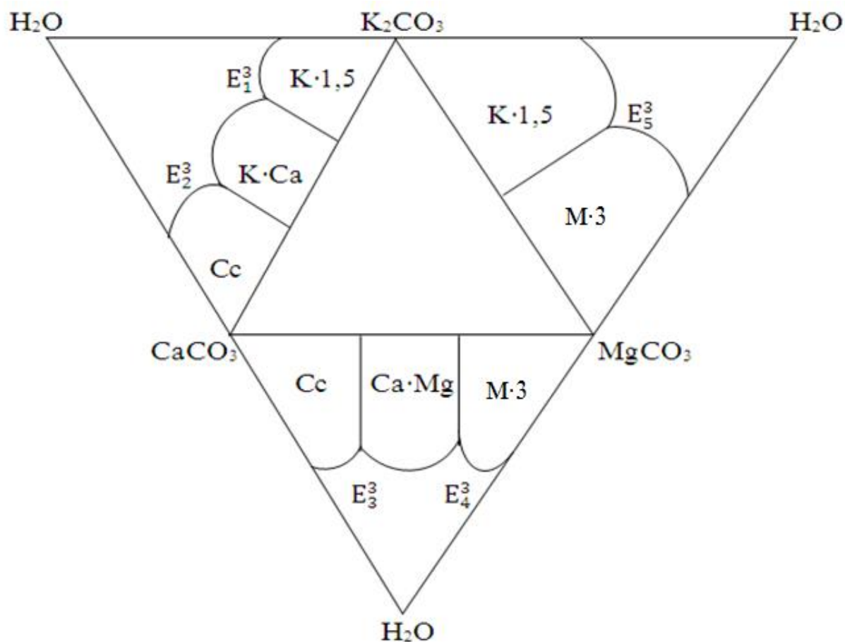
Расми 3.3. – Диаграмма мувозинатҳои фазагии системаи К,Мg,Са//СО 3 -Н 2 О барои ҳарорати 25 °С дар сатҳи секомпонентагӣ
