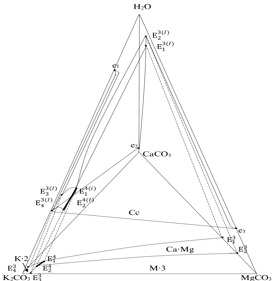
Расми 2.19. – Қисми обӣ-намакии диаграммаи ҳалшавандагии системаи \text{K,Mg,Ca//CO}_3\text{-H}_2\text{O} барои ҳарорати 0^\circ\text{C}
