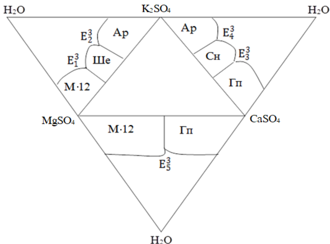
Расми 2.1. – Диаграмма мувозинатҳои фазагии системаи K, Mg, Ca//SO_4H_2O ба шакли пирамида барои ҳарорати 0\text{ }^{\circ}C , дар сатҳи секомпонентагӣ
