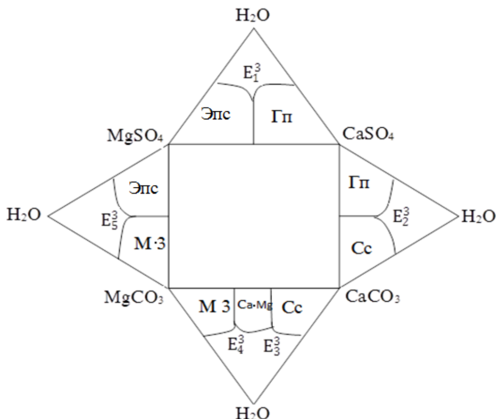
Расми 3.7. – Диаграмма мувозинатҳои фазагии системаи Ca,Mg//SO 4 ,CO 3 -H 2 O барои ҳарорати 25 °C дар сатҳи секомпонентагӣ
