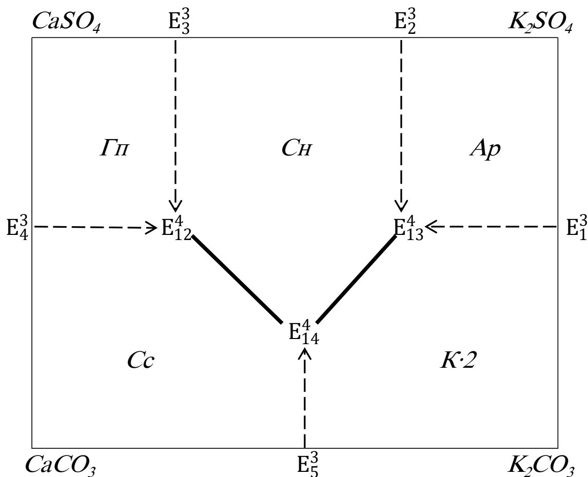
Расми 2.10. – Диаграммаи мувозинатҳои фазавии системаи K, Ca//SO_4, CO_3-H_2O барои ҳарорати 0^\circ C , дар сатҳи чоркомпонентагӣ
