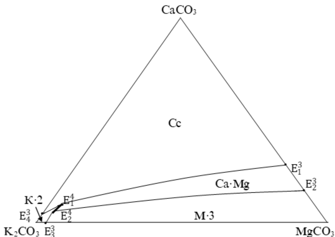
Расми 2.20. – Қисми намакии диаграммаи ҳалшавандагии системаи K, Mg, Ca/CO_3-H_2O барои ҳарорати 0\text{ }^{\circ}C
