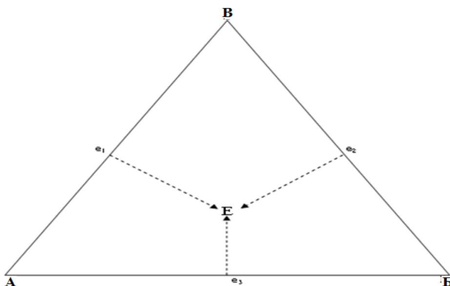
Расми 1.1. – Қисми намакии диаграммаи мувозинатҳои фазагии системаи A - B - V , дар вақти дар байни компонентҳо мавҷуд набудани баҳамтаъсиркунии химиявӣ
