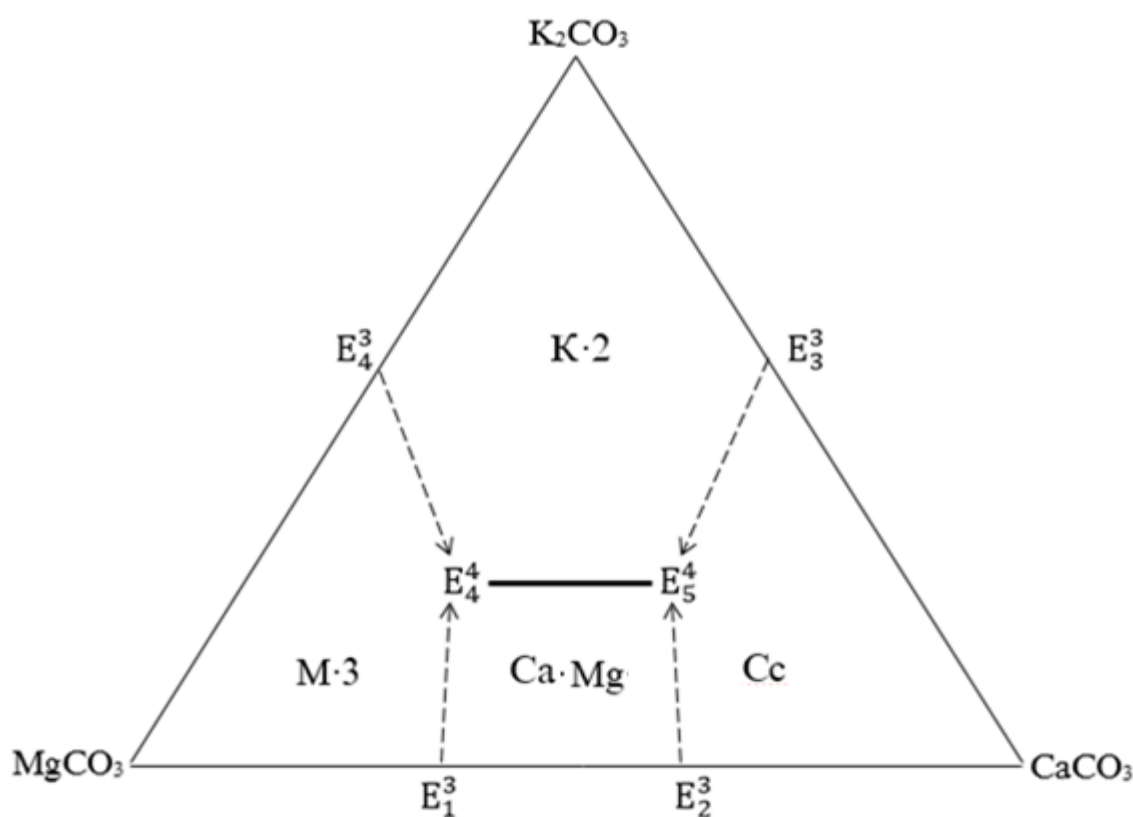
Расми 2.4. – Диаграммаи мувозинатҳои фазагии системаи K,Mg,Ca//CO 3 -H 2 O дар ҳарорати 0 °C
