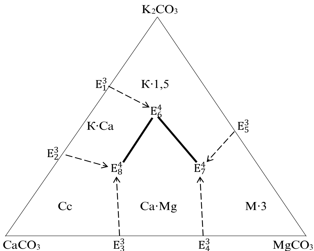
Расми 3.4. – Диаграммаи мувозинатҳои фазагии системаи К,Мg,Са//CO 3 -Н 2 О дар ҳарорати 25 °С дар сатҳи чоркомпонентагӣ
