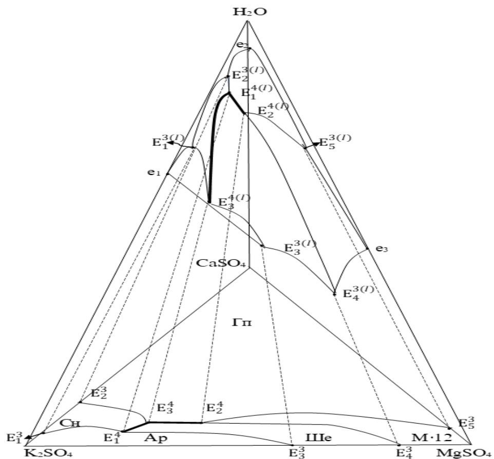
Расми 2.16. – Диаграммаи ҳалшавандагии системаи К,Мg,Са//SO 4 -Н 2 О барои ҳарорати 0 °С (қисми обӣ-намакӣ)
