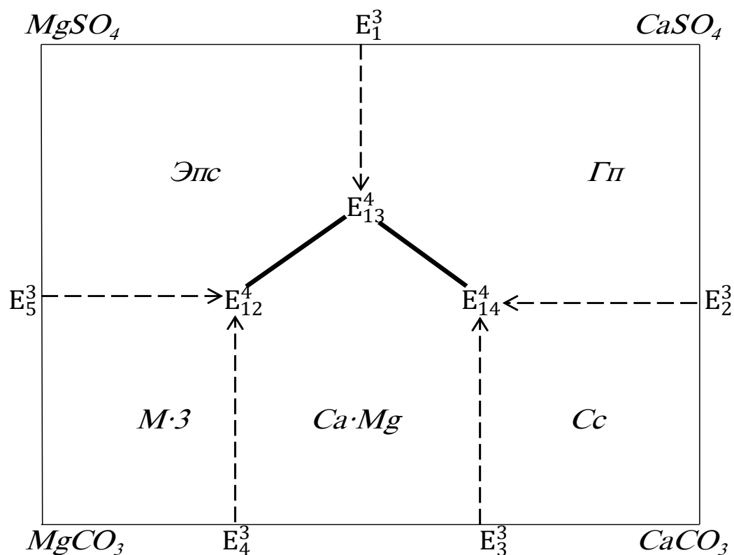
Расми 3.8. – Диаграммаи мувозинатҳои фазагии системаи \text{Ca,Mg//SO}_4,\text{CO}_3\text{-H}_2\text{O} дар ҳарорати 25\text{ }^\circ\text{C} , ки бо усули транслятсия сохта шудааст
