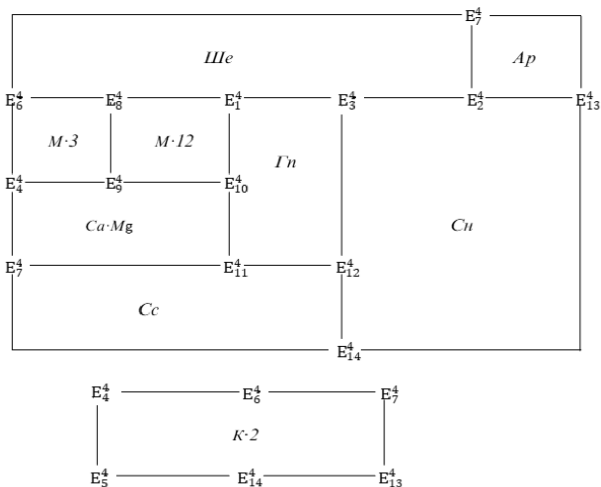
Расми 2.12. – Диаграмаи мувозинатҳои фазагии системаи K,Mg,Ca//SO 4 ,CO 3 -H 2 O дар сатҳи чоркомпонентагӣ барои ҳарорати 0 °C
