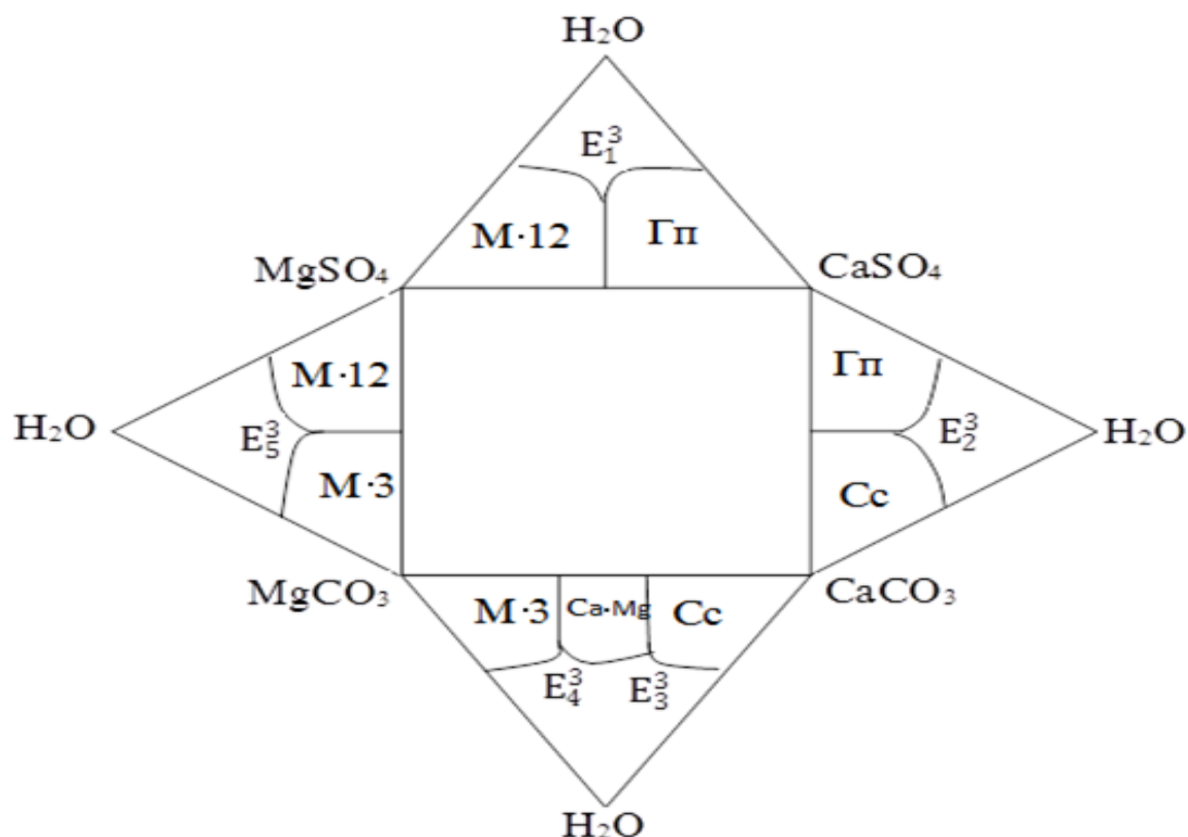
Расми 2.7. – Диаграммаи мувозинатҳои фазавии системаи \text{Ca,Mg//SO}_4\text{,CO}_3\text{-H}_2\text{O} барои ҳарорати 0^\circ\text{C} дар сатҳи секомпонентагӣ
