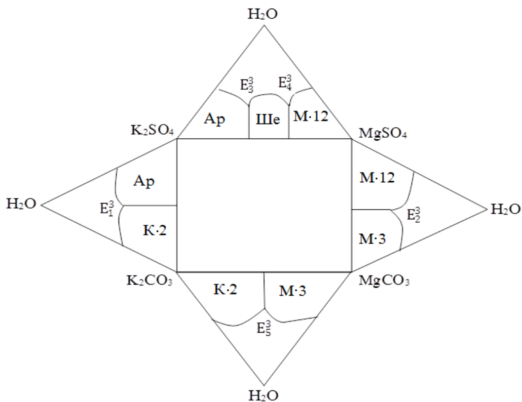
Расми 2.5. – Диаграмма мувозинатҳои фазагии системаи K, Mg//SO_4, CO_3-H_2O барои ҳарорати 0\text{ }^{\circ}C дар сатҳи секомпонентагӣ
