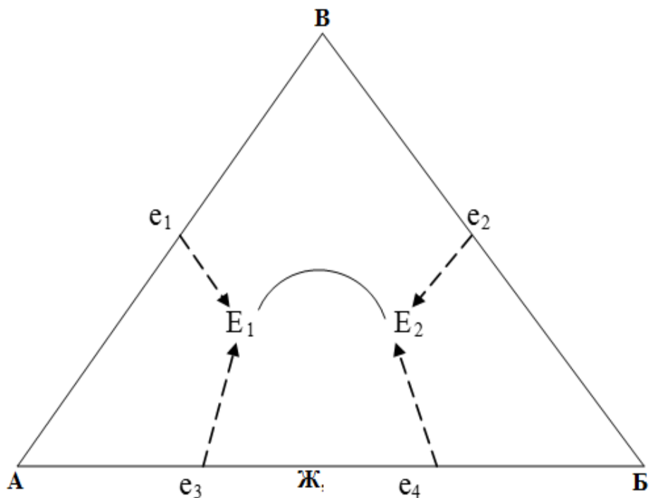
Расми 1.2. – Қисми намакии диаграммаи мувозинатҳои фазавии системаи A - B - V - \Gamma (дар ин ҷо \Gamma - ҳалкунанда), дар вақте, ки дар байни компонентҳои A ва B баҳамтаъсиркунии химиявӣ бо ҳосилшавии пайвастагии Ж қой дорад
