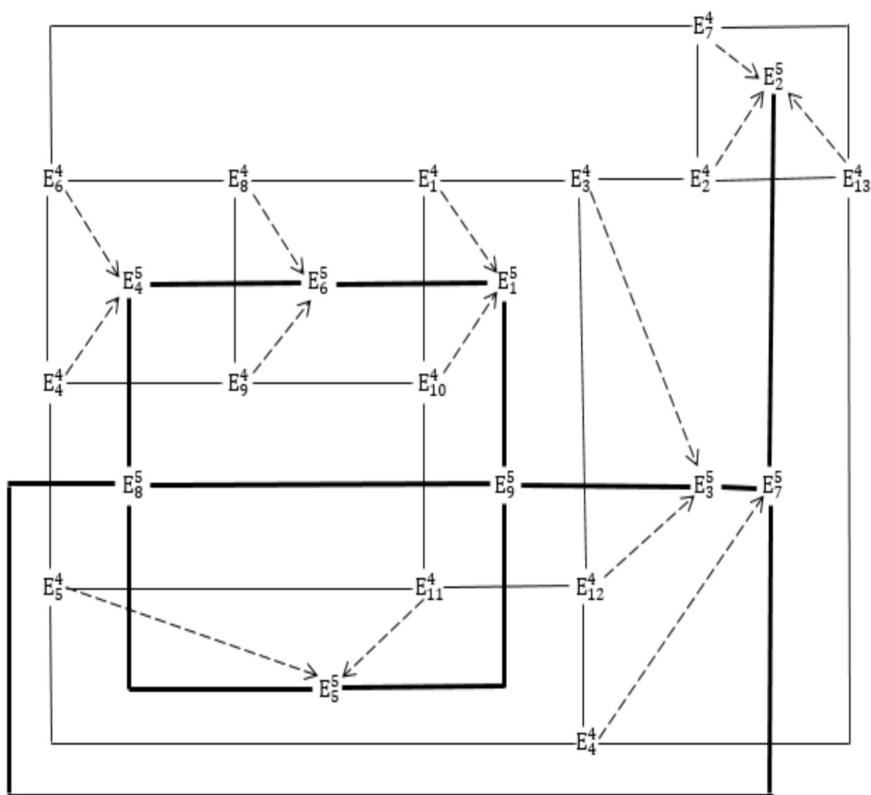
Расми 2.13. – Диаграммаи мувозинатҳои фазагии системаи K, Mg, Ca//SO_4, CO_3-H_2O дар сатҳи панҷкомпонентагӣ, барои ҳарорати 0^\circ C
