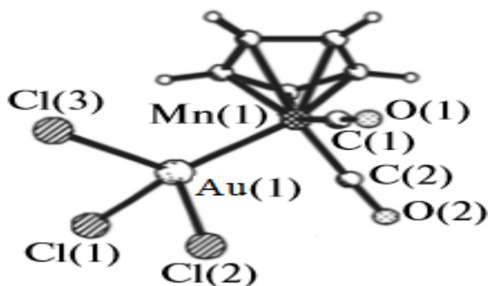
Рисунок 1.3.7. - Фрагмент молекулы координационного соединения ([\text{H}_3\text{O}][\text{Au}\{\text{S}_2\text{CN}(\text{CH}_2)_6\}]) \cdot [\text{Au}_2\{\text{S}_2\text{CN}(\text{CH}_2)_6\}_4][\text{MnCl}_4]_2)_n .
