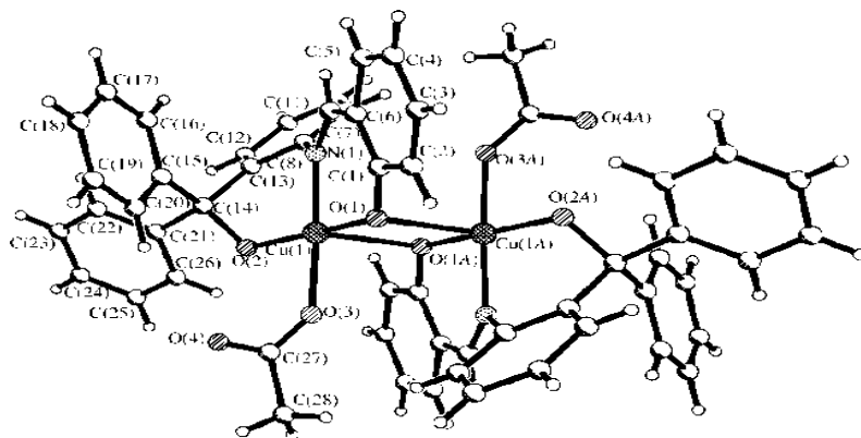
Рисунок 1.3.9. - Строение молекулы комплекса [\text{Cu}_2\text{L}_2\text{Ac}_2] .
