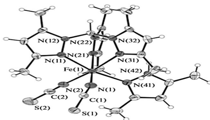
Рисунок 1.3.11. - Исследование структурных и физико-химических характеристик комплексов железа(II), содержащих роданид-ионы и лиганд \text{HC}(3,5\text{-Me}_2\text{Pz})_3 , проведено с использованием ряда спектральных и магнитных методов.
