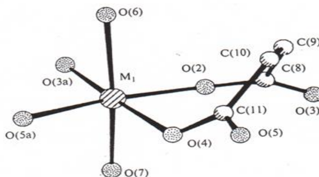
Рисунок 1.3.14. - Фрагмент координационного полиэдра нормальных малеатных комплексов состава [M(H_2O)_2(C_4H_2O_4)_2] \cdot H_2O , где M = Fe, Mn, Co, Ni(II) .
