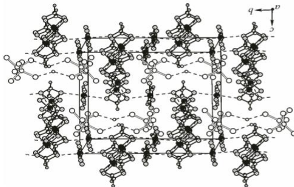
Рисунок 1.3.8. - Полимерный комплекс состава ([\text{H}_3\text{O}][\text{Au}\{\text{S}_2\text{CN}(\text{CH}_2)_6\}]\cdot[\text{Au}_2\{\text{S}_2\text{CN}(\text{CH}_2)_6\}_4][\text{MnCl}_4]_2)_n .
