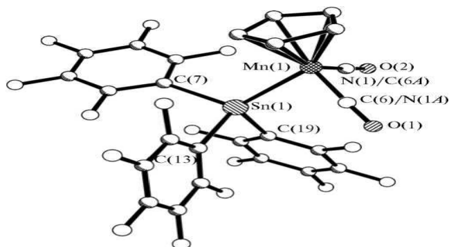
Рисунок 1.3.6. - Гетероядерное комплексное соединение, содержащее Mn: \text{C}_5\text{H}_5\text{Mn}(\text{CO})(\text{NO})\text{SnCl}_3
