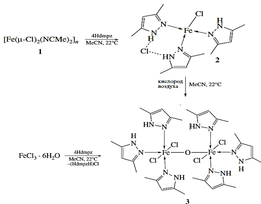
Рисунок 1.3.1. - Структура комплекса железа с азотсодержащими органическими лигандами
