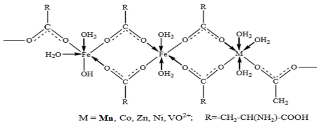
Рисунок 1.3.3. - Комплексы полимерного строения смешаннолигандных координационных соединений железа с аспарагиновой кислотой, содержащие в качестве основных координационных центров ионы \text{Fe}^{3+} и 3d-металлов.
