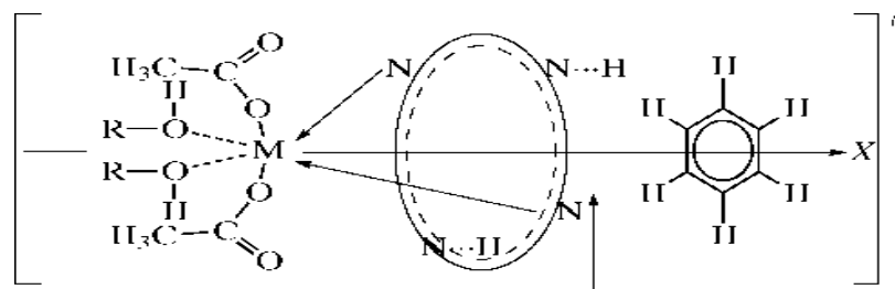
Рисунок 1.3.4. - Область экранирования связей N-H
