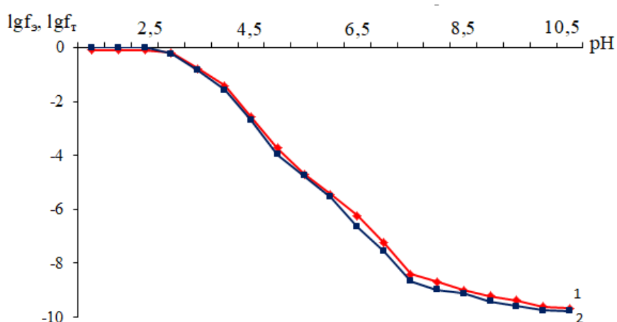
Рисунок 3.3.1. - Система железо III -железо II -марганец II -уксусная кислота-вода, T = 298,2 К. Зависимости величин логарифмов экспериментальной - f_{\text{Э}} (1) и теоретической - f_{\text{Т}} (2) окислительной функций от pH.
