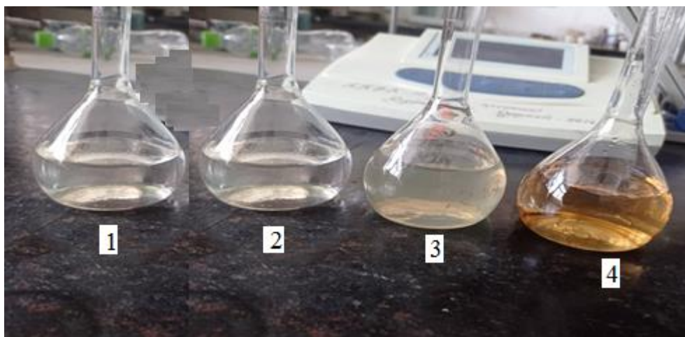
Рисунок 4.1.1. Рабочие растворы для получения гетероядерного комплекса Fe(II) - Fe(III)- и Mn(II) ацетат-ионами.
