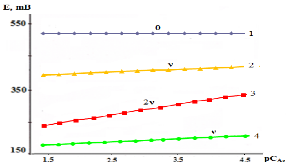
Рисунок 3.2.4. - Исследуемая система железо II -железо III -марганец II -уксусная кислота-вода и графические её зависимости ЭДС от -\lg концентрации Ас-ионов при T = 298,2 \text{ K} ; I = 1,0 ; концентрации металлов 1 \cdot 10^{-4} моль/л; рН: 1 – 2,5; 2 – 5,0; 3 – 7,0; 4 – 9,0.
