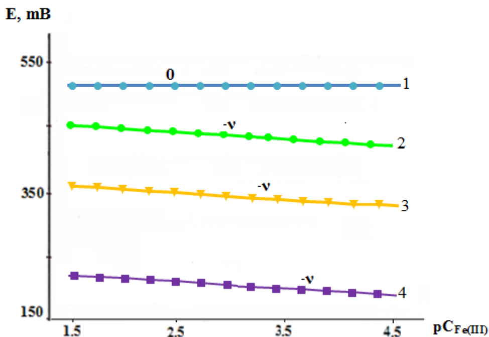
Рисунок 3.2.1. - Система железо II -железо III -марганец II -уксусная кислота-вода. Кривые зависимости ЭДС от рС Fe(III) при ионной силе раствора 1.0; концентрации металлов 1 \cdot 10^{-3} ; Ас-ионов 1 \cdot 10^{-3} моль/л и T = 298,2 К; pH: 1-2.0; 2-5.5; 3-7.0; 4-9.0.
