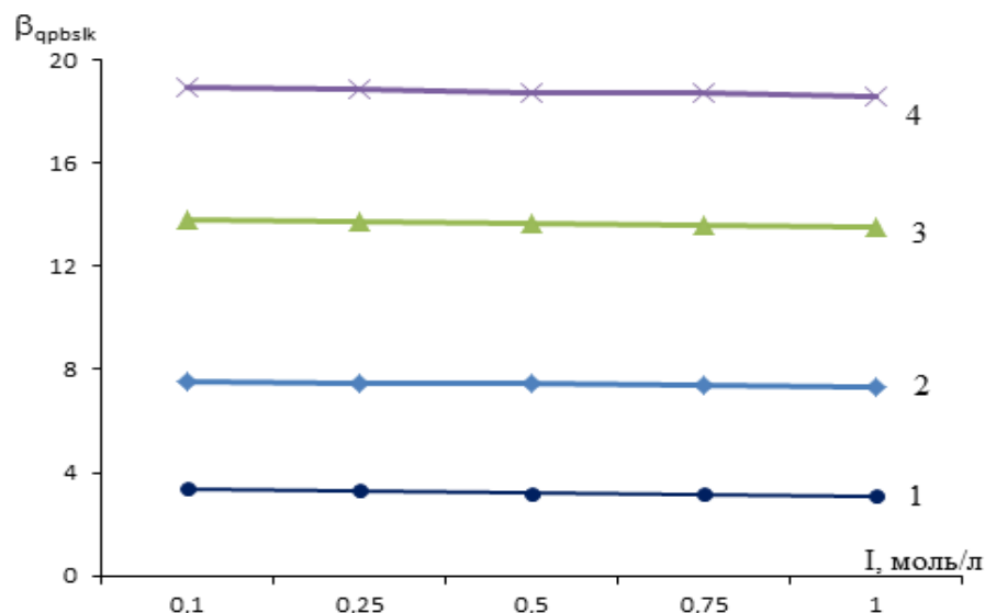
Рисунок 3.4.1. - Графическая зависимость констант устойчивости комплексов Fe(III): [\text{Fe}^{\text{III}}\text{Ac}(\text{H}_2\text{O})_5]^{2+} ; [\text{Fe}^{\text{III}}\text{AcOH}(\text{H}_2\text{O})_4]^+ ; [\text{Fe}^{\text{III}}\text{Mn}^{\text{II}}\text{Ac}(\text{H}_2\text{O})_{11}]^{4+} ; [\text{Fe}^{\text{III}}\text{Mn}^{\text{II}}\text{Ac}(\text{OH})_2(\text{H}_2\text{O})_9]^{2+} системы железо-марганец-укусная кислота-вода от I (моль/л), T = 298,2 \text{ К}
