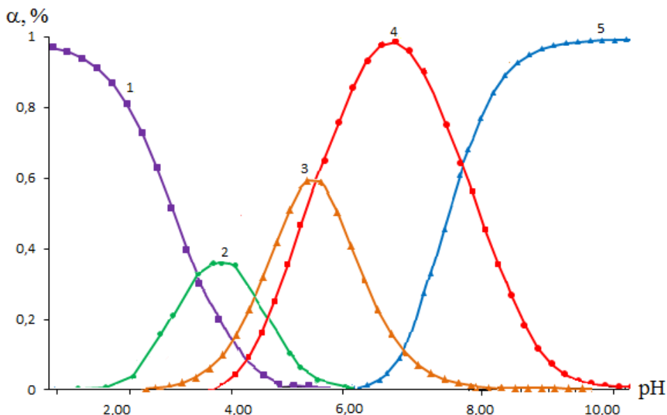
Рисунок 3.4.3. Диаграмма распределения комплексных соединений Fe(III) в системе Fe(III)-Fe(II)-Mn(II)-CH 3 COOH-H 2 O при ионной силе 1.0; C_{Mn(II)}=C_{Fe(II)}=C_{Fe(III)}=1\cdot10^{-4} ; C_{HAc}=1\cdot10^{-3} моль/л и температуре 298, 15 К. Кривые относятся: 1 – [Fe(H_2O)_6]^{3+} ; 2- [Fe^{III}Ac(H_2O)_5]^{2+} ; 3 - [Fe^{III}AcOH(H_2O)_4]^+ ; 4 - [Fe^{III}Mn^{II}Ac(H_2O)_9]^{4+} .
