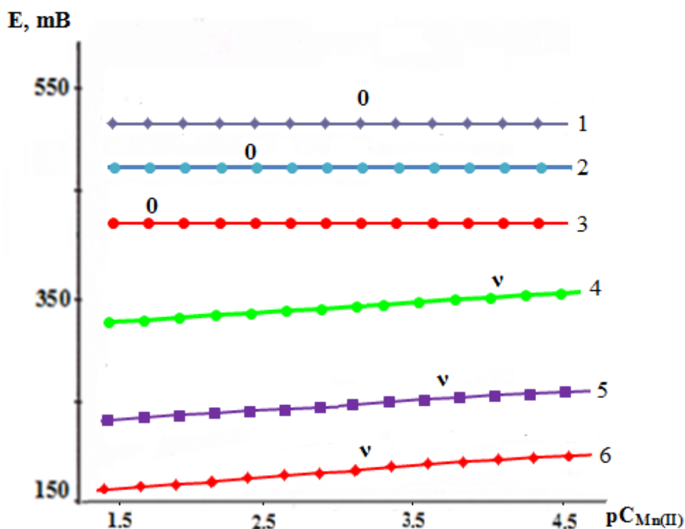
Рисунок 3.2.3. - Система железо III -марганец II -уксусная кислота-вода, графические зависимости ЭДС от -lg концентрации марганца при I = 1.0 ; концентрации металлов 1 \cdot 10^{-4} , Ас-ионов C_{HAc} = 1 \cdot 10^{-3} моль/л, T = 298,2 К; рН: 1 – 2,5; 2 – 5,0; 3 – 7,0; 4 – 9,0.
