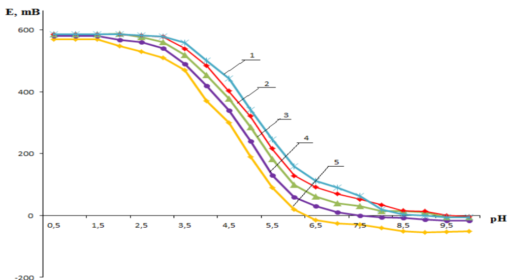
Рисунок 3.1.3. - Кривые зависимости ЭДС от pH для системы железо II -железо III -марганец II -уксусная кислота-вода при I раствора 1 - 0,10; 2 - 0,25; 3 - 0,50; 4 - 0,75; 5 - 1,00; концентрации трех металлов 1·10 -3 ; Ac-ионов 1·10 -2 моль/л, T= 298,2 К
