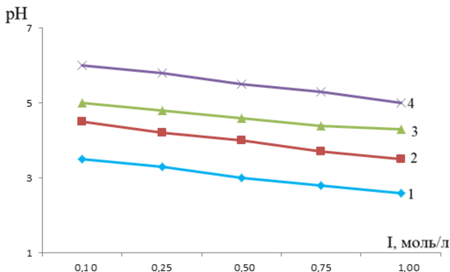
Рисунок 3.4.5. - Графическая зависимость pH начала образования комплексов Fe(III) 1 - [\text{Fe}^{\text{III}}\text{Ac}(\text{H}_2\text{O})_5]^{2+} ; 2 - [\text{Fe}^{\text{III}}\text{AcOH}(\text{H}_2\text{O})_4]^+ ; 3 - [\text{Fe}^{\text{III}}\text{Mn}^{\text{II}}\text{Ac}(\text{H}_2\text{O})_9]^{4+} ; 4 - [\text{Fe}^{\text{III}}\text{Mn}^{\text{II}}\text{Ac}(\text{OH})_2(\text{H}_2\text{O})_7]^{2+} системы железо-марганец-укусная кислота-вода от I (моль/л), T = 298,2 К
