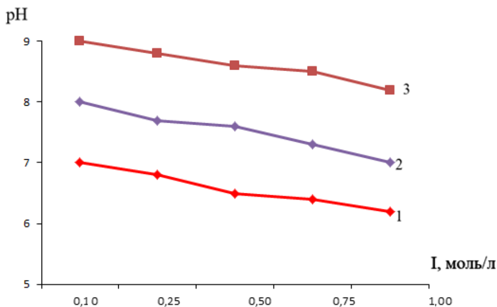
Рисунок 3.4.4. - Влияние ионной силы раствора на значение рН, соответствующее началу образования ацетатных комплексов Fe(II). от ионной силы раствора для системы Fe(III)-Fe(II)-Mn(II)-CH 3 COOH-H 2 O при C_{Fe(III)}=C_{Fe(II)}=C_{Mn(II)}=1\cdot10^{-4} и C_{HAc}=1\cdot10^{-3} моль/л, температуре 298,15 К. Кривые относятся к комплексам: 1 - [Fe^{II}Ac(H_2O)_5]^+ ; 2 - [Fe^{II}(Ac)_2(H_2O)_4]^0 ; 3 - [Fe^{II}(Ac)(OH)_2(H_2O)_3]^- .
