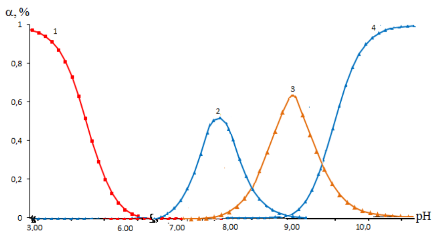
Рисунок 3.4.4. - Диаграмма распределения комплексных соединений Fe(II) в системе Fe(III)-Fe(II)-Mn(II)-CH 3 COOH-H 2 O при ионной силе 1.0; C_{\text{Mn(II)}}=C_{\text{Fe(II)}}=C_{\text{Fe(III)}}=1 \cdot 10^{-4} ; C_{\text{HAc}}=1 \cdot 10^{-3} моль/л и температуре 298, 15 К. Кривые относятся: 1 – [\text{Fe}(\text{H}_2\text{O})_6]^{2+} ; 2- [\text{Fe}^{\text{II}}\text{Ac}(\text{H}_2\text{O})_5]^+ ; 3- [\text{Fe}^{\text{II}}(\text{Ac})_2(\text{H}_2\text{O})_4]^0 ; 4 - [\text{Fe}^{\text{II}}(\text{Ac})(\text{OH})_2(\text{H}_2\text{O})_3]^- .
