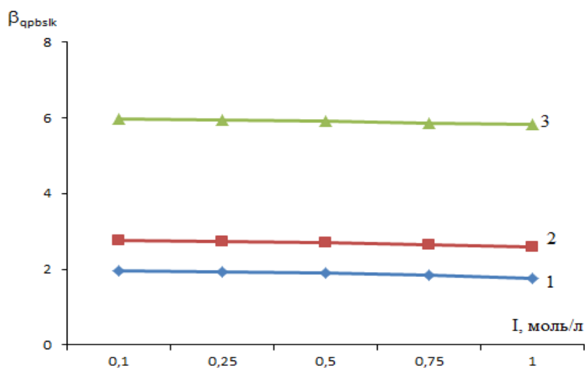
Рисунок 3.4.2. - Графическая зависимость констант устойчивости комплексов Fe(II): 1- [\text{Fe}^{\text{II}}\text{Ac}(\text{H}_2\text{O})_5]^+ ; 2- [\text{Fe}^{\text{II}}(\text{Ac})_2(\text{H}_2\text{O})_4]^0 ; 3- [\text{Fe}^{\text{II}}(\text{Ac})(\text{OH})_2(\text{H}_2\text{O})_3]^- системы железо-марганец-укусная кислота-вода от I (моль/л), T = 298,2 \text{ K} .
