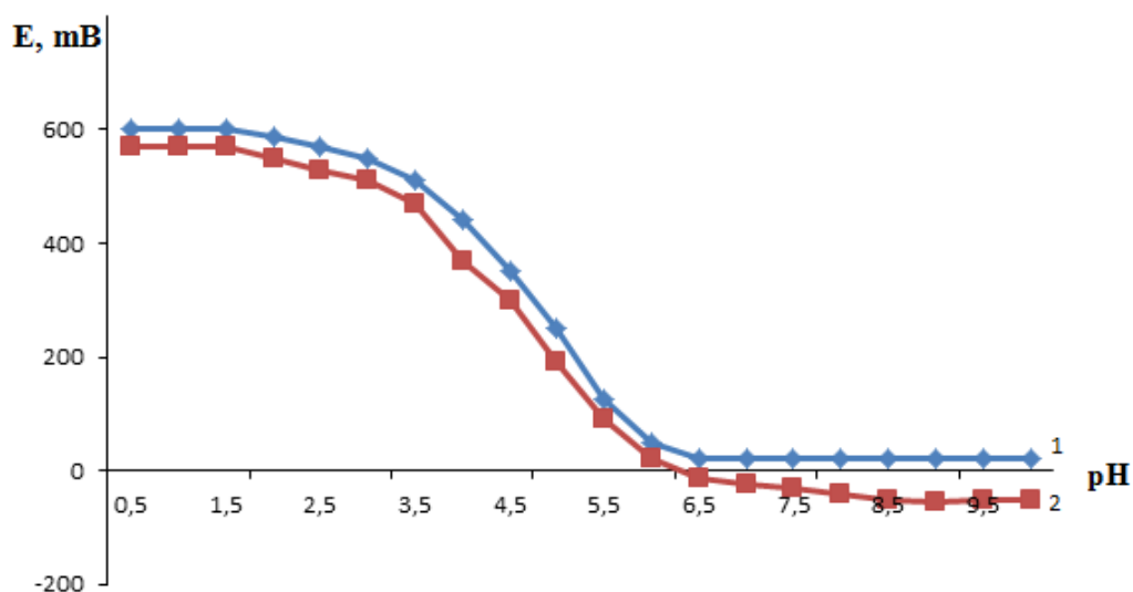
Рисунок 3.1.1. - Графические зависимости ЭДС системы железо(II)-железо(III)-уксусная кислота-вода (кр. 1) и железо(II)-железо(III)-марганец(II)-уксусная кислота-вода (кр. 2) от pH при I = 1,0; концентрации всех трех металлов 1·10 -3 ; Ac – иона 1·10 -2 моль/л, T = 298,2 К.
