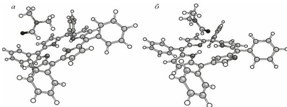
Рисунок 1.3.5. - Типы взаимодействия молекул диметилформамида.
