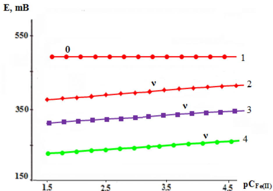
Рисунок 3.2.2. - Система железо II -железо III -марганец II -уксусная кислота-вода. Кривые зависимости ЭДС от pC_{Fe(II)} при ионной силе раствора 1,0; концентрации металлов 1 \cdot 10^{-4} ; Ас-ионов 1 \cdot 10^{-3} моль/л и T = 298,2 К.
