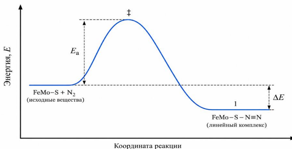
Рисунок 1.2.1. - Схема фиксации азотата. 1 - образование линейного комплекса
