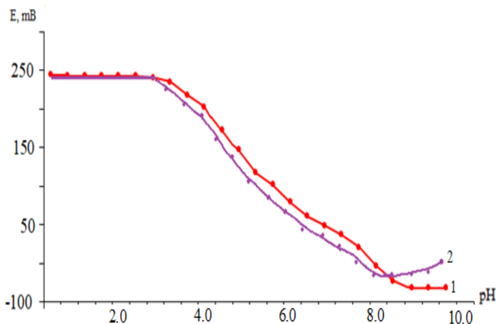
Рисунок 3.1.2. - Кривые зависимости ЭДС системы железо II -железо III -марганец II -уксусная кислота-вода от pH при I раствора 1.0; концентрации всех трех металлов 1 \cdot 10^{-4} моль/л, T = 1- 308,2; 2- 318,2 К.
