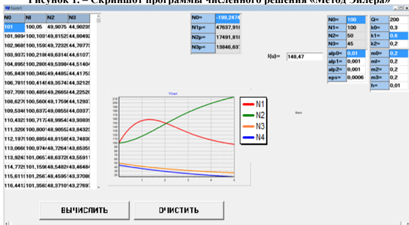
Рисунок 2. – Скриншот программы «Метод Эйлера»
