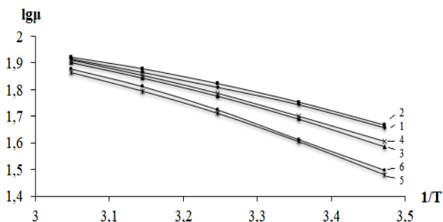
Расми 6. - Вобастагии ҳароратии ҷараёнгузаронии молярӣ \lg\mu аз 1/T , 1-[Ag(C 7 H 6 N 2 S)(H 2 O) 3 NO 3 ]; 2-[Ag(C 7 H 6 N 2 S) 2 (H 2 O) 2 NO 3 ]; 3-[Ag(C 7 H 6 N 2 S) 2 Cl]; 4-[Ag(C 7 H 6 N 2 S) 2 Br]; 5-[Ag(C 7 H 6 N 2 S) 2 (H 2 O) 2 SO 4 ] и 6-[Ag(C 7 H 6 N 2 S) 2 (H 2 O)SCN]
