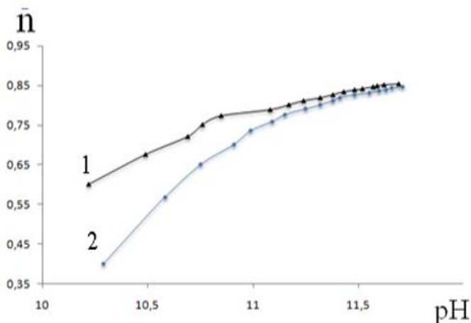
Рисунок 1. – Зависимость \bar{n} от рН при 1-10 и 2-25 об.% метанола при 298К.
