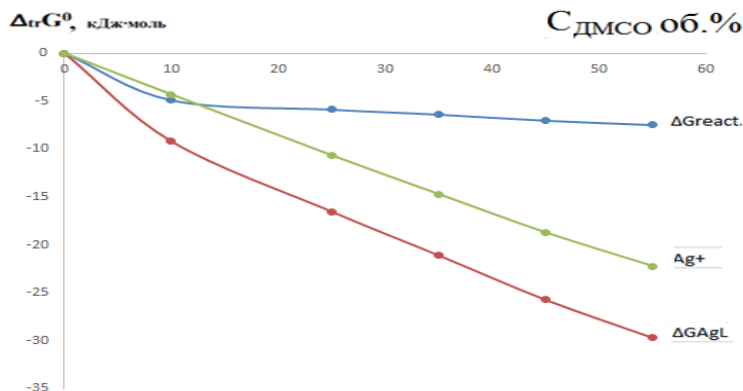
Расми 5.- Тағйирёбии энергияи Гиббси ҳосилшавии комплексҳои нукра бо 2-меркаптобензимидазол дар ДМСО
