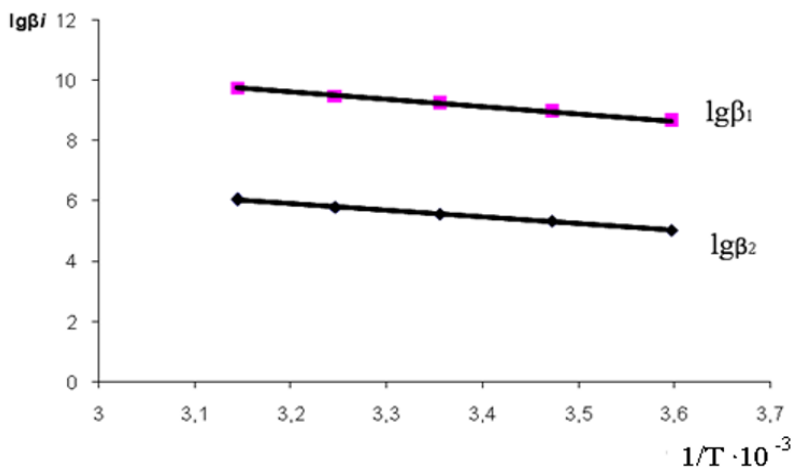
Расми 2. - Вобастагии \lg\beta_i аз 1/T барои ҳосилшавии комплексҳои 2-меркаптобензимидазолии нукра
