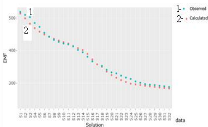
Рисунок.3. – Изменение потенциала системы \text{Ag}^+/\text{Ag}^0 для образования комплексных форм серебра (I) с 2-меркаптобензимидазолом. Салс-теорет. и Obs.-эксп.
