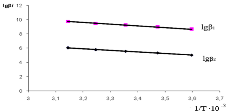
Рисунок 2. – Зависимость \lg\beta_i от 1/T для образования 2-меркаптобензимидазольных комплексов серебра
