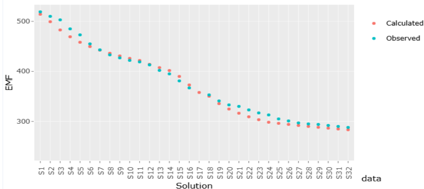
Расми 4. - Тағйирёбии потенциали системаи Ag^+/Ag^0 барои ҳосилшавии шаклҳои комплекси нукра (I) бо 2-меркаптобензимидазол. Calc-наз. ва Obs.-таҷр.
