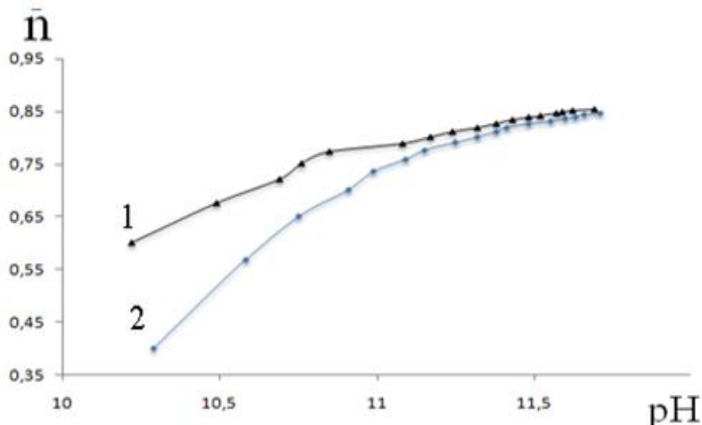
Расми 1. - Вобастагии \bar{n} аз рН 2-25 ҳаҷм.% метанол дар 298 К.
