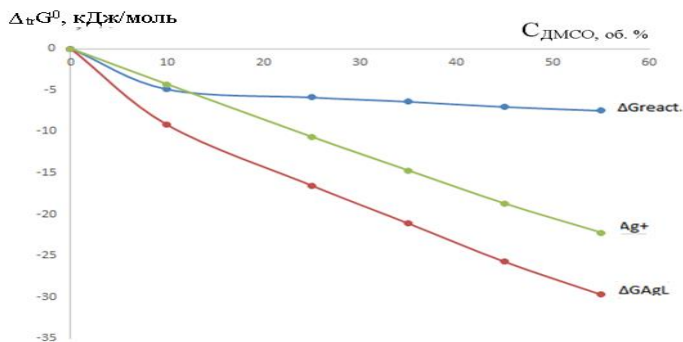
Рисунок 4. – Изменение энергии Гиббса образования комплексов серебра с 2-меркаптобензимидазолом в ДМСО
