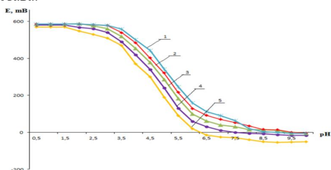
Рисунок 3. - Кривые зависимости ЭДС от pH для системы железо II -железо III -марганец II -уксусная кислота-вода при I раствора 1 - 0,10; 2 - 0,25; 3 - 0,50; 4 - 0,75; 5 - 1,00; концентрации трех металлов 1 \cdot 10^{-3} ; Ас-ионов 1 \cdot 10^{-2} моль/л, T = 298,2 К.
