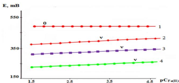
Рисунок 5. - Система железо II -железо III -марганец II -уксусная кислота-вода. Кривые зависимости ЭДС от pC_{Fe(II)} при ионной силе раствора 0,5; концент. металлов 1 \cdot 10^{-4} ; Ас-ионов 1 \cdot 10^{-3} моль/л и T = 298,2 К.
