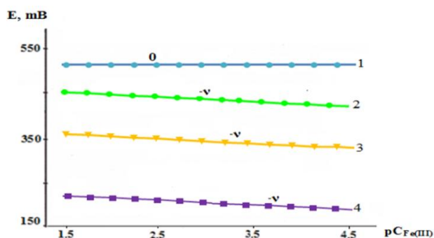
Расми 4. - Системаи оҳан(II)-оҳан(III)-манган(II)-кислотаи атсетат-об. Качхаттаҳои вобастагии ҚЭХ аз рН аз pC_{Fe(III)} ҳангоми қувваи ионии маҳлул 1,00; консентратсияи метал 1 \cdot 10^{-3} ; Ас-ионов 1 \cdot 10^{-3} мол/л ва T=298,2 К, рН: 1-2,0; 2-5,5; 3-7,0; 4-9,0.
