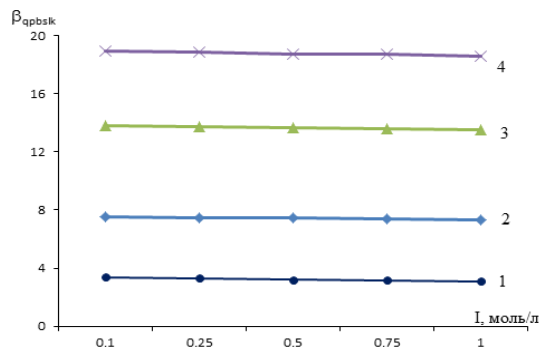
Рисунок 11. - Графическая зависимость констант устойчивости комплексов \text{Fe(III)} : [\text{Fe}^{\text{III}}\text{Ac}(\text{H}_2\text{O})_5]^{2+} ; [\text{Fe}^{\text{III}}\text{AcOH}(\text{H}_2\text{O})_4]^+ ; [\text{Fe}^{\text{III}}\text{Mn}^{\text{II}}\text{Ac}(\text{H}_2\text{O})_{11}]^{4+} ; [\text{Fe}^{\text{III}}\text{Mn}^{\text{II}}\text{Ac}(\text{OH})_2(\text{H}_2\text{O})_9]^{2+} системы железо(III)-железо (II)-марганец(II)-уксусная кислота-вода от I (моль/л), T = 298,2 К.
