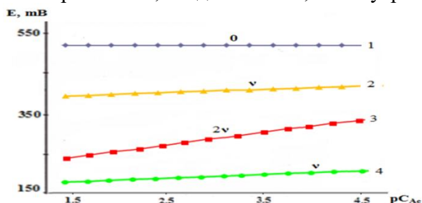
Рисунок 7. - Исследуемая система железо II -железо III -марганец II -уксусная кислота-вода и графические её зависимости ЭДС от -lg конц. Ас-ионов при T = 298,2 К; I = 1,0 ; концент. металлов 1 \cdot 10^{-4} моль/л, pH : 1 – 2,5; 2 – 5,0; 3 – 7,0; 4 – 9,0.
