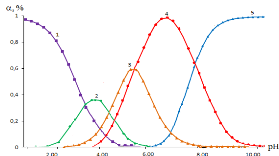
Рисунок 9. - Система железо(III)-железо(II)-марганец(II)-укусная кислота-вода, T = 298,2 \text{ K} , I (\text{моль/л}) = 1,0 ; Кривые диаграммы распределения комплексов железа(III) относятся: 1 – аквакомплекс [\text{Fe}(\text{H}_2\text{O})_6]^{3+} 2- [\text{Fe}^{\text{III}}\text{Ac}(\text{H}_2\text{O})_5]^{2+} ; 3 - [\text{Fe}^{\text{III}}\text{AcOH}(\text{H}_2\text{O})_4]^+ ; 4 - [\text{Fe}^{\text{III}}\text{Mn}^{\text{II}}\text{Ac}(\text{H}_2\text{O})_9]^{4+} .
