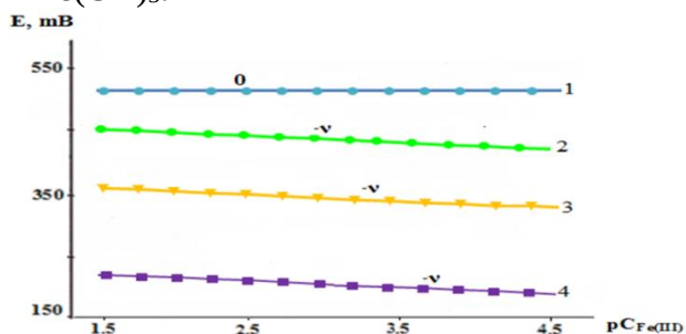
Рисунок 4. - Система железо II -железо III -марганец II -уксусная кислота-вода. Кривые зависимости ЭДС от pC_{Fe(III)} при ионной силе раствора 1.0; концент. металлов 1 \cdot 10^{-3} ; Ас-ионов 1 \cdot 10^{-3} моль/л и T = 298,2 К, pH: 1- 2.0; 2-5.5; 3-7.0; 4-9.0.
