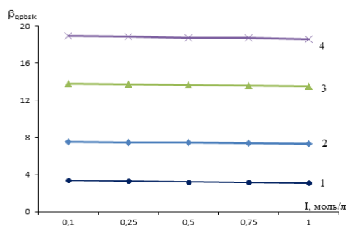
Расми 11. - Вобастагии графikiи константҳои устувории комплекси \text{Fe}(\text{III}) : [\text{Fe}^{\text{III}}\text{Ac}(\text{H}_2\text{O})_5]^{2+} ; [\text{Fe}^{\text{III}}\text{AcOH}(\text{H}_2\text{O})_4]^+ ; [\text{Fe}^{\text{III}}\text{Mn}^{\text{II}}\text{Ac}(\text{H}_2\text{O})_{11}]^{4+} ; [\text{Fe}^{\text{III}}\text{Mn}^{\text{II}}\text{Ac}(\text{OH})_2(\text{H}_2\text{O})_9]^{2+} барои системаи оҳан(III)-оҳан(II)-манган(II)-кислотаи атсетат-об аз I (мол/л), T = 298,2 \text{ K} .
