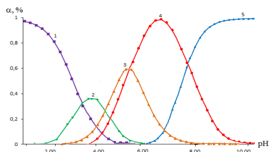
Расми 9. - Системаи оҳан(III)-оҳан(II)-манган(II)-кислотаи атсетат-об, T = 298,2 K, I (мол/л)=1.0; Качхатҳои диаграммаи тақсимои комплекси оҳан(III) тааллуқдоранд: 1 – аквакомплекс [Fe(H_2O)_6]^{3+} ; 2- [Fe^{III}Ac(H_2O)_5]^{2+} ; 3 - [Fe^{III}AcOH(H_2O)_4]^+ ; 4 - [Fe^{III}Mn^{II}Ac(H_2O)_9]^{4+} .
