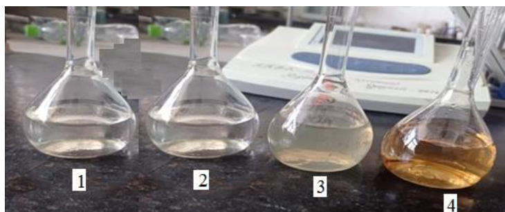
Рисунок 12. - Рабочие растворы для получения гетероядерного комплекса Fe(III) и Mn(II) с ацетат-ионами. Колбы с растворами: 1 - уксусная кислота; 2 - сульфат марганца - \text{MnSO}_4 ; 3 - сульфат железа(II) - \text{FeSO}_4 ; 4 - сульфат железа (III) - \text{Fe}_2(\text{SO}_4)_3 .
