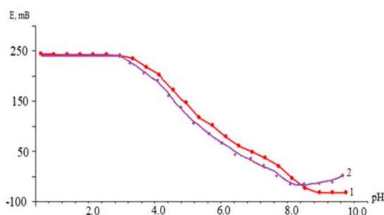
Рисунок 2 - Кривые зависимости ЭДС системы железо II -железо III -марганец II -уксусная кислота-вода от pH при I раствора 1.0; концентрации всех трех металлов 1 \cdot 10^{-4} моль/л, T = 1- 308,15; 2- 318,15 К.
