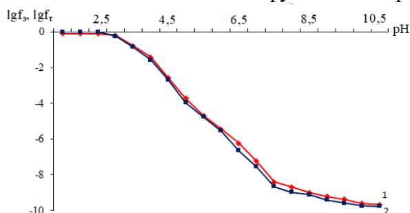
Рисунок 8. - Система железо III -железо II -марганец II -укусная кислота-вода, T = 298,2 \text{ K} . Зависимости величин логарифмов экспериментальной - f , (1) и теоретической - f_t (2) окислительных функций от pH.
