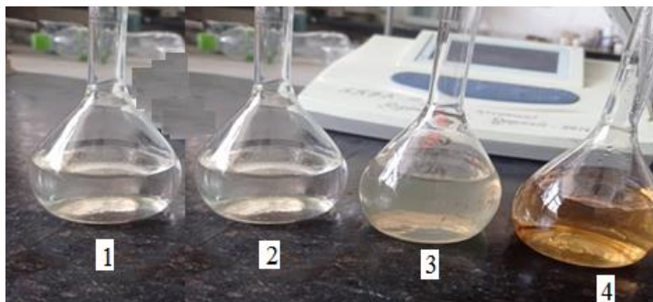
Расми 12. - Маҳлулҳои корӣ барои ба даст овардани комплекси гетероядроии Fe(III) ва Mn(II) бо ионҳои атсетат. Колбаҳо бо маҳлулҳо: 1 - кислотаи атсетат; 2 - сульфати манган - \text{MnSO}_4 ; 3 - сульфати оҳан(II) - \text{FeSO}_4 ; 4 - сульфати оҳан(III) - \text{Fe}_2(\text{SO}_4)_3 .
