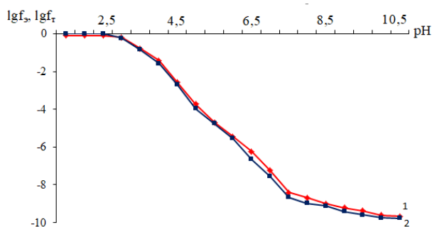
Расми 8. - Системаи оҳан(III)-оҳан(II)-манган(II)-кислотаи атсетат-об, T = 298,2 К. Вобастагии бузургҳои логарифмҳои функсияҳои таҷрибавӣ - f_1 (1) ва назариявӣ- f_2 (2) аз pH.
