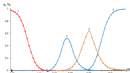
Расми 10. - Системаи оҳан(III)-оҳан(II)-манган(II)-кислотаи атсетат-об, T = 298,2 \text{ K} , I (\text{мол/л}) = 1,0 ; Диаграммаҳои қачхатҳои тақсимшавии комплекси оҳан(II) инҳоянд: 1 - аквакомплекс [\text{Fe}(\text{H}_2\text{O})_6]^{2+} ; 2- [\text{Fe}^{\text{II}}\text{Ac}(\text{H}_2\text{O})_5]^+ ; 3 [\text{Fe}^{\text{II}}(\text{Ac})_2(\text{H}_2\text{O})_4]^0 ; 4 - [\text{Fe}^{\text{II}}(\text{Ac})(\text{OH})_2(\text{H}_2\text{O})_3]^- .
