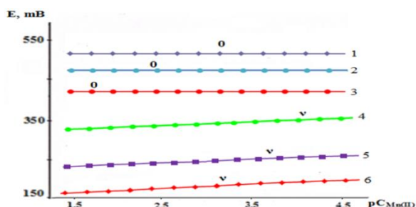
Рисунок 6. - Система железо III -марганец II -уксусная кислота-вода, графические зависимости ЭДС от -lg конц. марганца при I = 1,0 ; концент. металлов 1 \cdot 10^{-4} , Ас-ионов 1 \cdot 10^{-3} моль/л, T = 298,2 К, pH : 1 – 2,5; 2 – 5,0; 3 – 7,0; 4 – 9,0.
