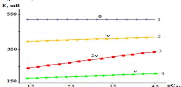
Расми 7. - Системаи оҳан(II)-оҳан(III)-манган(II)-кислотаи атсетат-об ва Качхаттаҳои вобастагии ҚЭХ аз -lg конс. Ас-ионҳо ҳангоми T = 298,2 К; I=1,0 ; консен. металҳо 1 \cdot 10^{-4} мол/л, рН: 1 – 2,5; 2 – 5,0; 3 – 7,0; 4 – 9,0.
