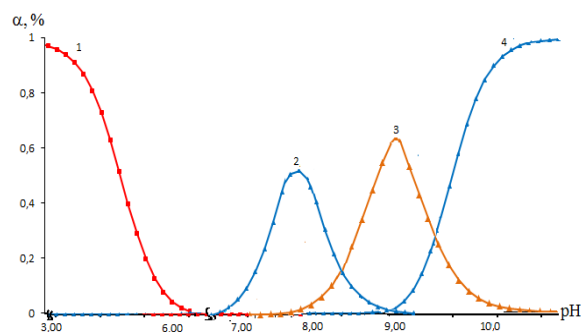
Рисунок 10. - Система железо(III)-железо (II) - марганец(II)-укусная кислота-вода, T = 298,2 К, I (моль/л) =1.0; Кривые диаграммы распределения комплексов железа(II) относятся: 1 - аквакомплекс [\text{Fe}(\text{H}_2\text{O})_6]^{2+} ; 2 - [\text{Fe}^{\text{II}}\text{Ac}(\text{H}_2\text{O})_5]^+ ; 3- [\text{Fe}^{\text{II}}(\text{Ac})_2(\text{H}_2\text{O})_4]^0 ; 4 - [\text{Fe}^{\text{II}}(\text{Ac})(\text{OH})_2(\text{H}_2\text{O})_3]^- .
