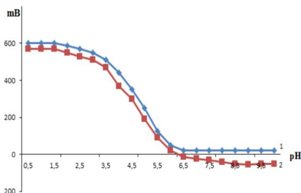
Рисунок 1. - Графические зависимости ЭДС системы железо(II)-железо(III)-уксусная кислота-вода (кр. 1) и железо(II)-железо(III)-марганец(II)-уксусная кислота-вода (кр. 2) от pH при I = 1,0 ; концентрации всех трех металлов 1 \cdot 10^{-3} ; Ас – иона 1 \cdot 10^{-2} моль/л, T = 298,2 К.
