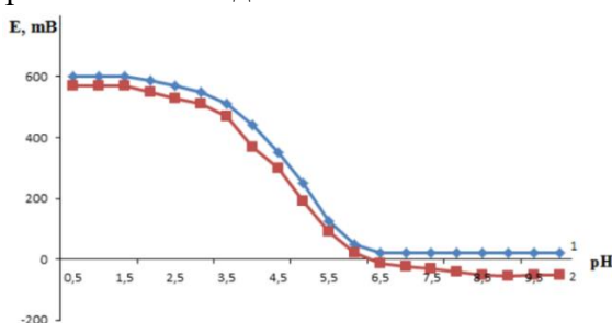
Расми 1. - Вобастагии графический ҚЭХ-и системаи оҳан(II)-оҳан(III)-кислотаи атсетат-об (кач. 1) ва оҳан(II)-оҳан(III)-манган(II)-кислотаи атсетат-об (кач. 2) аз pH дар I = 1,0; концентратсияи ҳар се метал 1 \cdot 10^{-3} ; Ас – ион 1 \cdot 10^{-2} мол/л, T = 298,2 К.
