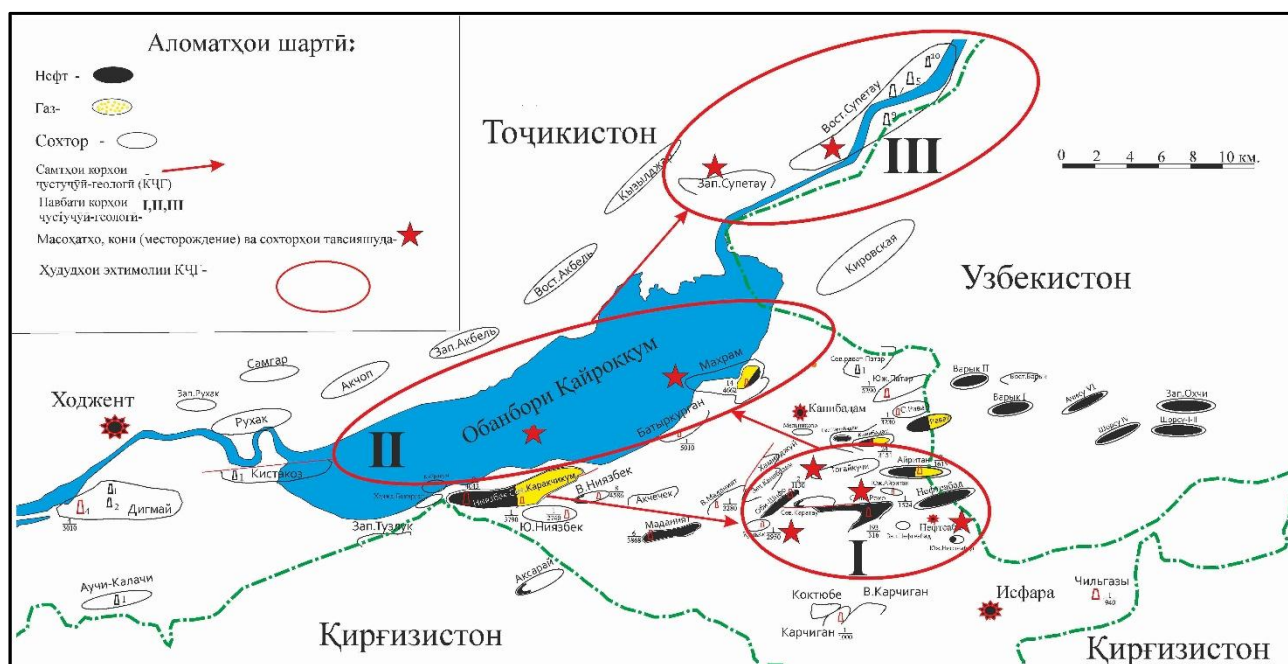
Расми 11. — Схемат азҳудкунии маҷмӯии сохторҳои нафтугаздор ва самтҳои афзалиятноки КҒР дар қисми ғарбии пастхамии Фарғона (Мураттибон: Раҳимов Ф.А., Мавлонӣ С.Р., соли 2025)
