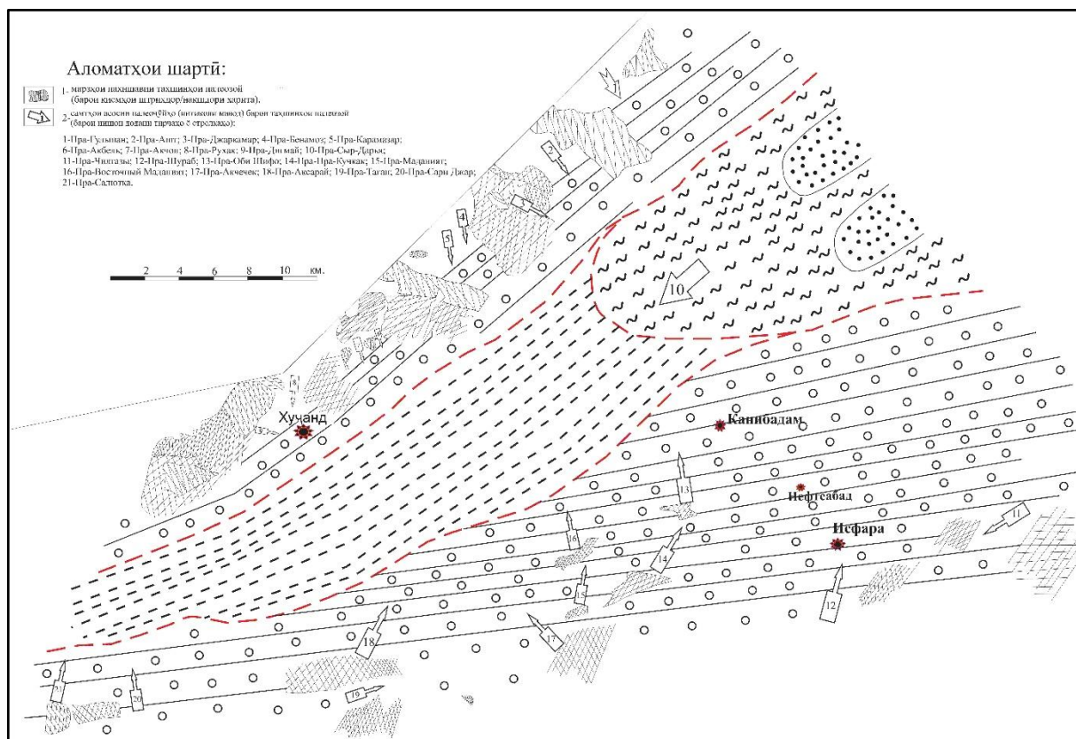
Расми 8. — Харитаи схематикӣ палеочуғрофии даврани чамъшавии таҳшинҳои мезосикли аввал (табошири поёӣ). (Ишораҳои шартӣ палеоландшафтҳо дар расми 10 бинед) (Мураттибон: Раҳимов Ф.А., Мавлонӣ С.Р., соли 2025)
