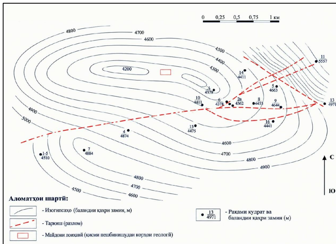
Расми 6. – Харитаи сохтори рӯи (кровля) қабати II-и майдони Махрам (Мурағтӣбон: Мавлони С.Р., Раҳимов Ф.А., соли 2025)
