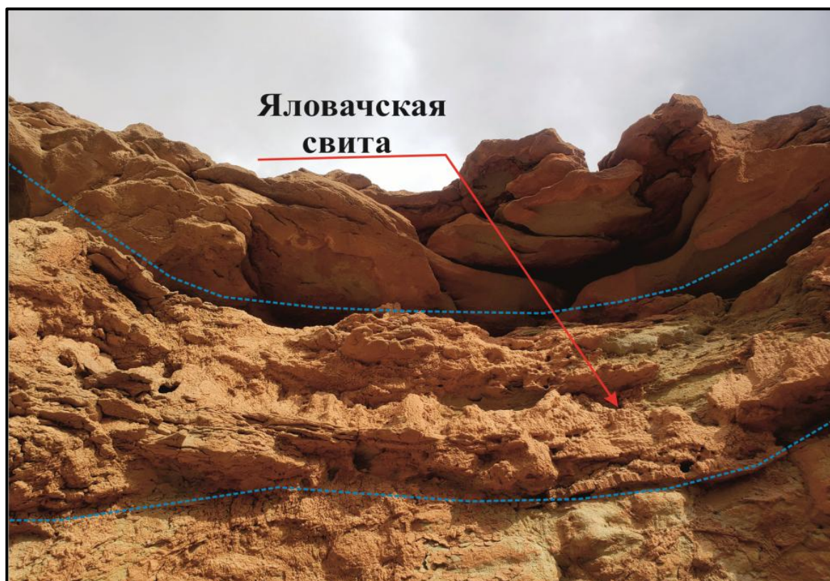
Рисунок 3.- Фото отложения яловачской свиты (поселок Нефтеабад) (Составил Рахимова Ф.А., 2025 год)
