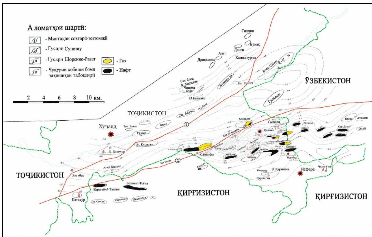
Расми 4. — Харитаи сохторӣ аз рӯи болон (кровляи) қабати (свитаи) Гознау (Мураттибон: Раҳимов Ф.А., Мавлонӣ С.Р., соли 2025)
