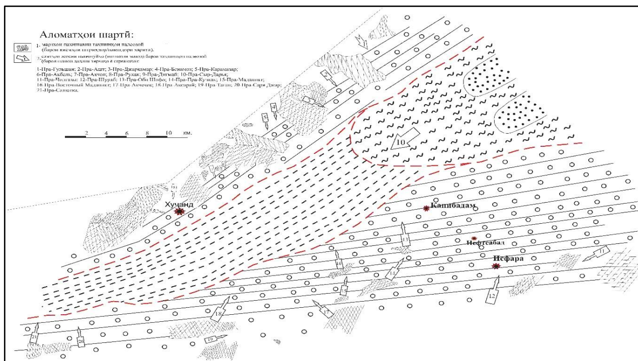
Расми 10. — Харитаи схематикӣ палеочуғрофии давраи ҷамъшавии тахшинҳои свитаи Экзогир (турони поёнӣ) (Мураттибон: Раҳимов Ф.А., Мавлонӣ С.Р., соли 2025)
