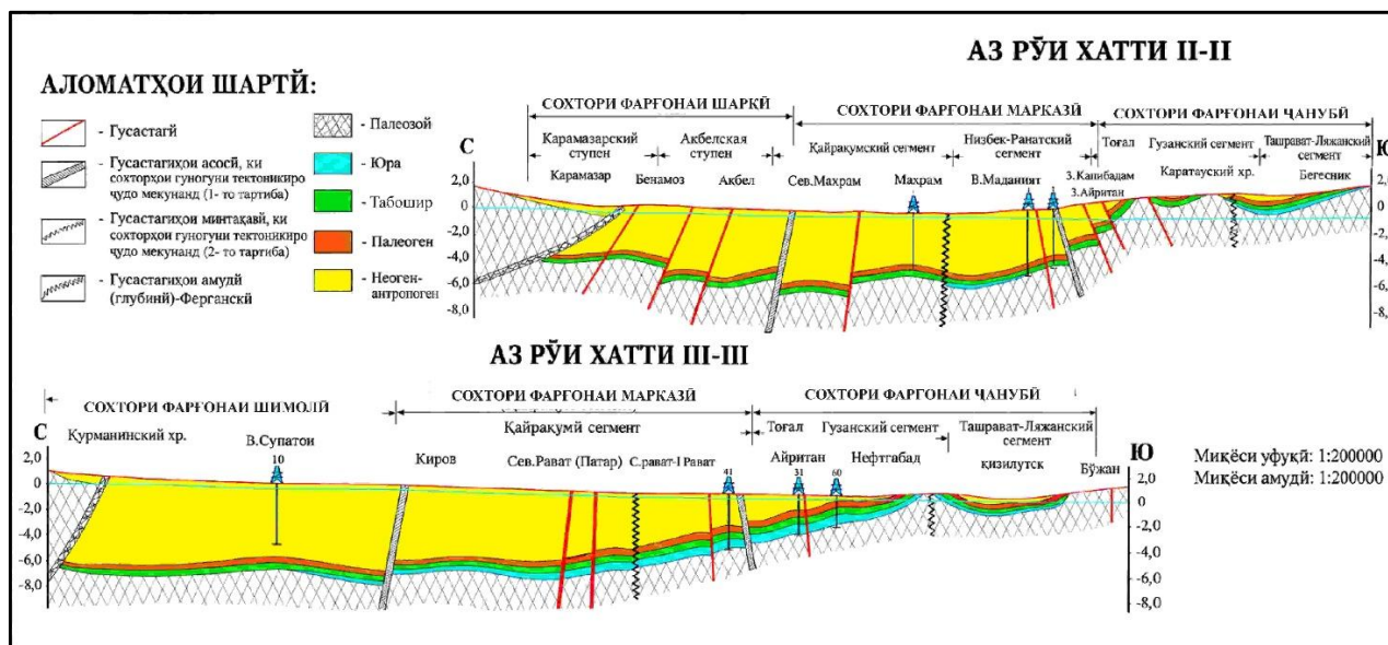
Расми 5. — Схемани сохти умқии МСТ-и шимолӣ (Мураттибон: Мавлонӣ С.Р., Раҳимов Ф.А., соли 2025)
