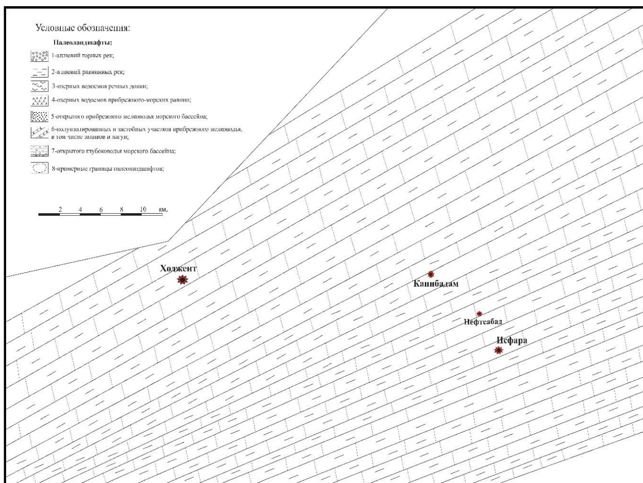
Рисунок 10. - Схематическая палеогеографическая карта времени накопления осадков экзогировой свиты (нижний Турон) (Составили Рахимов Ф.А., Мавлони С.Р., 2025 год)
