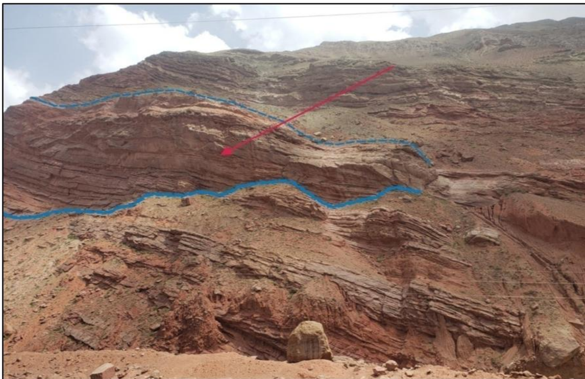
Расми 9. — Шусташавии дохилиформатсионӣ (внутриформационный размыв) дар қумсангҳои свитаи Яловач (Муратгиб: Раҳимов Ф.А., соли 2025)
