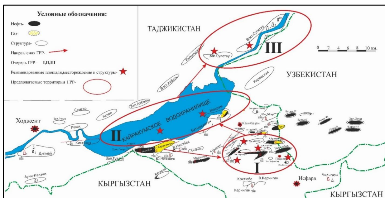
Рисунок 11. - Схема комплексного освоения нефтегазоносных структур и приоритетные направления ГРП в Западной части Ферганской впадины (Составили Рахимов Ф.А., Мавлони С.Р., 2025 год)
