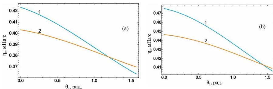
Рис. 5. Зависимость \eta_s(\omega) метанола от углов \theta_1 и \theta_2 при фиксированном \xi_1-\xi_2=0^\circ и температуре t=20^\circ\text{C} , линии 1 по формуле (6) и линии 2 по формуле (1).
