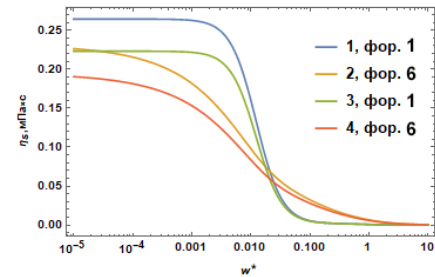
Рис. 1. Изотермическая частотная зависимость \eta_s(\omega) жидкого CH 4 : 1 и 2 при T=100 К; 3 и 4 при T=150 К.
