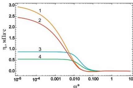
Расм 3. Вобастагии басомадии коэффицентҳои часпакии ҳаҷмӣ \eta_v(\omega) барои метанол дар температураҳои t=10 °C (хатҳои 1,3), t=40 °C (хатҳои 2,4) ва зичиҳои мутобиқи онҳо ҳангоми доимӣ будани \theta_1 = 30^\circ , \theta_2 = 45^\circ , \xi_1 - \xi_2 = 0^\circ ; хатҳои 1 ва 2 бо формулаи (7) ва хатҳои 3 ва 4 бо формулаи (2) ҳисоб шудаанд.
