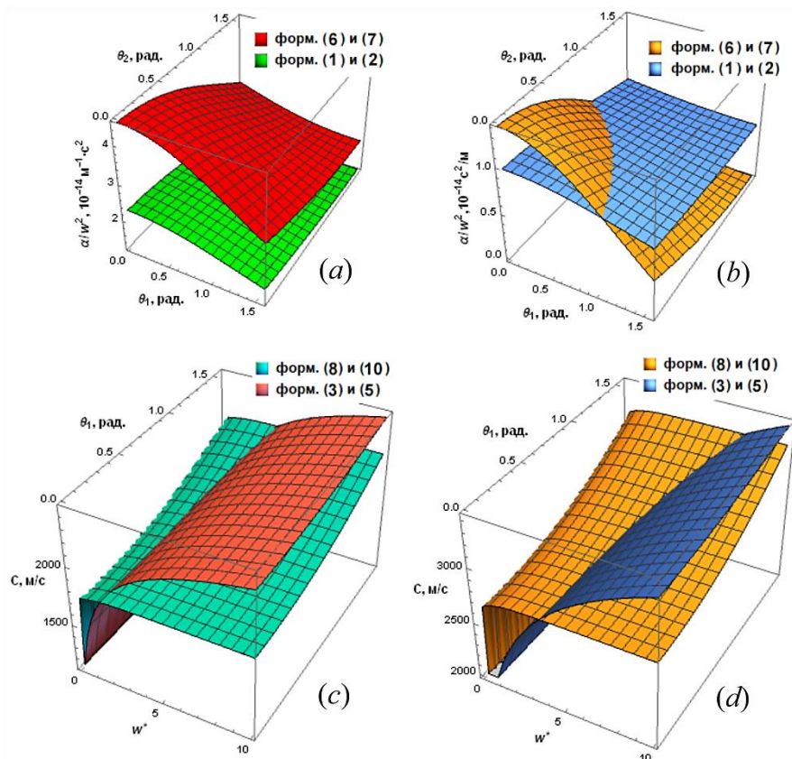
Расм 8. Вобастагии коэффисенти фурубурд \alpha/\omega^2 ва суръати C(\omega) мавҷҳои садо аз кунҷҳои \theta_1 ва \theta_2 дар мавриди доими будани \xi_1 - \xi_2 = 0^\circ : (а) ва (б) - барои спирти метилӣ барои температураи t=20^\circ\text{C} ; (с) ва (д) - барои об дар температураи t=40^\circ\text{C} .
