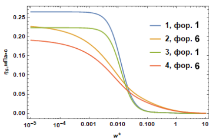
Расм 1. Вобастагии басомадии изотермии \eta_s(\omega) барои метани моеъ ( \text{CH}_4 ): хатҳои 1 ва 2 дар температураи T=100 К; хатҳои 3 ва 4 дар температураи T=150 К.
