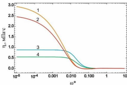
Рис. 4. Частотная зависимость коэффициента объемной \eta_v(\omega) вязкости метанола при температурах t=10 °C (линии 1,3), t=40 °C (линии 2,4) и соответствующих им
