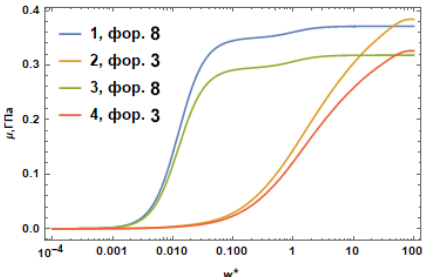
Рис. 2. Изотермическая частотная зависимость \mu(\omega) жидкого CH 4 : 1 и 2 при T=100 К; 3 и 4 при T=150 К.
