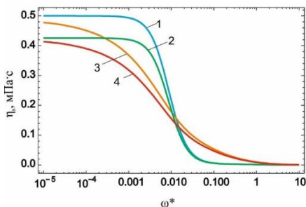
Рис. 3. Частотная зависимость коэффициента сдвиговой \eta_s(\omega) вязкости метанола при температурах t=10 °C (линии 1,3), t=40 °C (линии 2,4) и соответствующих им
