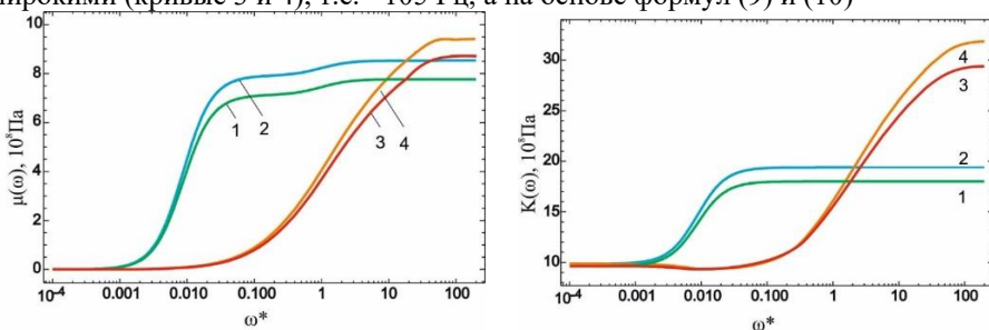
Рис. 6. Зависимость сдвигового \mu(\omega) и объёмного K(\omega) модулей упругости метанола от частоты при температурах t=30^\circ\text{C} (линии 2,4), t=50^\circ\text{C} (линии 1,3) и соответствующих им плотностях при фиксированных \theta_1=30^\circ , \theta_2=45^\circ , \xi_1-\xi_2=0^\circ . Линии 1,2 по формулам (3) и (4), линии 3,4 по формулам (9) и (10).
