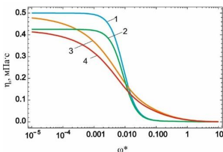
Расм 3. Вобастагии басомадии коэффицентҳои часпакии лағжишӣ \eta_s(\omega) барои метанол дар температураҳои t = 10 °C (хатҳои 1,3), t = 40 °C (хатҳои 2,4) ва зичиҳои мутобиқи онҳо ҳангоми доимӣ будани \theta_1 = 30^\circ , \theta_2 = 45^\circ , \xi_1 - \xi_2 = 0^\circ ; хатҳои 1 ва 2 бо формулаи (6) ва хатҳои 3 ва 4 бо формулаи (1) ҳисоб шудаанд.
