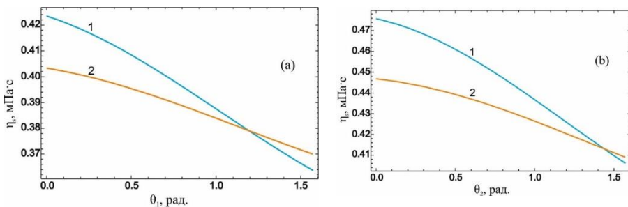
Расм 5. Вобастагии коэффиенти часпакии лағжишии \eta_s(\omega) барои метанол аз кунҷҳои \theta_1 ва \theta_2 дар мавриди доимӣ будани \xi_1 - \xi_2 = 0^\circ ва температураи t = 20^\circ\text{C} ; хатти 1 бо формулаи (6) ва хатти 2 бо формулаи (1) ҳисоб шудааст.
