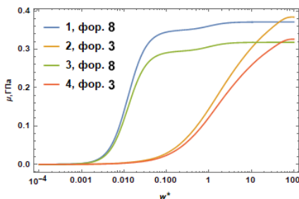
Расм 2. Вобастагии басомадии изотермии \mu(\omega) барои метани моеъ: хатҳои 1 ва 2 дар температураи T=100 К; хатҳои 3 ва 4 дар температураи T=150 К.
