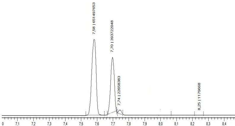
Расми 2 (6). ХБЭ - пайвастаи 11.
