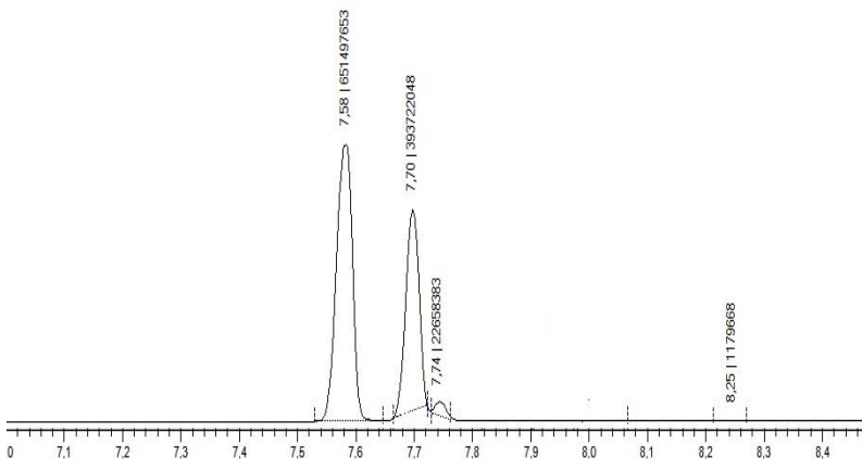
Рисунок 2 (б). ГЖХ - вещества 11.
