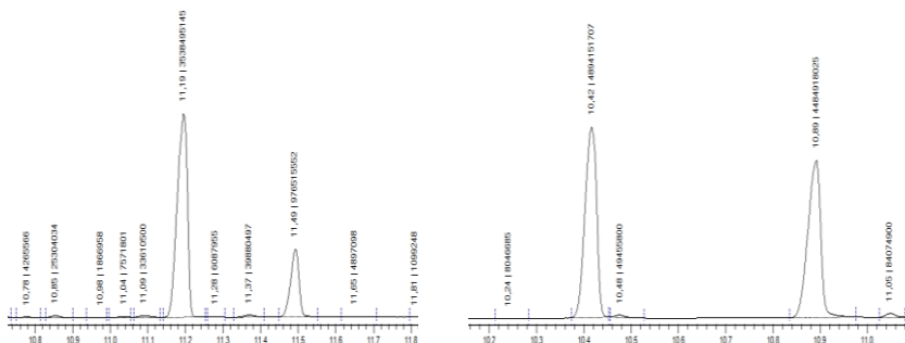
Рисунок 1 (4). ХБЭ – изомеров 5-а,б и 6-а,б
