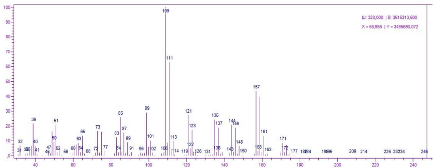
Расми 5 (8). Спектри массавии ДХСП
