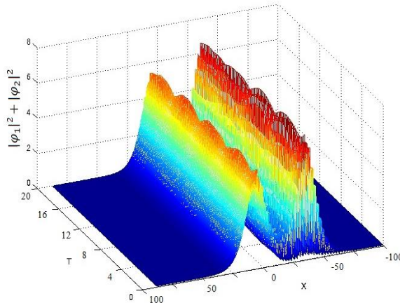
Расми 50. – Графикҳои эволютсияи зичии шумораи зарраҳо ҳангоми суръати ҳаракат v=0.24 .
