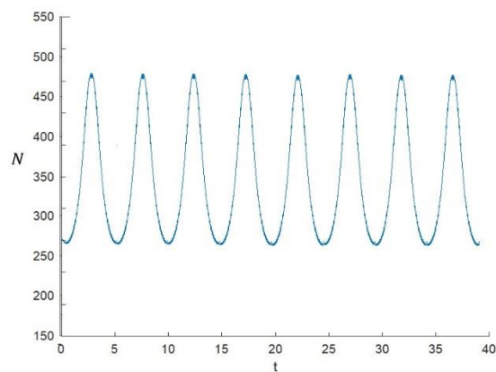
Расми 61. – Интеграли шумораи зарраҳои солитон
