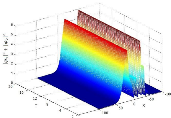
Расми 48. – Графикҳои эволютсияи зичии шумораи зарраҳо ( |\varphi_1|^2 + |\varphi_2|^2 )
