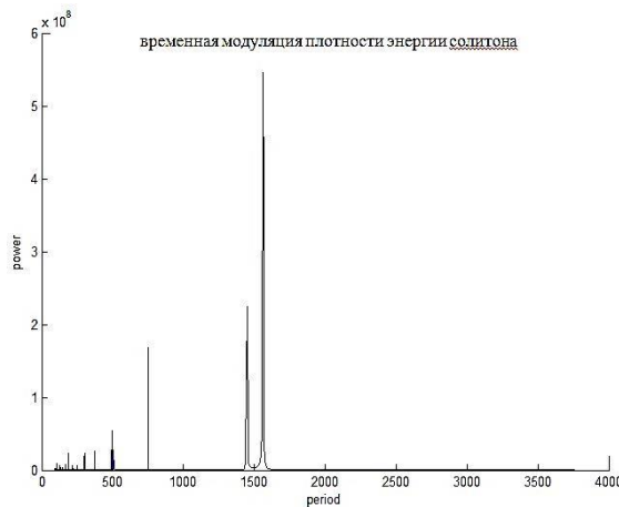
Рисунок 33. - Фурье-анализ временной модуляции плотности энергии двухсолитонного решения
