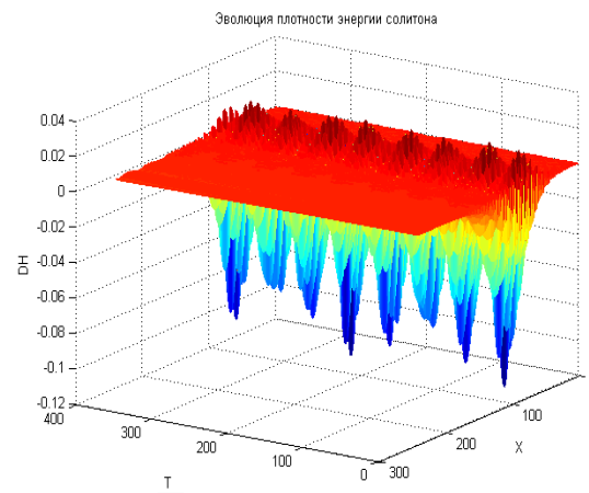
Рисунок 38. - Эволюция плотности энергии солитона с учётом затухания, подкачки и скорости движения v=0.19
