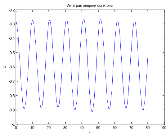
Расми 37. – График, ки вобастагии интегралҳои энергияи солитонро аз вақт бо дарназардошти таъсири хомӯшшавӣ, воридшавии энергия ва суръати ҳаракат v=0.19 инъикос мекунад
