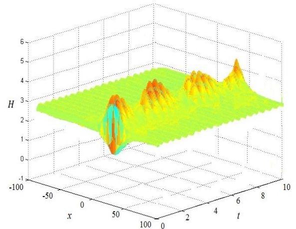
Рисунок 32. - Графики эволюции плотности энергии солитона
