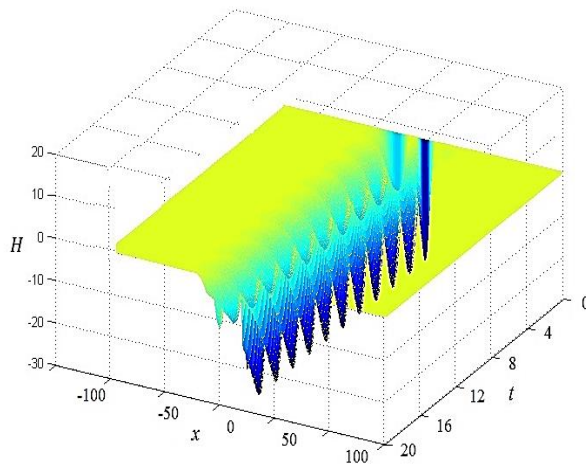
Расми 23. – Эволютсияи зичии энергияи солитон
