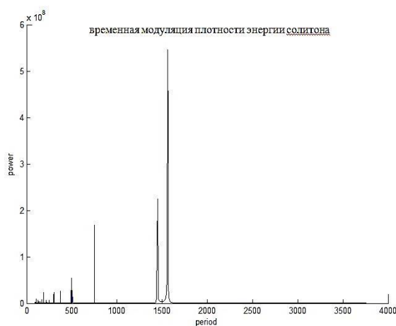
Расми 35. – Таҳлили Фурье-и модулятсияи вақтии зичии энергияи ҳалли дусолитонӣ
