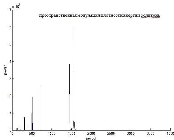
Расми 32. – Таҳлили Фурье-и модулятсияи фазоии зичии энергияи ҳалли дусолитонӣ
