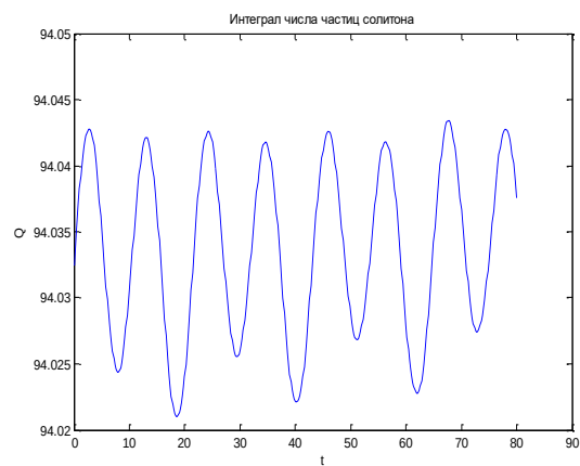
Расми 38. – График вобастагии интегралҳои шумораи зарраҳои солитон аз вақт бо дарназардошти таъсири хомӯшшавӣ, воридшавии энергия ва суръати ҳаракат v = 0.19
