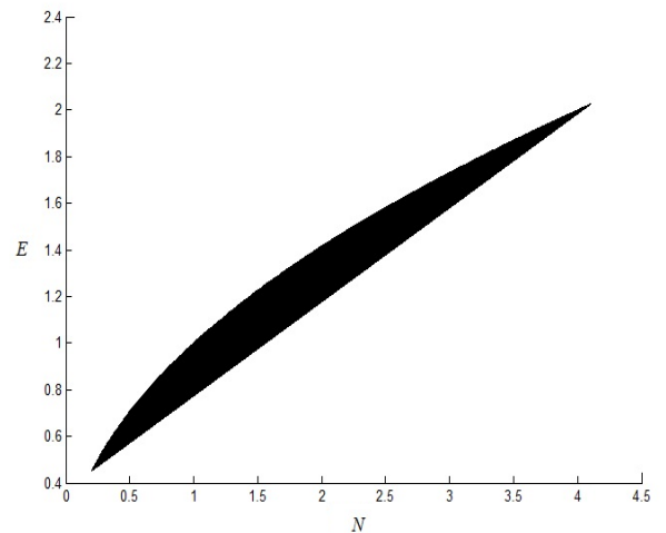
Расми 21. – Масири фазогии система
