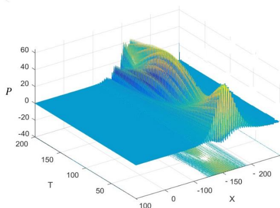
Рисунок 13. - График эволюции плотности импульса солитона при учёте диссипации, подкачки и ненулевой скорости движения
