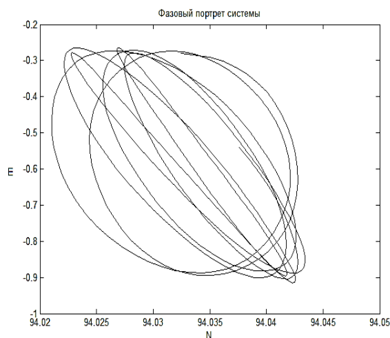
Рисунок 39. - Фазовый портрет солитона, отражающий зависимость интеграла энергии от интеграла числа частиц
