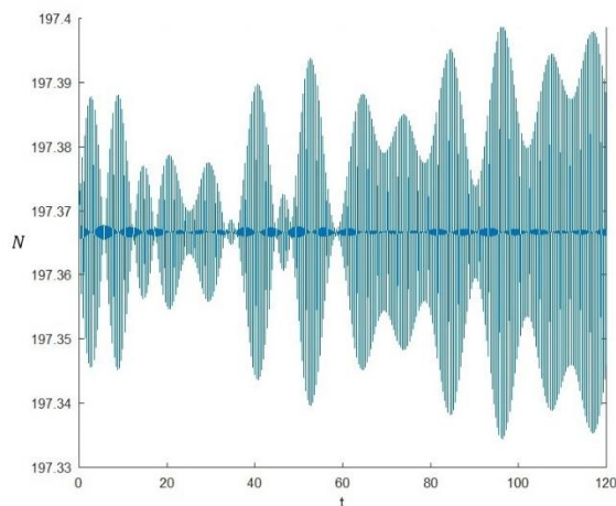
Расми 55. – Интегралҳои шумораи зарраҳои солитон (бо дарназардошти хомӯшшавӣ ва воридшавии берунаи майдонҳо ҳангоми суръати ҳаракат v=0.24 )
