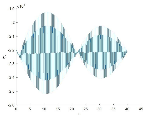
Расми 9. – Графики интегралҳои энергияи солитон бо дарназардошти ҳомӯшшавӣ ва воридшавии энергия
