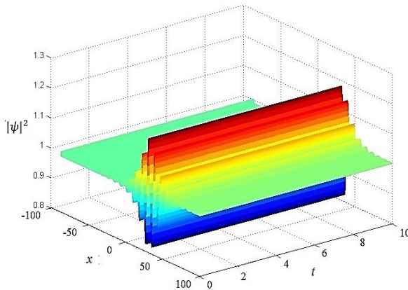
Расми 25. – Графики эволютсияи шумораи зарраҳои солитон
