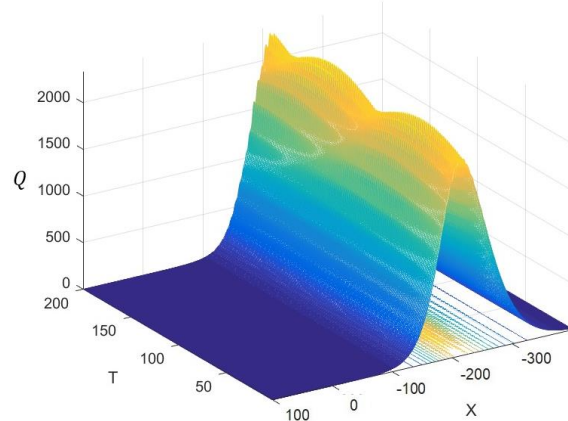
Рисунок 10. - График эволюции плотности числа частиц солитона при учёте диссипации и подкачки
