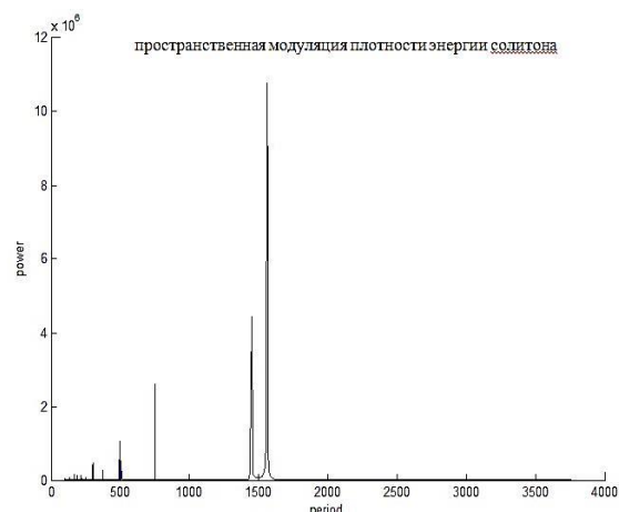
Расми 36. – Таҳлили Фурье-и модулятсияи фазоии зичии энергияи ҳалли дусолитонӣ
