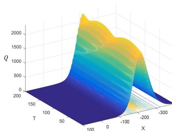
Расми 10. – Графики эволютсияи зичии энергияи солитон бо дарназардошти ҳомӯшшавӣ ва воридшавии энергия
