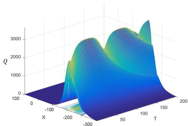
Расми 16. – Графики эволюцияи зичии шумораи зарраҳои солитон бо дарназардошти хомӯшшавӣ, воридшавии энергия ва суръати ҳаракат
