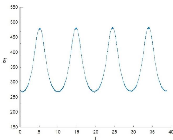
Расми 62. – Интеграли энергияи солитон
