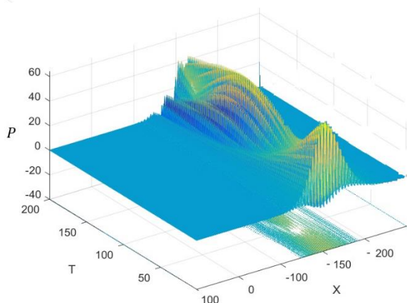
Расми 15. – Графики эволюцияи зичии импулси солитон бо дарназардошти хомӯшшавӣ, воридшавии энергия ва суръати ғайрисиғрии ҳаракат
