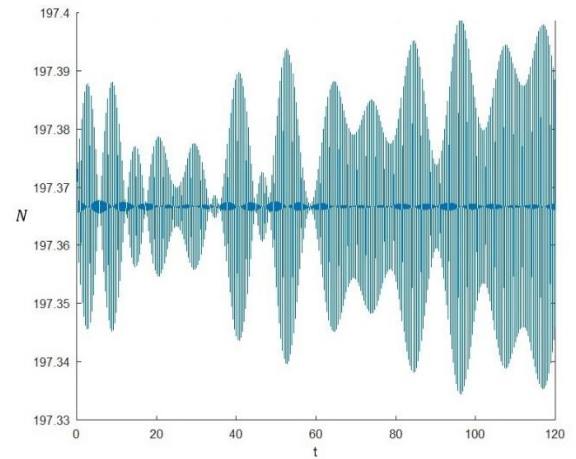
Рисунок 53. - Интеграл числа частиц солитона (при учёте диссипации и подкачки внешними полями со скоростью движения v=0.24 )
