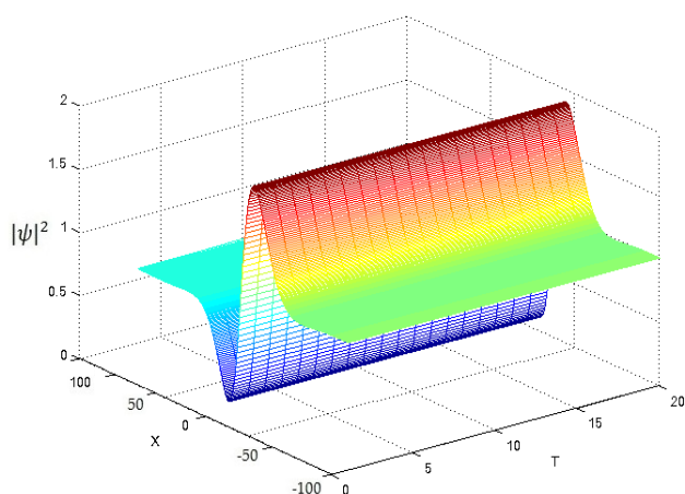
Расми 17. – Динамикаи эволютсияи шумораи зарраҳои солитон бо параметрҳои b = 1 , k_1 = 0.03 , \alpha_1 = 0.19 , \alpha_2 = 0.12 , \beta_1 = 0.096 , \beta_2 = 0.01 , \lambda = 1 , \gamma_1 = 1.265 , \gamma_2 = 0.85
