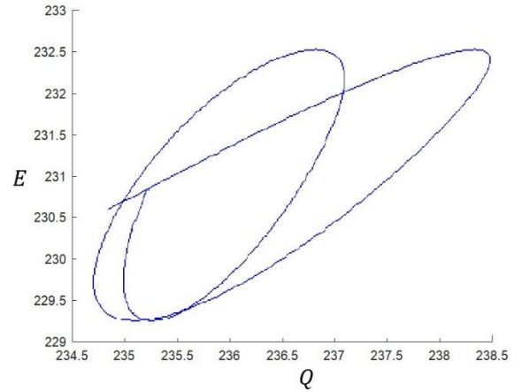
Рисунок 57. - Фазовый портрет системы, показывающий зависимость интеграла числа частиц от интеграла энергии солитона при скорости движения v=0.11
