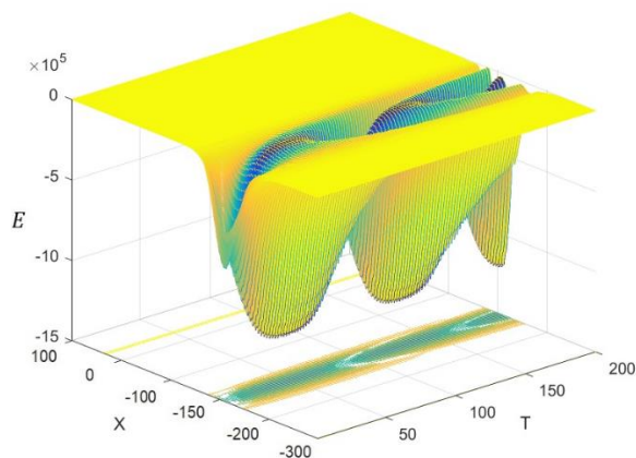
Расми 14. – Графики эволюцияи зичии энергияи солитон бо дарназардошти хомӯшшавӣ, воридшавии энергия ва суръати ҳаракат ( v=0.11 )
