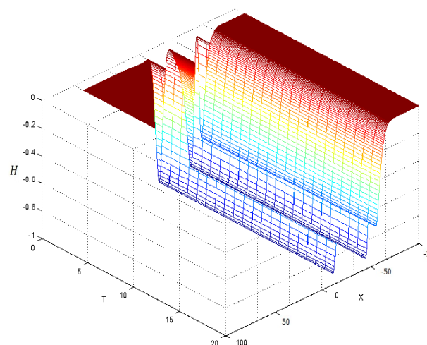
Расми 20. – Динамикаи зичии энергияи солитон дар параметрҳои b = 1 , k_1 = 0.05 , \alpha_1 = 0.019 , \alpha_2 = 0.11 , \beta_1 = 0.096 , \beta_2 = 0.11 , \lambda = 0.5 , \gamma_1 = 0.85 , \gamma_2 = 0.485
