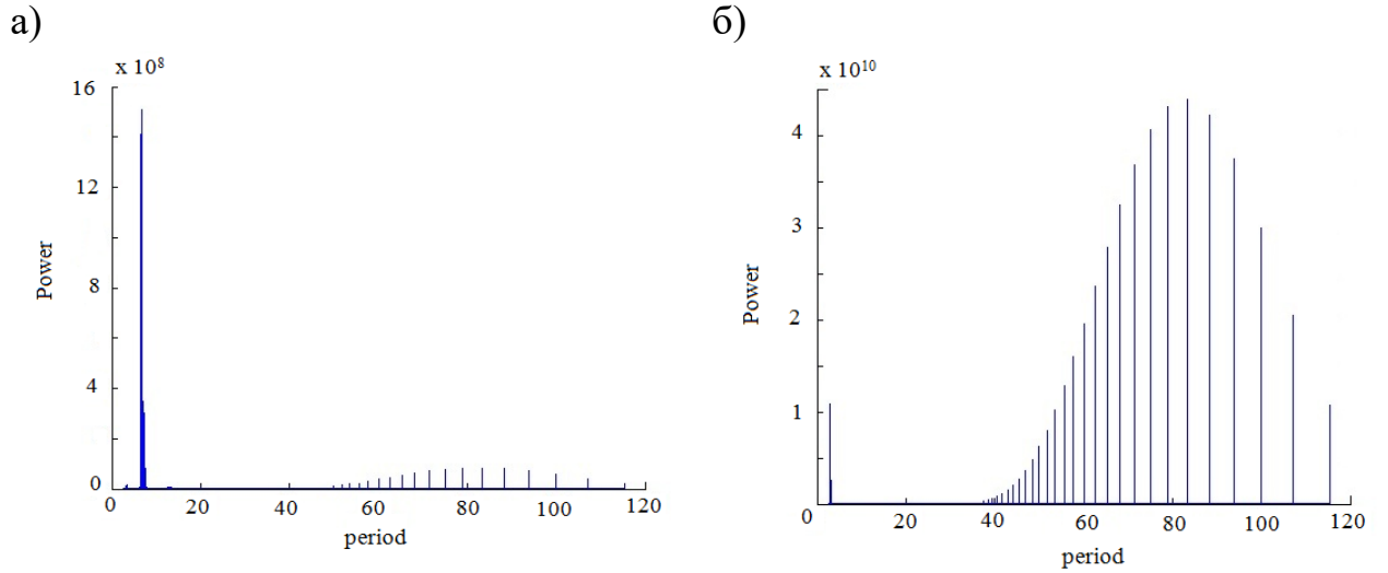
Рисунок 45. - Фурье-анализ временной модуляции плотности энергии (а – для покоящегося солитона, б – при скорости движения v = 0.2 )
