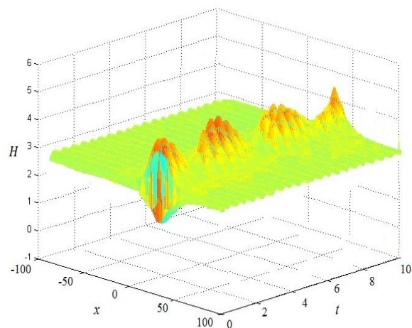
Расми 34. – Графики эволютсияи зичии энергияи солитон
