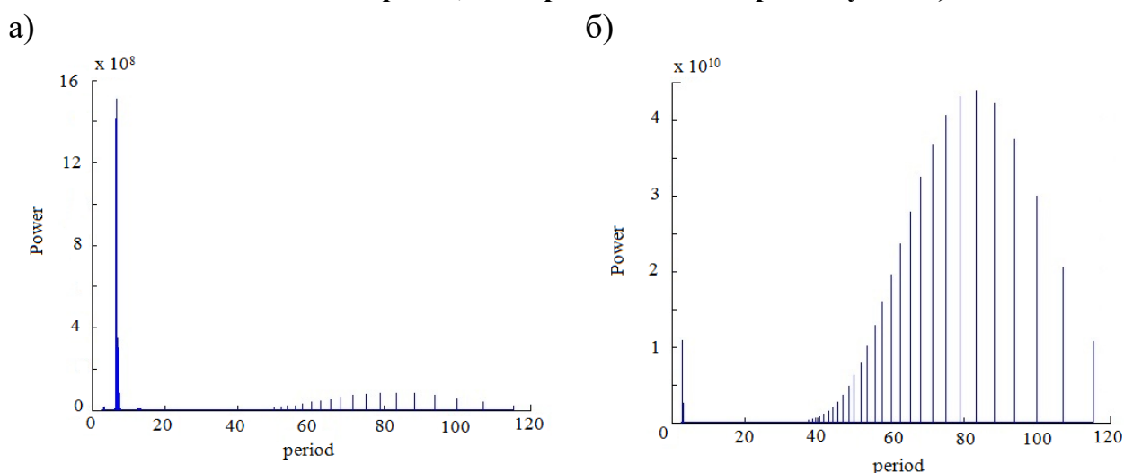
Расми 47. – Таҳлили Фурье-и модулятсияи вақтии зичии энергия (а – барои солитони беҳаракат, б – ҳангоми суръати ҳаракат v=0.2 )
