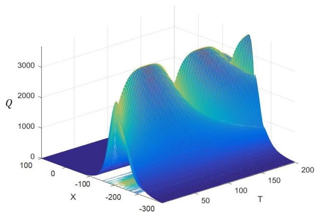
Рисунок 14. - График эволюции плотности числа частиц солитона при учёте диссипации, подкачки и скорости движения
