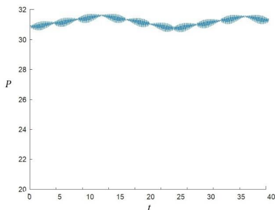
Расми 60. – Интеграли импулси солитон
