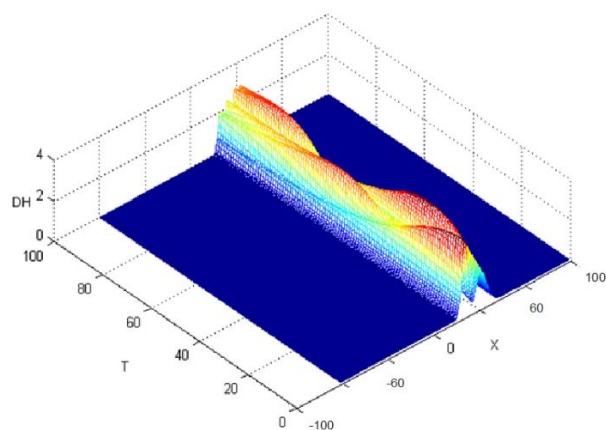
Рисунок 6. - График эволюции плотности энергии солитона ( v=0.12 )
