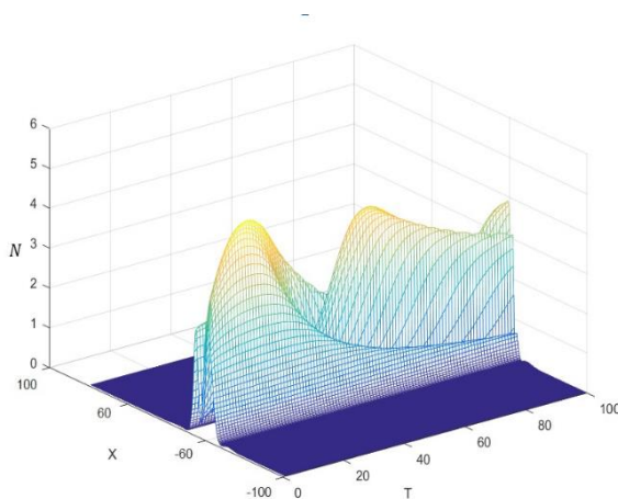
Рисунок 5. - График эволюции плотности числа частиц солитона ( v=0.12 )
