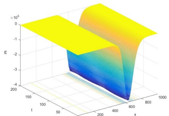
Расми 4. - Графики эволюции зичии энергияи солитон
