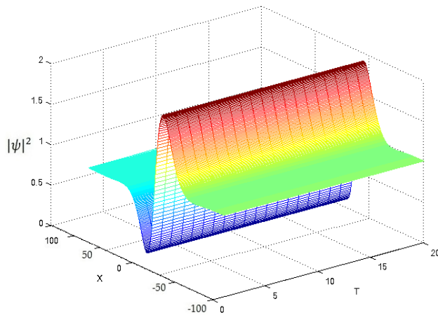
Рисунок 15. - Динамика эволюции числа частиц солитона при параметрах b = 1 , k_1 = 0.03 , \alpha_1 = 0.19 , \alpha_2 = 0.12 , \beta_1 = 0.096 , \beta_2 = 0.01 , \lambda = 1 , \gamma_1 = 1.265 , \gamma_2 = 0.85
