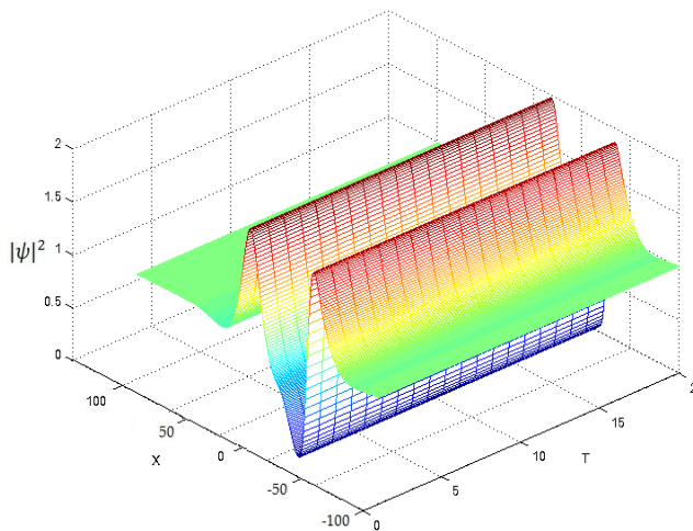
Рисунок 17. - Динамика эволюции числа частиц солитона при параметрах b = 1 , k_1 = 0.05 , \alpha_1 = 0.019 , \alpha_2 = 0.11 , \beta_1 = 0.096 , \beta_2 = 0.11 , \lambda = 0.5 , \gamma_1 = 0.85 , \gamma_2 = 0.485
