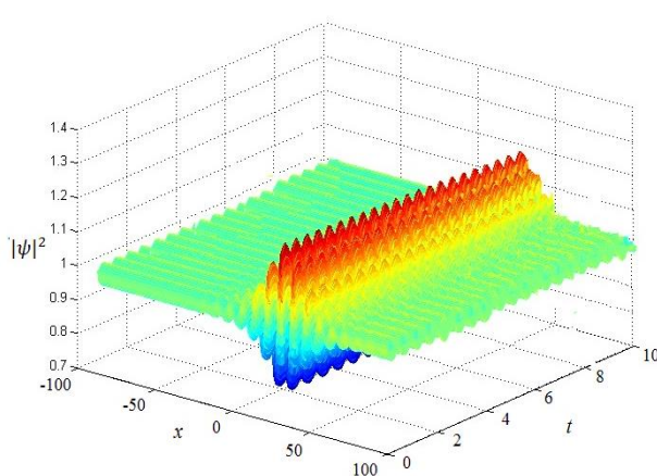
Расми 29. – Эволютсияи шумораи зарраҳои солитон
