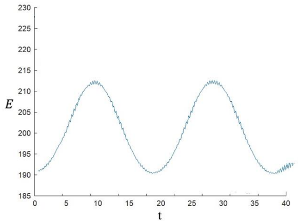
Расми 58. – Интегралы энергияи солитон ҳангоми суръати ғайрисиқри ҳаракат
