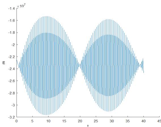
Расми 13. – Графики интегралы энергияи солитон бо дарназардошти хомӯшшавӣ, воридшавии энергия ва суръати ҳаракат ( v=0.11 )
