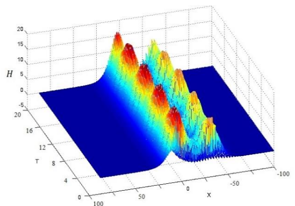
Рисунок 49. - Графики эволюции плотности энергии движущегося солитона
