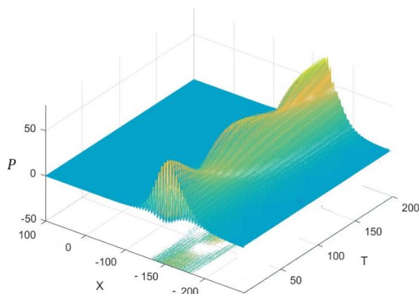
Рисунок 9. - График эволюции плотности импульса солитона при учёте диссипации и подкачки
