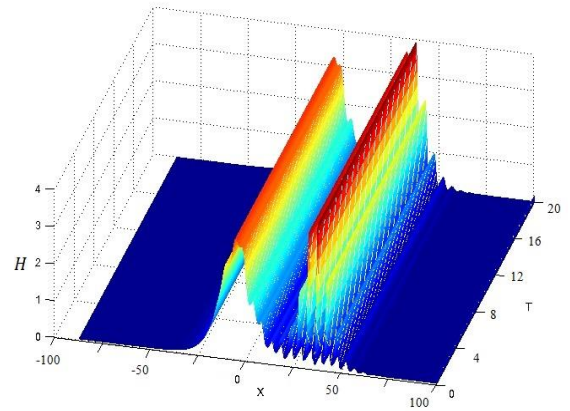
Рисунок 47. - Графики эволюции плотности энергии солитона
