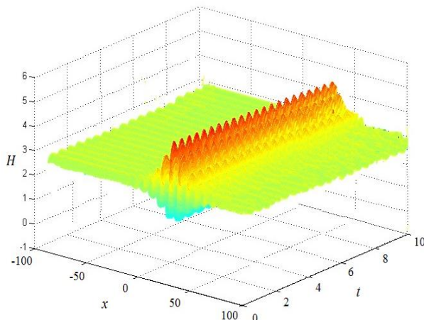
Расми 30. – Графики эволютсияи зичии энергияи солитон
