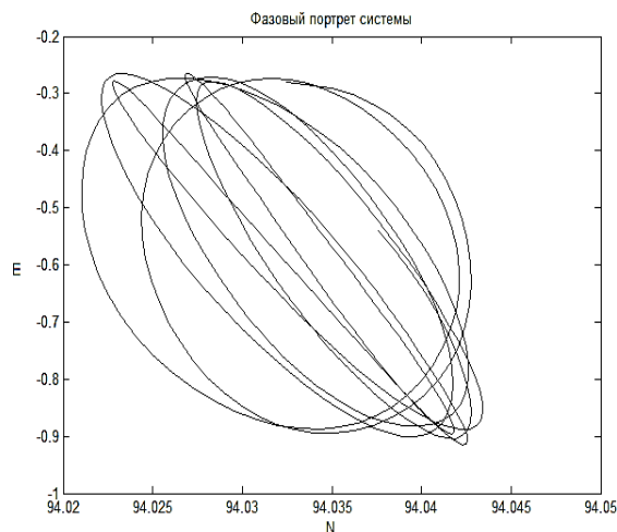
Расми 41. – Масири фазогии солитон, ки вобастагии интегралҳои энергияро аз интегралҳои шумораи зарраҳо инъикос мекунад
