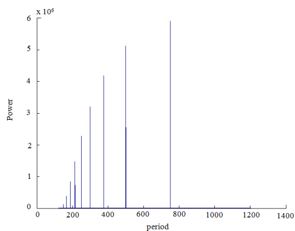
Рисунок 44. - Фурье-анализ пространственной модуляции плотности энергии солитона (а – неподвижного солитона, б – движущегося солитона)
