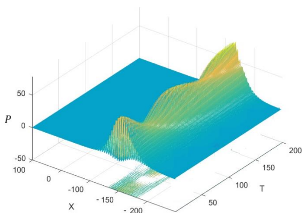
Расми 9. – Графики интегралҳои энергияи солитон бо дарназардошти ҳомӯшшавӣ ва воридшавии энергия
