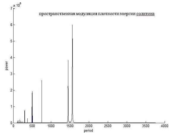
Рисунок 30. - Фурье-анализ пространственной модуляции плотности энергии двухсолитонного решения
