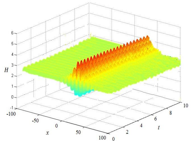
Рисунок 28. - Графики эволюции плотности энергии солитона
