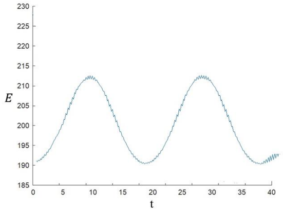
Рисунок 56. - Интеграл энергии солитона при ненулевой скорости движения
