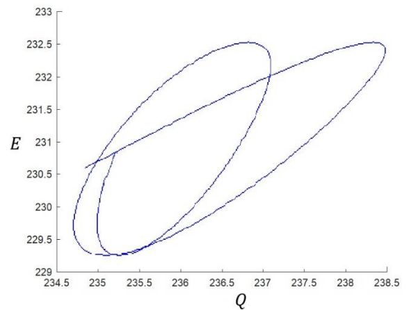
Расми 59. – Масири фазогии система, ки вобастагии интегралы шумораи зарраҳоро аз интегралы энергияи солитон ҳангоми суръати ҳаракат v=0.11 нишон медиҳад
