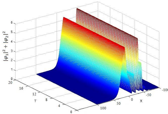
Рисунок 46. - Графики эволюции плотности числа частиц ( |\varphi_1|^2 + |\varphi_2|^2 )
