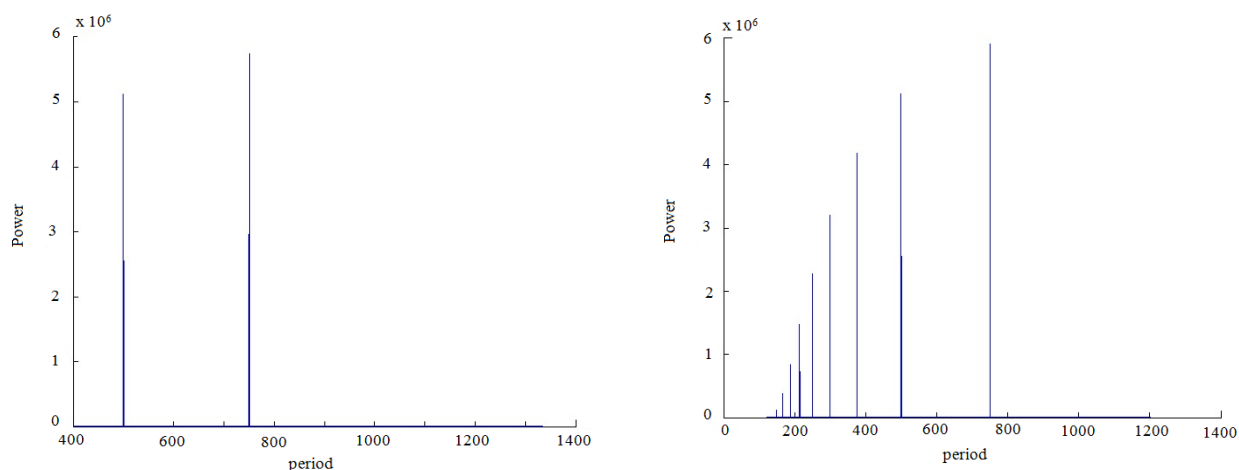
Расми 46. – Таҳлили Фурье-и модулятсияи фазии зичии энергияи солитон (а – барои солитони беҳаракат, б – барои солитони ҳаракаткунанда)
