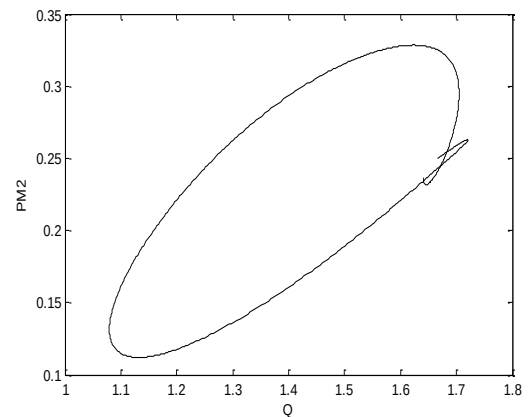
Рисунок 2. - Фазовый портрет солитона
