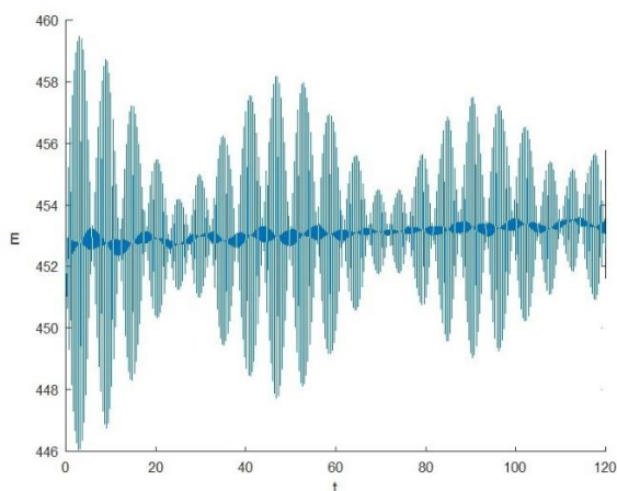
Расми 54. – Интегралҳои энергияи солитон (бо дарназардошти хомӯшшавӣ ва воридшавии берунаи майдонҳо ҳангоми суръати ҳаракат v=0.24 )
