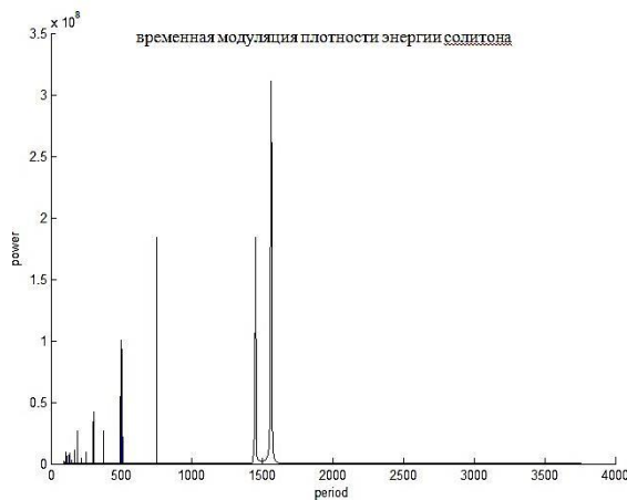
Рисунок 29. - Фурье-анализ временной модуляции плотности энергии двухсолитонного решения
