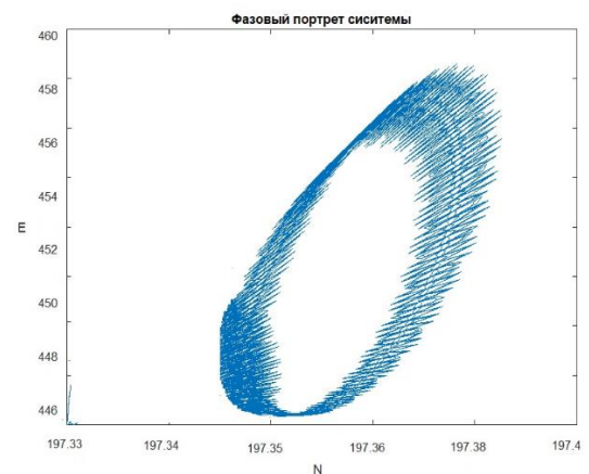
Расми 53. – Масири фазогии система, ки вобастагии интегралҳои энергияро аз интегралҳои шумораи зарраҳо бо дарназардошти хомӯшшавӣ ва воридшавии берунаи майдонҳо дар шароити суръати v=0.24 тасвир мекунад
