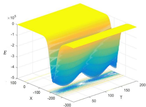
Расми 10. – Графики эволютсияи зичии энергияи солитон бо дарназардошти ҳомӯшшавӣ ва воридшавии энергия
