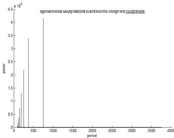
Рисунок 25. - Фурье-анализ временной модуляции плотности энергии двухсолитонного решения
