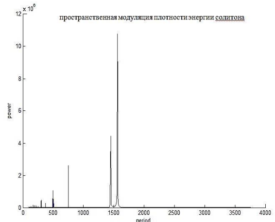
Рисунок 34. - Фурье-анализ пространственной модуляции плотности энергии двухсолитонного решения
