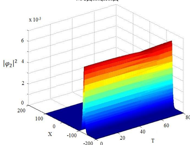
Расми 43. – Графикҳое, ки эволютсияи зичии шумораи зарраҳо барои компонентаи дуюмро ( |\varphi_2|^2 ) нишон медиҳанд
