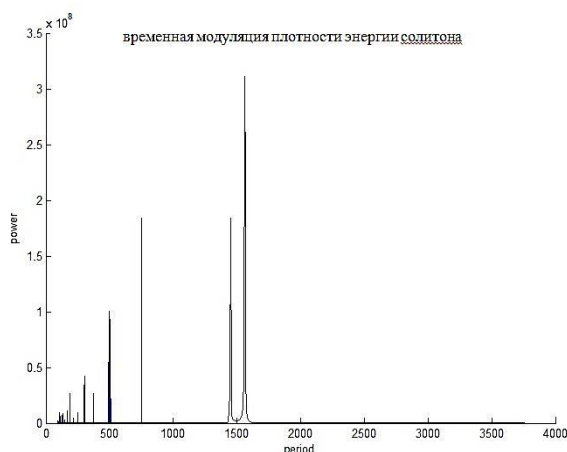
Расми 31. – Таҳлили Фурье-и модулятсияи вақтии зичии энергияи ҳалли дусолитонӣ
