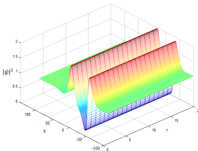
Расми 19. – Динамикаи эволютсияи шумораи зарраҳои солитон дар параметрҳои b = 1 , k_1 = 0.05 , \alpha_1 = 0.019 , \alpha_2 = 0.11 , \beta_1 = 0.096 , \beta_2 = 0.11 , \lambda = 0.5 , \gamma_1 = 0.85 , \gamma_2 = 0.485
