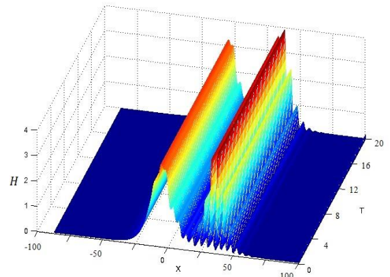
Расми 49. – Графикҳои эволютсияи зичии энергияи солитон
