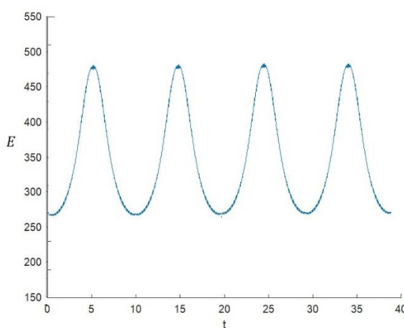
Рисунок 60. - Интеграл энергии солитона
