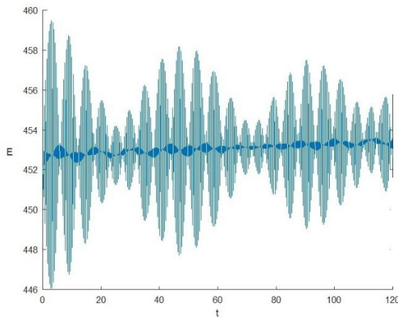
Рисунок 52. - Интеграл энергии солитона (при учёте диссипации и подкачки внешними полями со скоростью движения v=0.24 )
