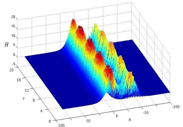
Расми 51. – Графикҳои эволютсияи зичии энергияи солитони ҳаракаткунанда
