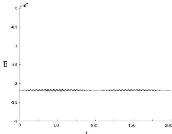
Расми 3. - Графики интегралы энергии солитон
