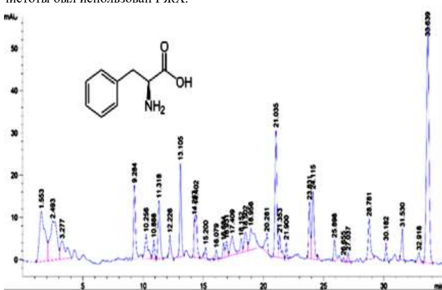
Рисунок 3- Хроматограмма треонина*, Thr, полученного из соединения шалфея мускатного
