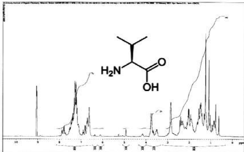
Рисунок 2- ПМР- спектра (S)-2- аминокислота (Валин), полученная из соединения шалфея мускатного
