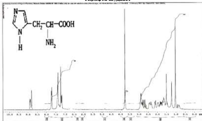
Расми 6. -спектри - РМП - Треонин*, Ҳг ки аз таркиби мармараки мускатӣ гирифта шудааст
