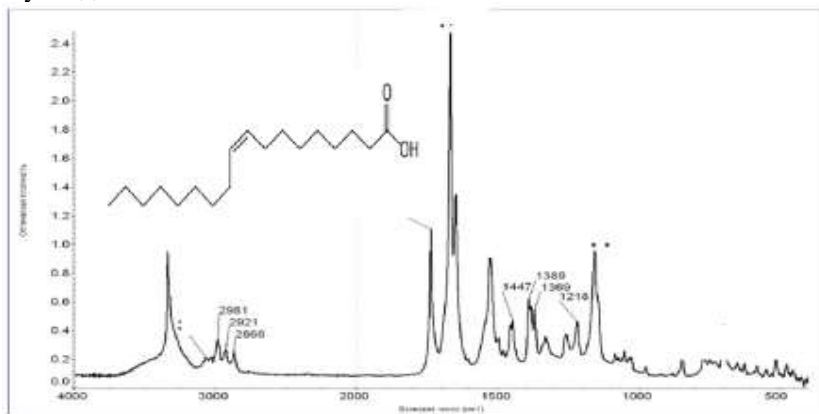
Расми 8.- СИ - кислотаи олеинӣ ки аз таркиби мармараки мускатӣ ғирифта шудааст
