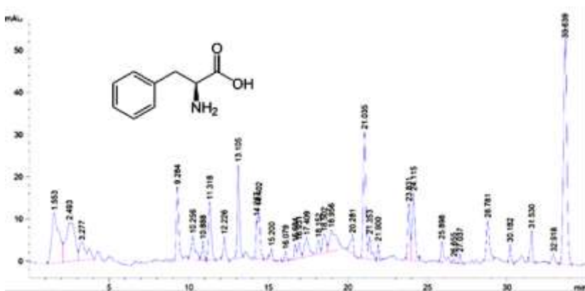
Расми 3.- Хроматограммаи Треонин*, T hr ки аз таркиби мармараки мускатӣ гирифта шудааст
