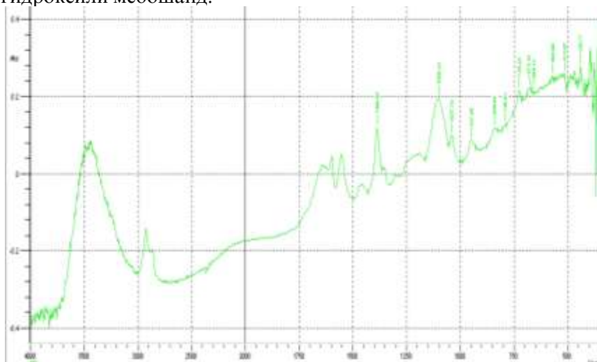
Расми 5.- СИ- Треонин*, Ҳг ки аз таркиби мармараки мускатӣ гирифта шудааст
