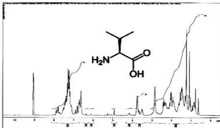
Расми 2. -спектри - РМП-(S)-2-амино-3-кислотаи метилбутанат (Валин) ки аз таркиби мармараки мускатӣ гирифта шудааст
