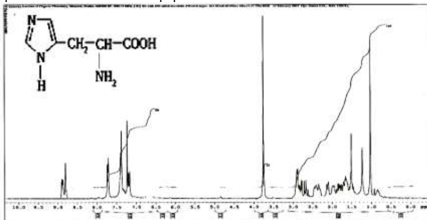
Рисунок 6- ^1\text{H} -ЯМР-спектра Треонин*, Thr, полученный из соединения шалфея мускатного
