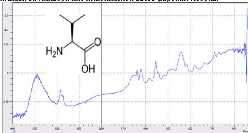
Расми 1.- СИ- (S)-2-амино-3-кислотаи метилбутанат (Валин) ки аз таркиби мармараки мускатӣ гирифта шудааст
