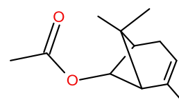
цис-Хризантенил ацетат
