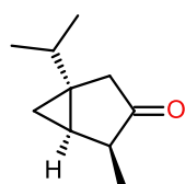
\alpha -Туйон
