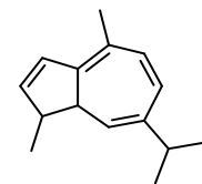
Дигидрохамазулен
