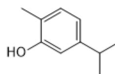
Карвакрол
