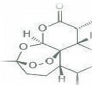
Артемизинин
