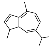
Дигидрохамазулен
