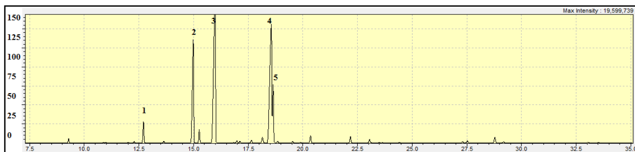
Расми 1. Хроматограммаи рағани атрии баргҳои Ferula clematidifolia 1. \alpha -пинен 2. сабинен 3. мирсен 4. лимонен 5. \beta -фелландрен
