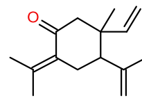
Камфора
