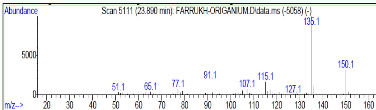
Расми 5. Намунаи фрагментатсияи m/z -и молекулаи тимол, ки ҳангоми таҳлили хроматографияи газӣ-масс-спектрометрии рағани атрии Origanum tyttanthum сабт гардидааст.
