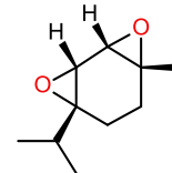
Изоаскаридол
