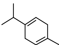
γ-Терпинен
