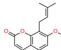
Остол
