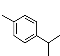
п-Симол
