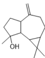
Спатуленол
