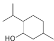
Неоментол
