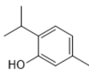
Тимол
