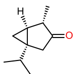
сис-Пинокамфон
