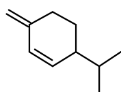
β-Фелландрен
