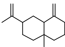
β-Селинен
