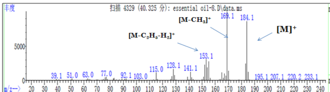
Расми 6. Намунаи масс фрагментатсияи m/z-и молекулаи хамазулен
