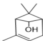
сис-Хризантенол
