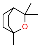
1,8-Синеол
