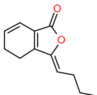
(Z)-Лигустилид
