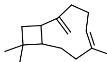
Бициклогермакрен
