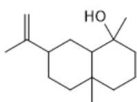
Интермедел
