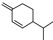
β-Фелландрен
