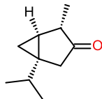
\beta -Туйон
