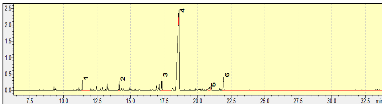
Расми 2. Хроматограммаи РА-и Galagania fragrantissima . 1. деканал 2. (4E)-додеканал 3. додеканал 4. (2E)-додеканал 5. (2E)-додекенал 6. (2E)-тетрадекенал.
