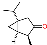
\alpha -Туйон
