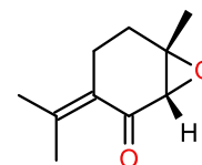
сис -Пиперитенон оксид
