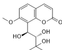
Юғанин А
