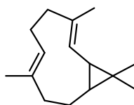
Бисиклогермакрен
