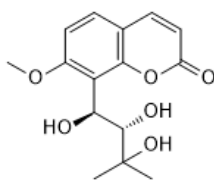
Юганин А
