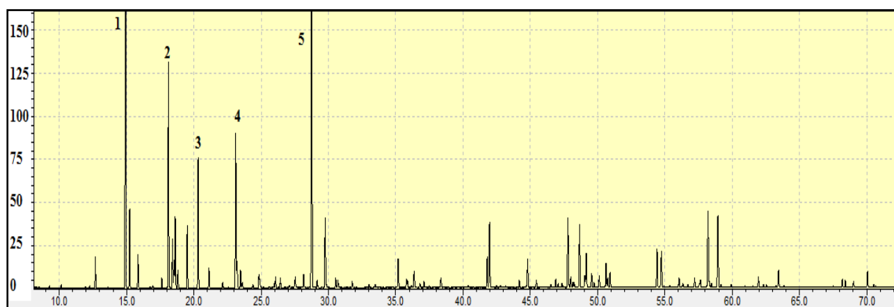
Расми 3. Хроматограммаи РА-и Polychrysium tadshikorum . 1. сабинен 2. п-симол 3. \gamma -терпинен 4. линалоол 5. терпинен-4-ол.
