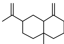
β-Селинен
