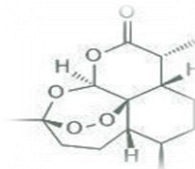
Артемизинин
