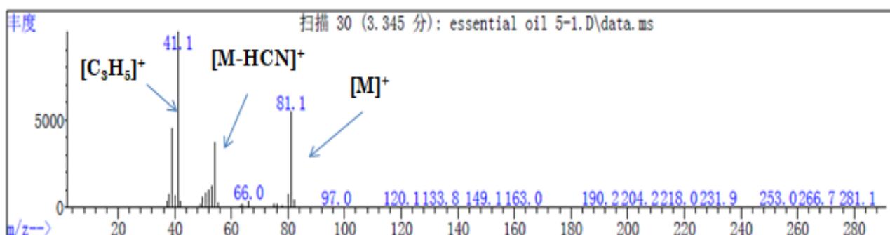
Расми 10. Намунаи масс фрагментатсияи m/z-и молекулаи 3-метил-2-бутеннитрил
