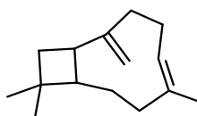
Бисиклогермакрен
