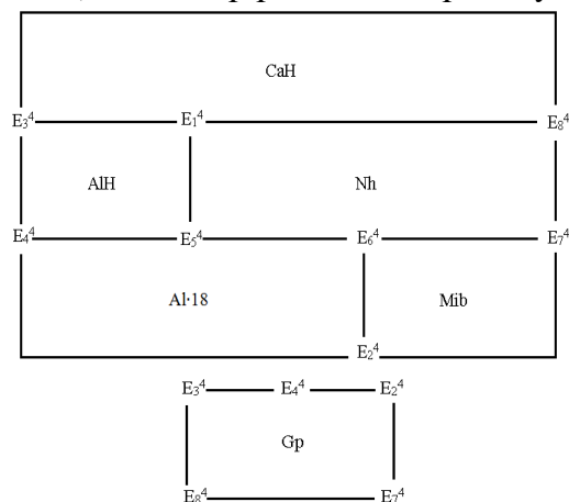
Расми 5 – Диаграммаи схематикӣ сатҳи чоркомпонентагӣ табдилоти фазагӣ дар системаи тартиби дуум (ионҳои натрий, калсий, алюминий, гидрокарбонат, сульфат ва об) дар 273 К.
