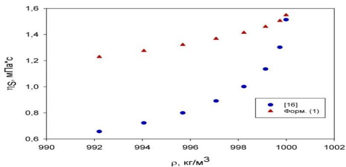
Рис. 3. Плотностная зависимость сдвигового вязкости для воды
