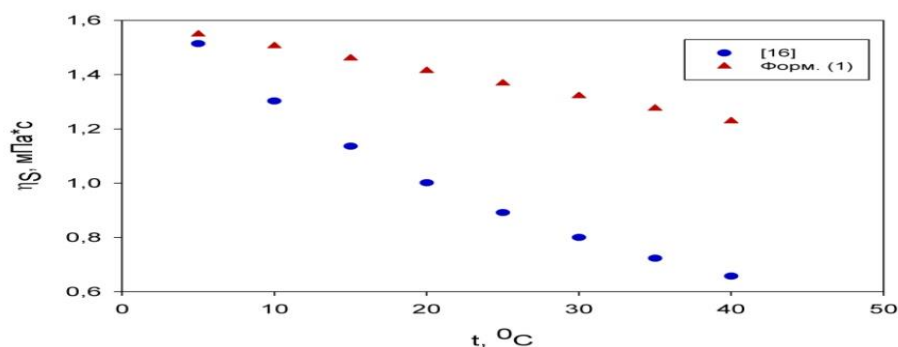
Рис. 2. Температурная зависимость сдвигового вязкости воды
