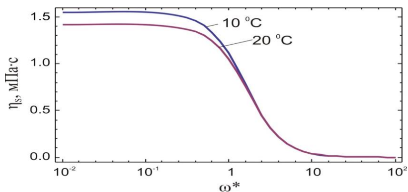
Рис. 1. Частотная зависимость коэффициента сдвиговой вязкости воды при различных температурах.
