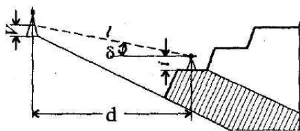
Расми 4. Нивелиркунонии тригонометри дар қарер
