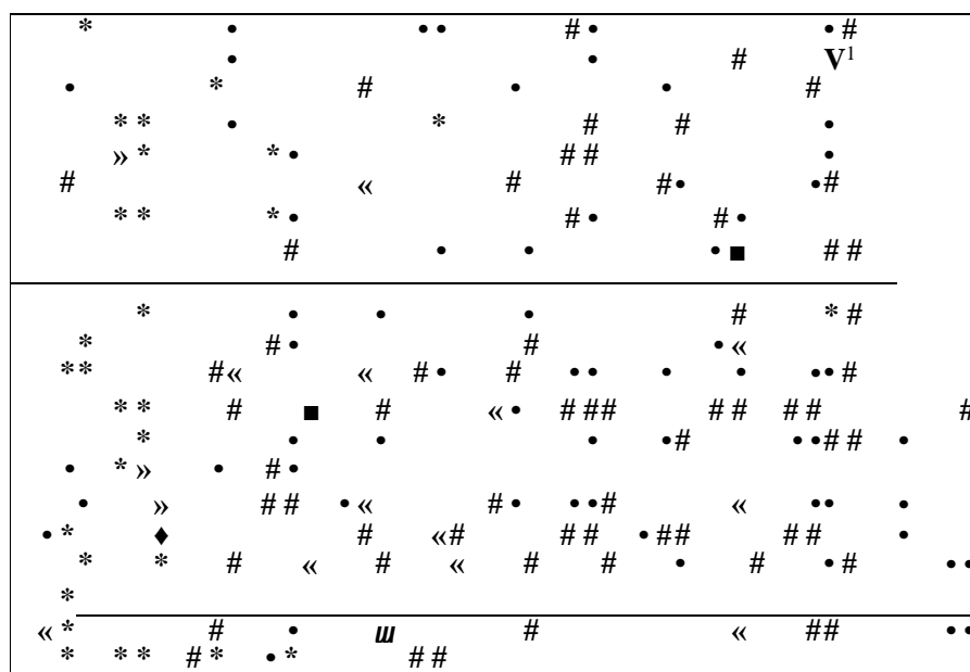
Рис. 4. Полнота первой степени
