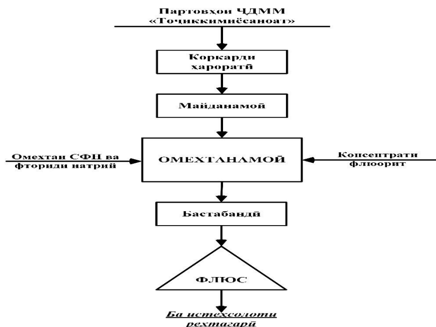
Расми 2 – Схекаи принципиалию технологияи ҳосил намудани флюс дар асоси СФН ва фториди натрий.
