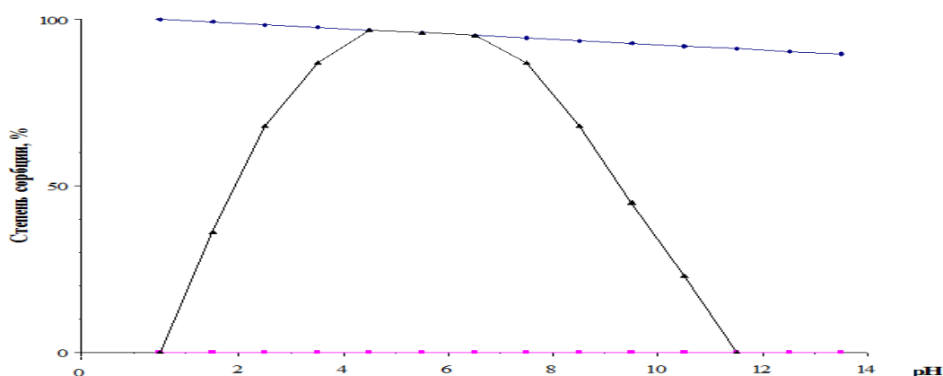
Рис.1. Сорбция 1 \cdot 10^{-6} моль ^{198}\text{Au} ГО железа (III) 1-Сорбция из 1 моль KCl
