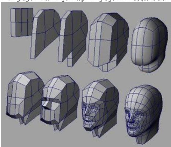
Расми 4 - Моделсозии сари инсон бо усули полигон
