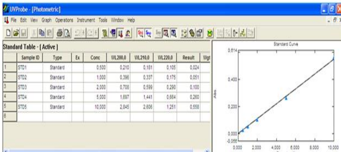
Расми 3. Қиматҳои нурфурубарии маҳлулҳои стандартии калтсий ва графики вобастагии нурфурубарӣ аз консентратсияи он
