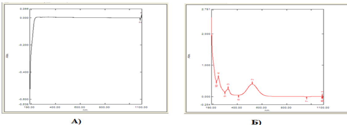
Расми 7. Спектри фурубари маҳлули ионҳои тилло А) дар маҳлули обӣ ва Б) дар иштироки дитизон
