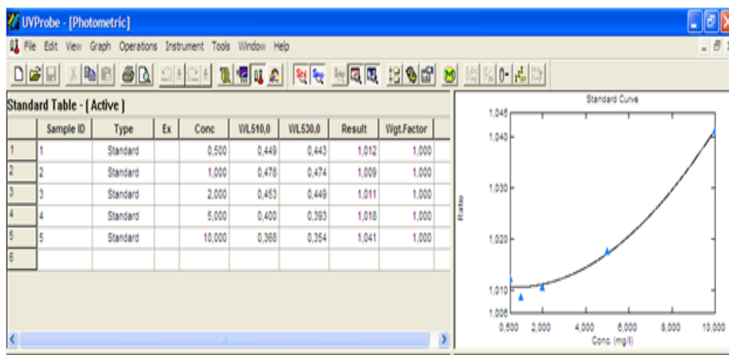
Расми 8. Қиматҳои нурфурубари маҳлулҳои стандартии тилло ва графики вобастагии нурфурубарӣ аз консентратсияи он
