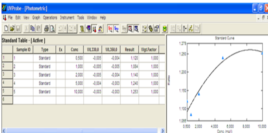
Расми 4. Қиматҳои нурфурубарии маҳлулҳои стандартии магний ва графики вобастагии нурфурубарӣ аз консентратсияи он
