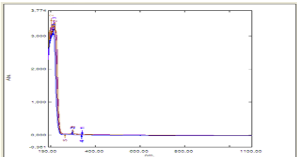
Расми 1. Спектри фурубарии маҳлули калтсий дар иштироки Эриохроми сик Т.
