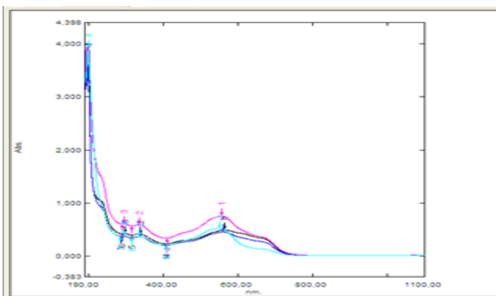
Расми 2. Спектри фурубарии маҳлули магний дар иштироки Эриохроми сиёҳ Т.
